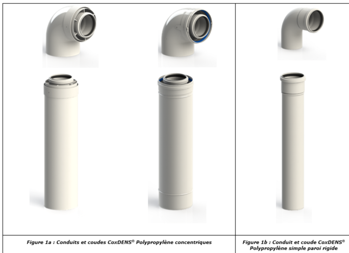
Figure 1 : Conduits CoxDENS® Polypropylène
