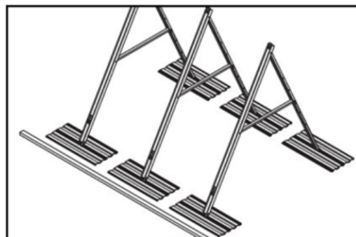
Alignement des bâtis
