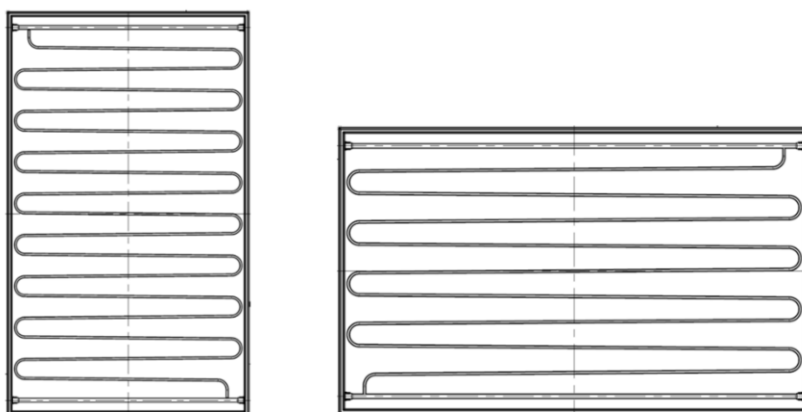
Figure 4 - Grille hydraulique d'absorbeur
