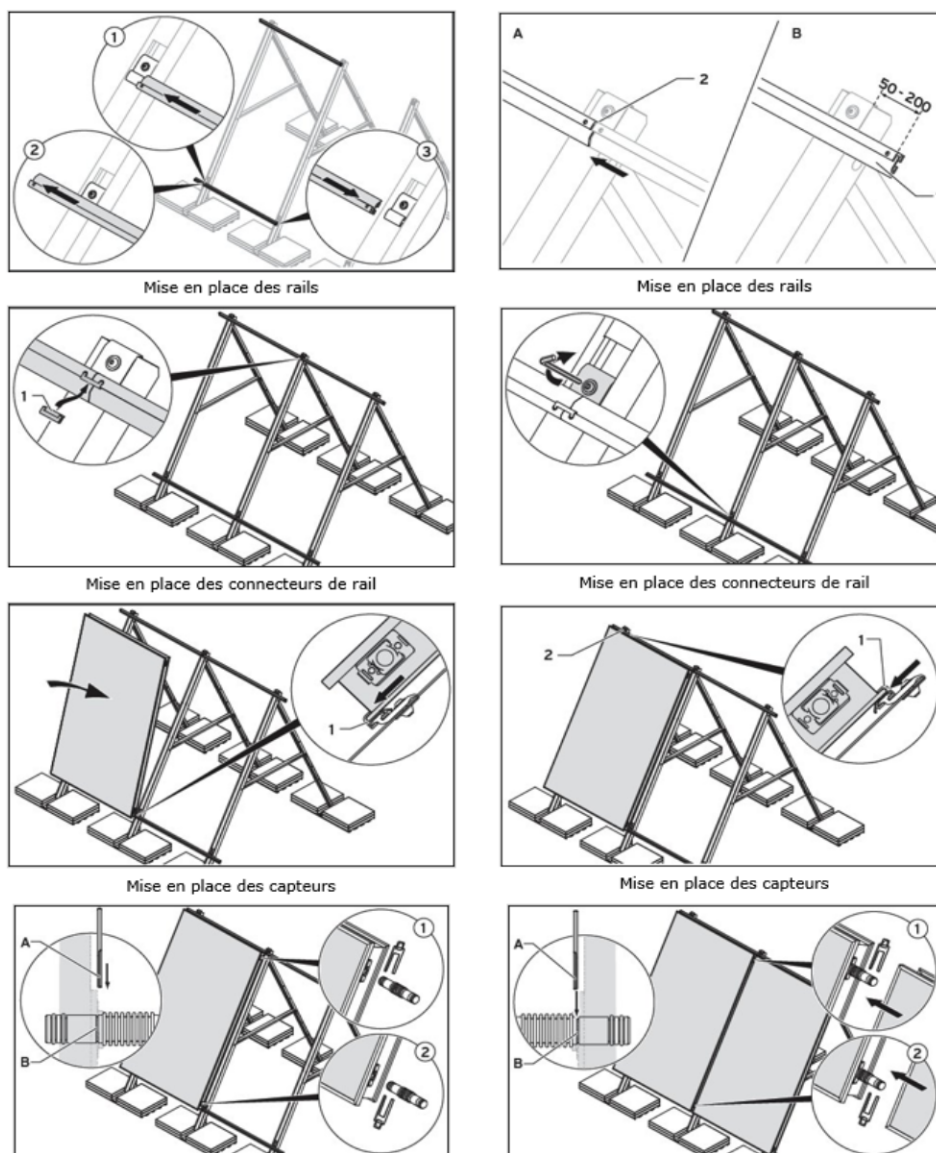
Figure23 – Mise en œuvre des capteurs sur les châssis
