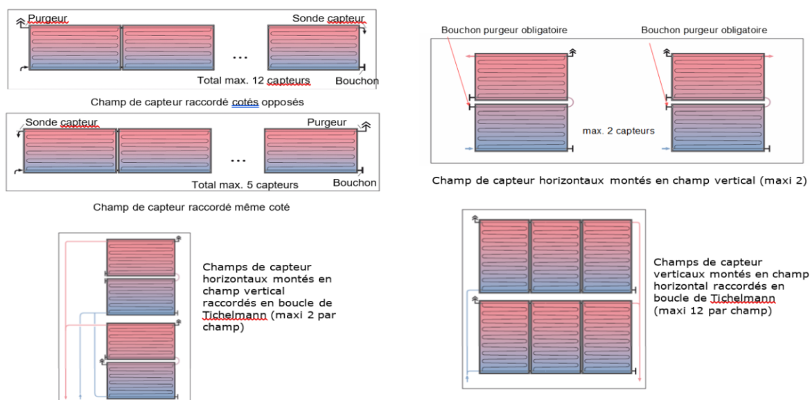
Figure 6 – Raccordement hydraulique des capteurs
