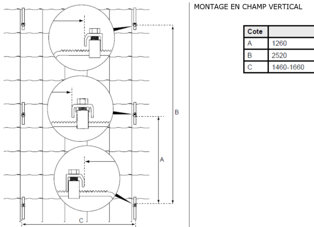
Figure 10 – Agencement des capteurs (suite)
