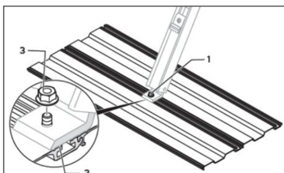
Boulonnage des bâtis sur les plaques
