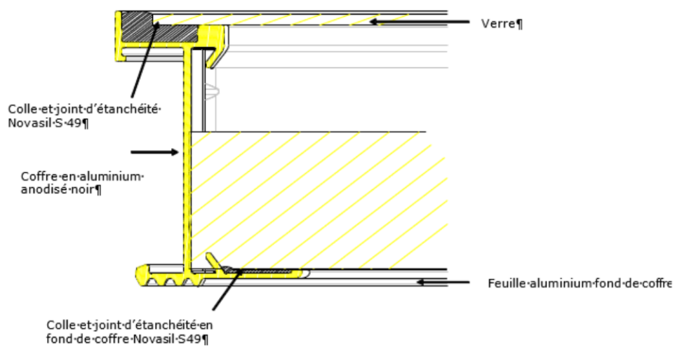
Figure 2 – Vue en coupe du coffre
