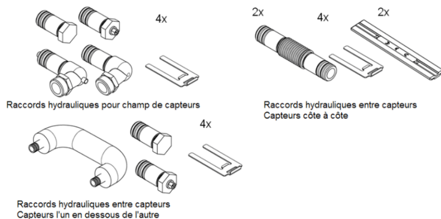
Figure 5 - Raccords hydrauliques et manchons thermo rétractables pour raccordement de la sonde
