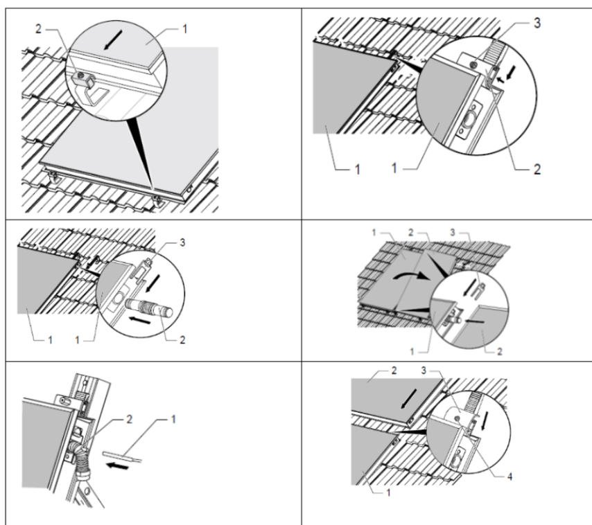
Figure 16 – Montage des capteurs
