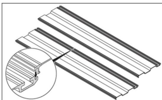
Emboîtement des plaques de lestage
