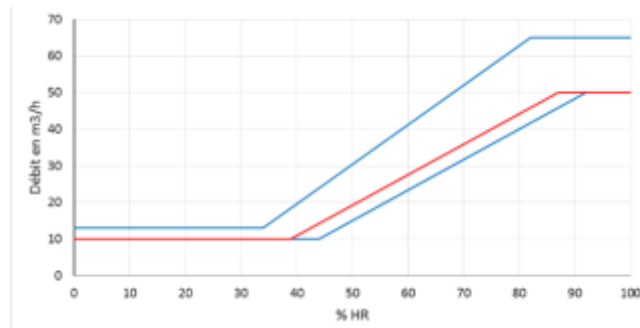
Figure 11 – VTH C1 – Courbe hygroaéroulrique
