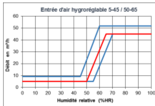
Figure 2 – Entrée d'air hygroréglable 5-45 / 50-65 (HY) Caractéristiques hydroaérodynamiques pour une différence de pression de 20 Pa
