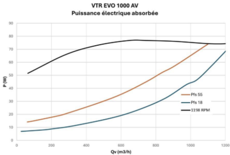
Figure 35 – VTR EVO 1000 AV Courbes débit/pression (en mode « courbe plate » et en mode « vitesse auto régulée ») et courbe débit/puissance
