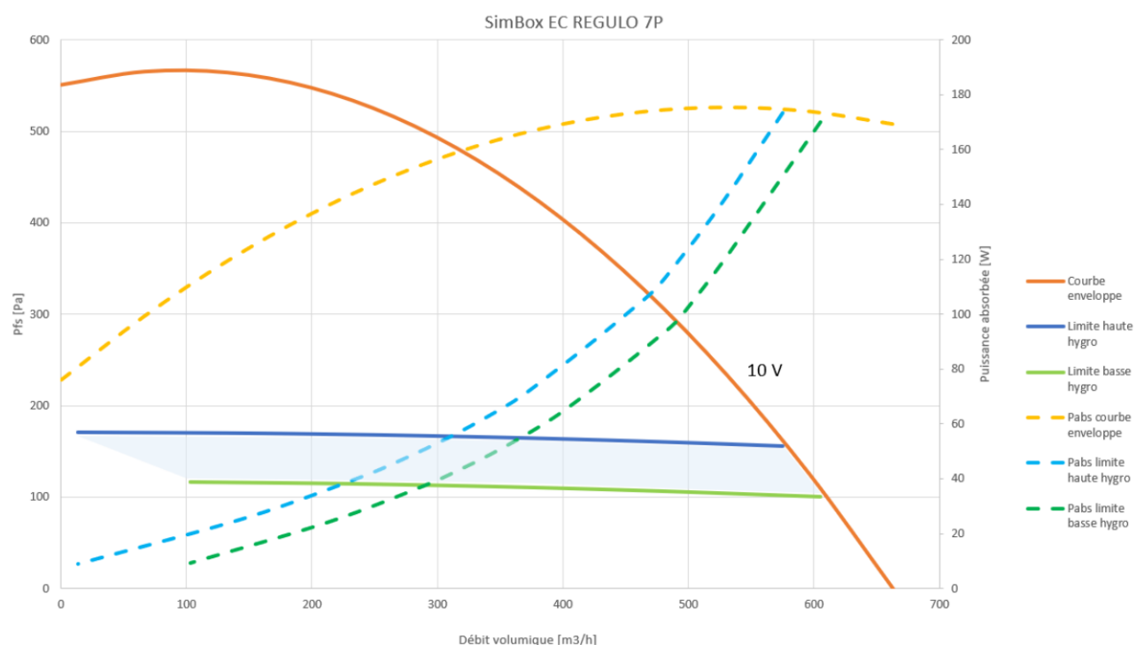
Figure 69 –SimBox EC REGULO 7P
