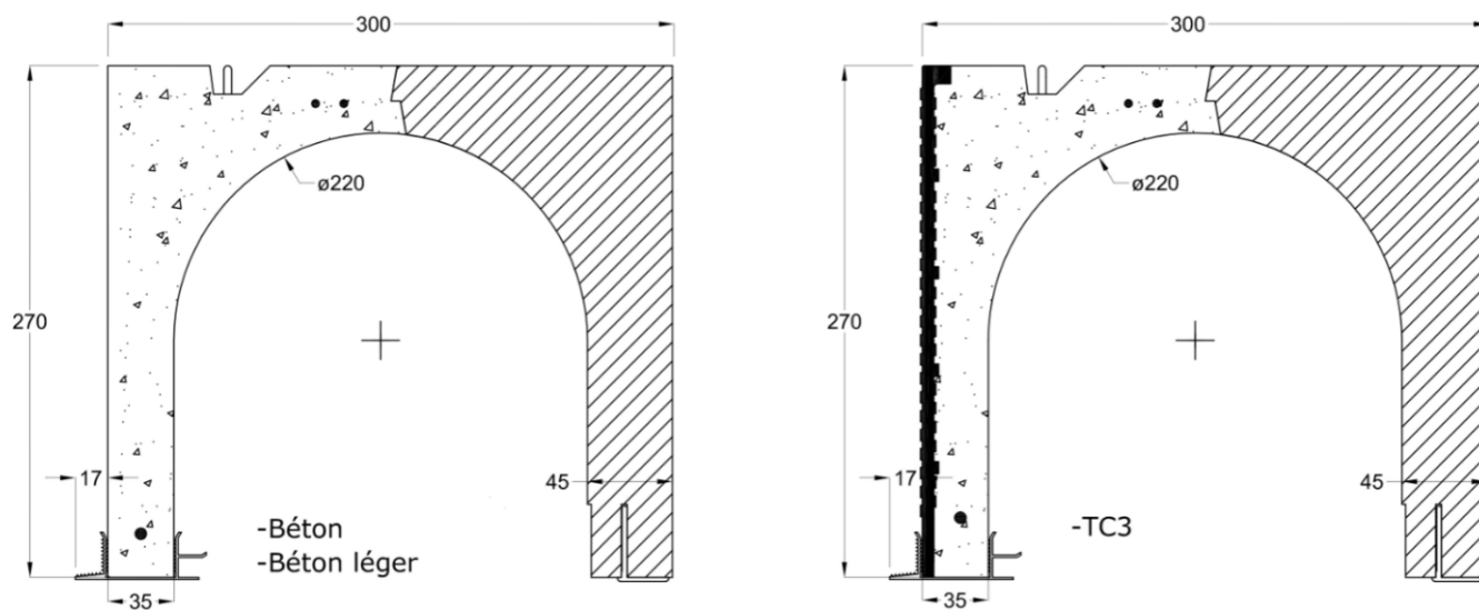
Figure 2 – Coffre PERFECTO Gen3 : finitions extérieures : béton, béton léger et béton standard + terre cuite (TC3)
