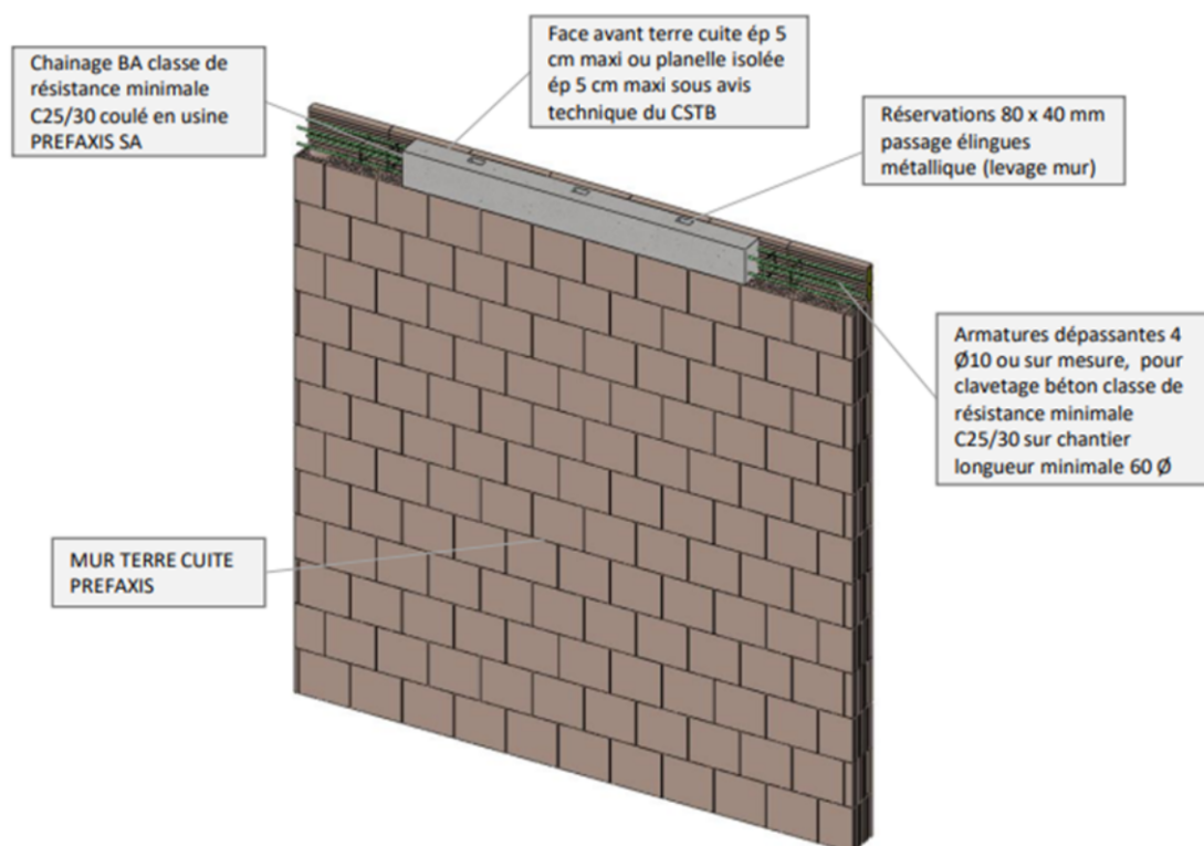
Figure 29 Détail mur avec chainage horizontal
