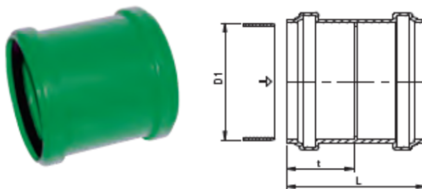
Figure 3.4 : Manchons à butée
