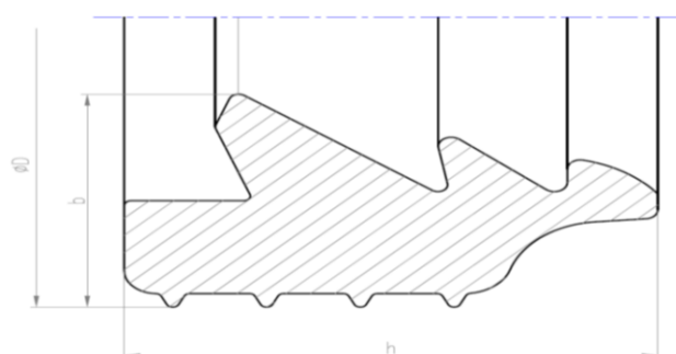
Figure 2 : Garniture d'étanchéité – joint à triple lèvre pour tubes et raccords
