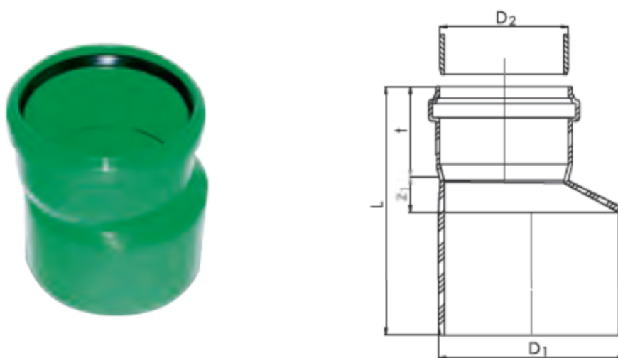
Figure 3.3 : Augmentations excentrées
