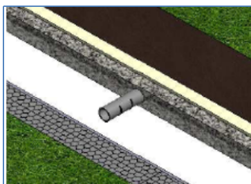
Figure 4a – Système de ventilation avec matériaux drainants (sur Nidaplast ou Nidaflow)
