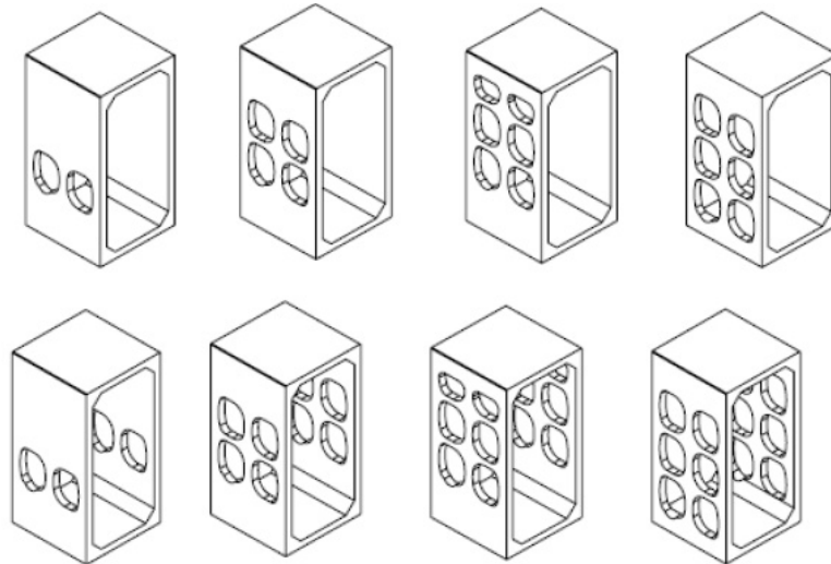
Figure 10 : Gamme de cadres pour la réalisation de la galerie d'accès
