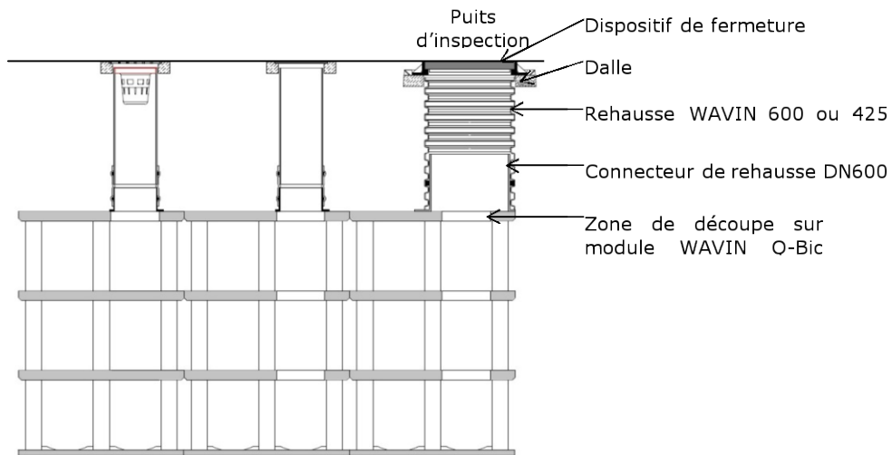
Figure 9b –Détail de puits d'inspection et d'un puits de ventilation pour bassin à plusieurs couches de modules WAVIN Q-Bic Plus
