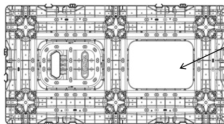
Figure 7 - Détail de découpe d'un puits d'inspection intégré
