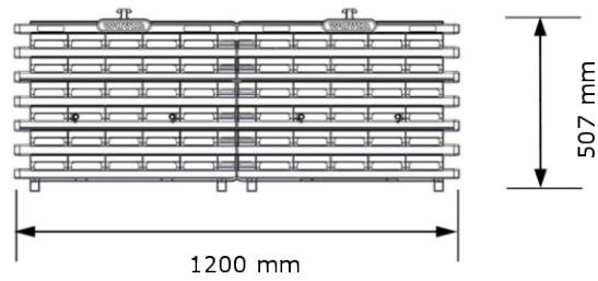
Figure 3b – Caractéristiques dimensionnelles de la plaque latérale
