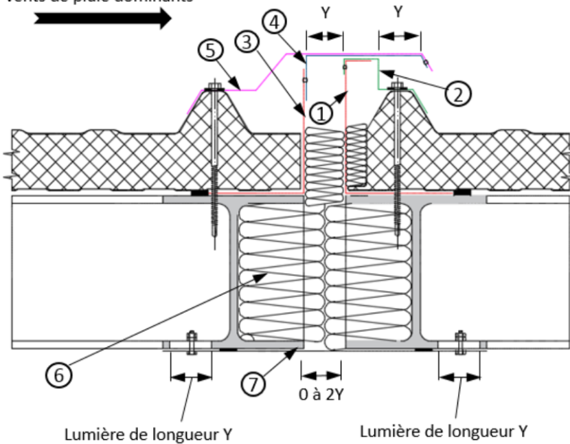
Figure 28 - Exemple 2 de joint de dilatation
