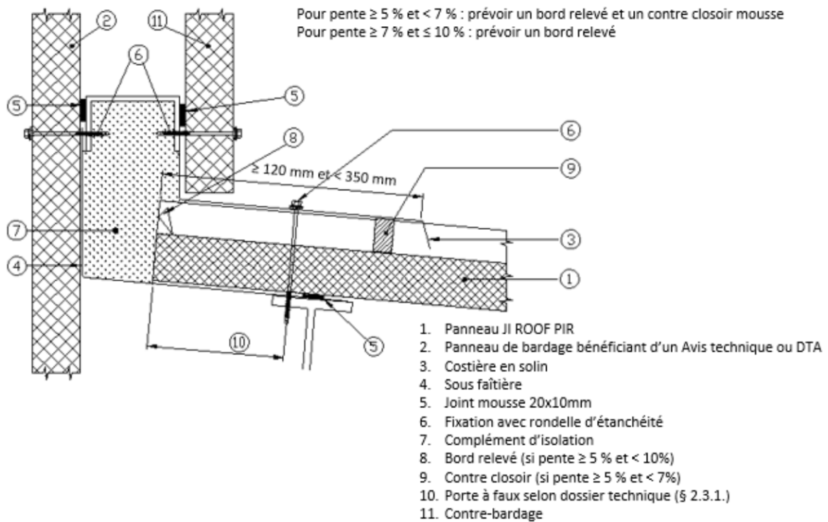
Figure 20 - Faîtage en solin
