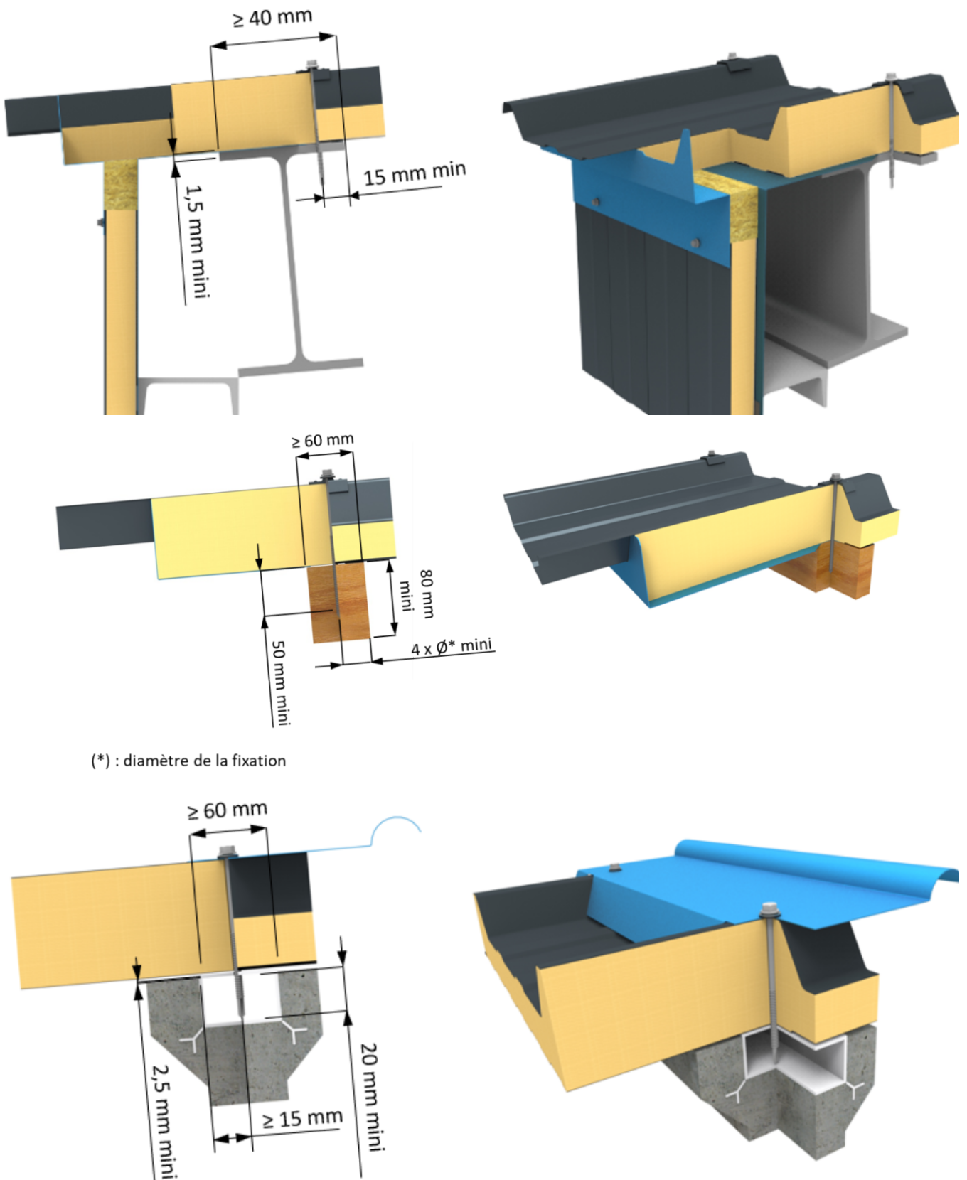
Figure 6 - Appuis d'extrémité
