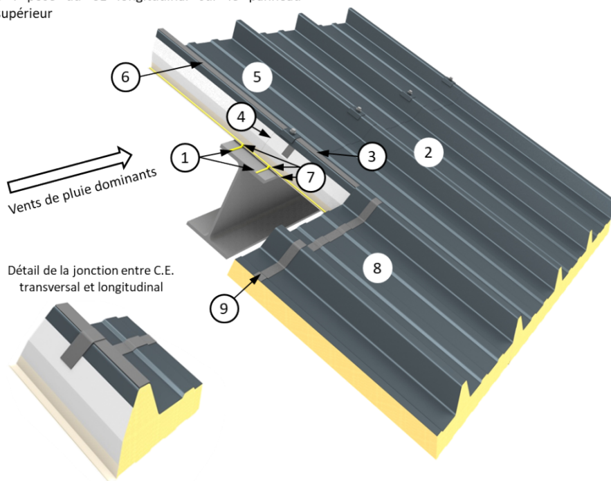
Figure 11 - Détail sur appui – Joints sur appui au droit d'un recouvrement transversal de panneaux avec Complément d'Etanchéité (C.E.) transversal et longitudinal - locaux climatisés (cf. §2.4.4)
