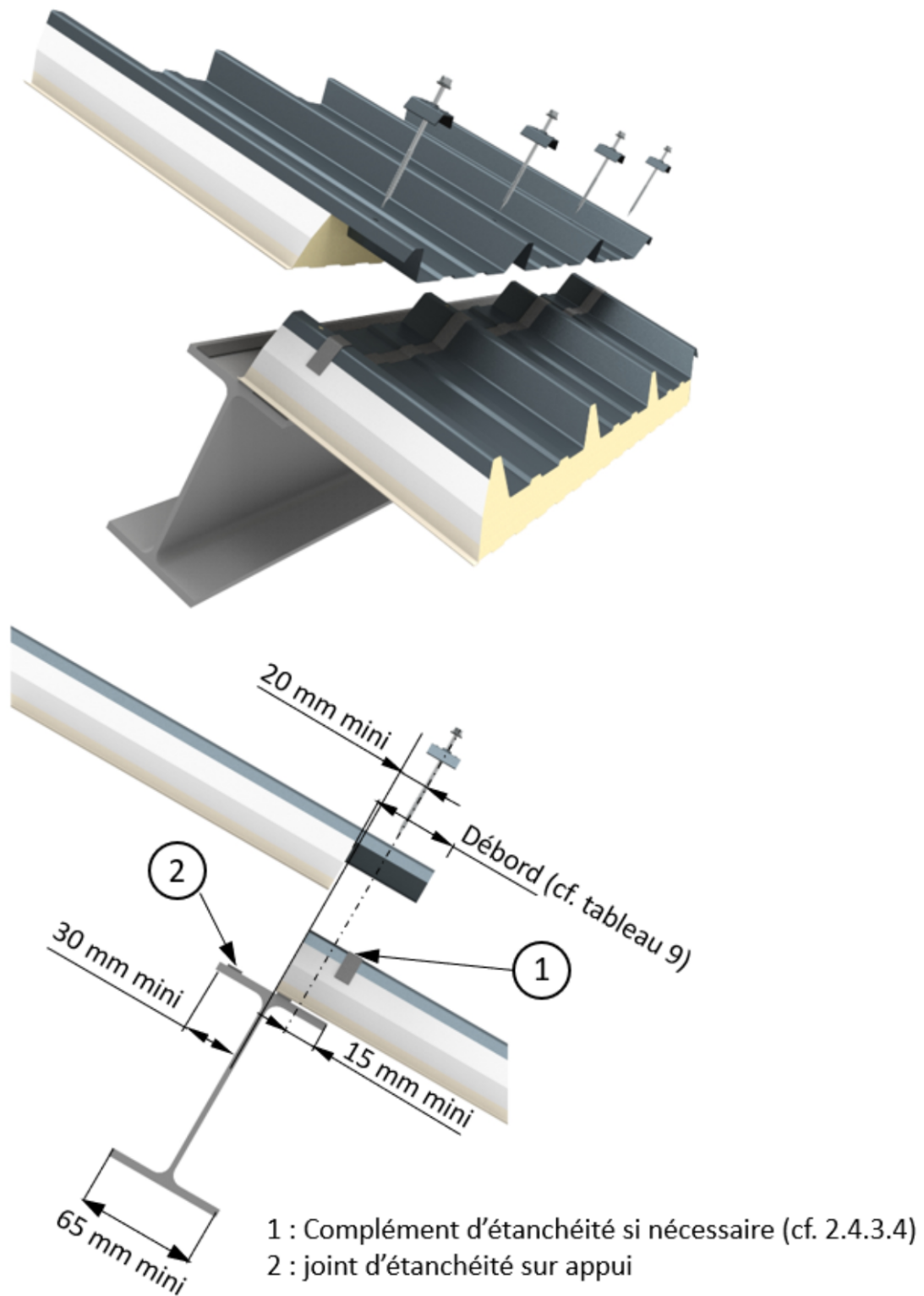
Figure 7 - Jonction transversale - cas sur support acier (cf. tableau 8)
