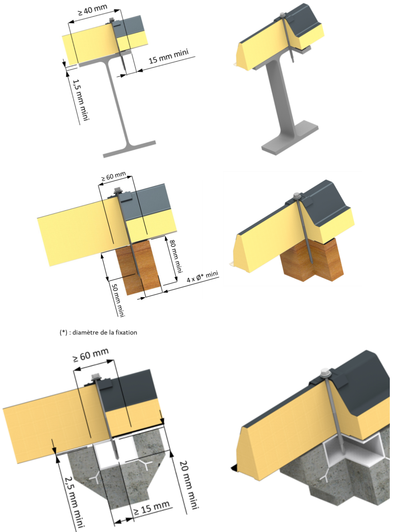
Figure 5 – Appuis intermédiaire
