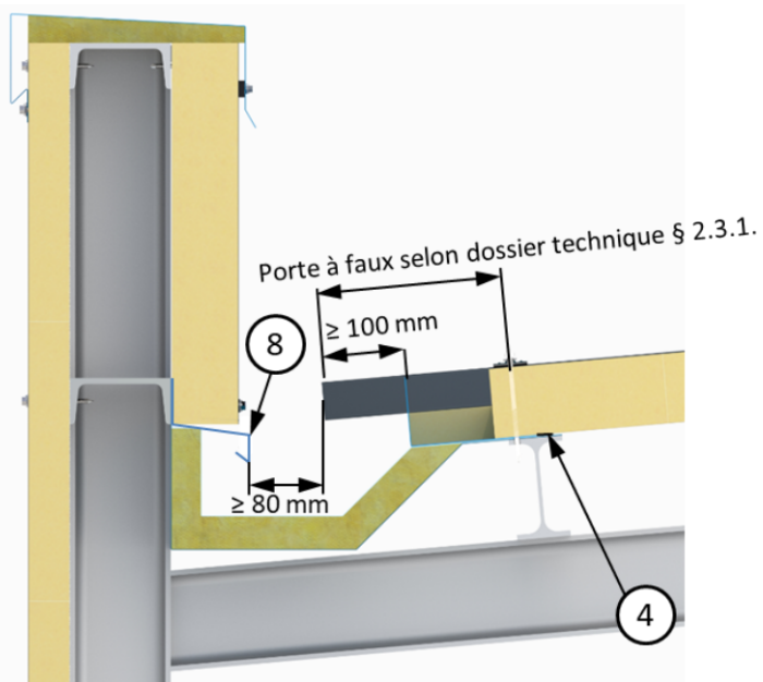
Figure 24 - Chéneau contre acrotère
