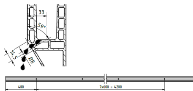
Figure 45 bis – EASY GLASS SMART latéral
