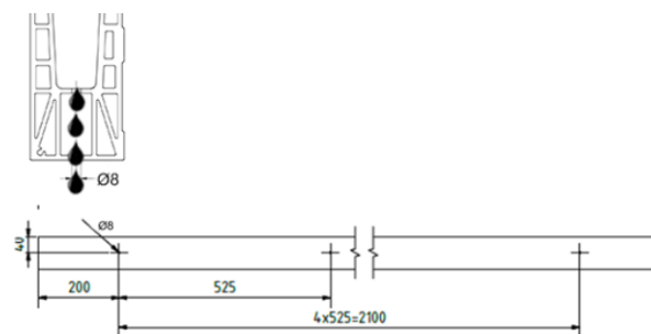
Figure 48 bis – EASY GLASS MAX latéral
