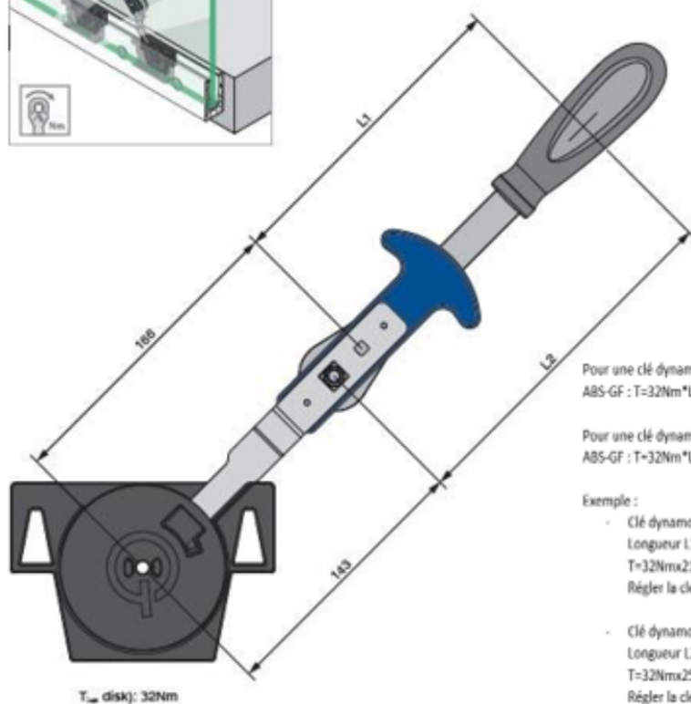
Figure 36 – Utilisation clé dynamométrique
