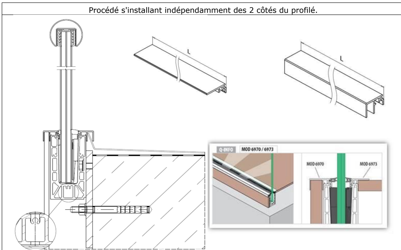
Figure 31 – Profils de raccords au sol
