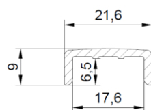
Figure 15 - Profilé de protection bord du vitrage
