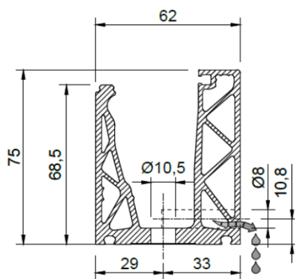
Figure 6 - Section transversale du profilé DFP88.60 avec indication de perçage pour drainage
