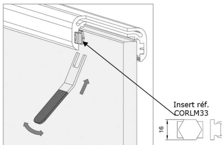
Figure 14 - Installation des mains courantes en aluminium avec clef en U réf. CORLM45
