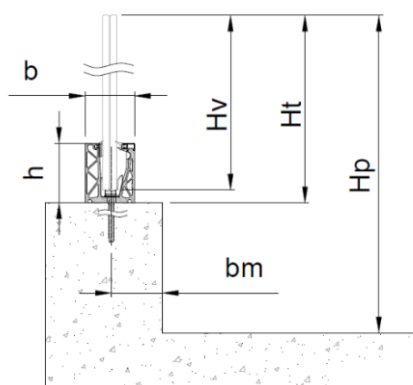
Figure 4 - Schéma en vue latérale du système DEFENDER DF88PICO
