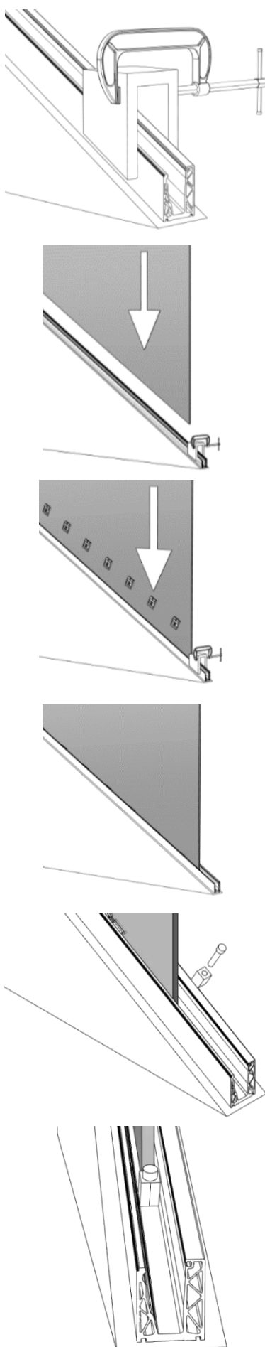
Figure 19 - Installation en rampant du système DEFENDER PICO avec calage provisoire et définitif
