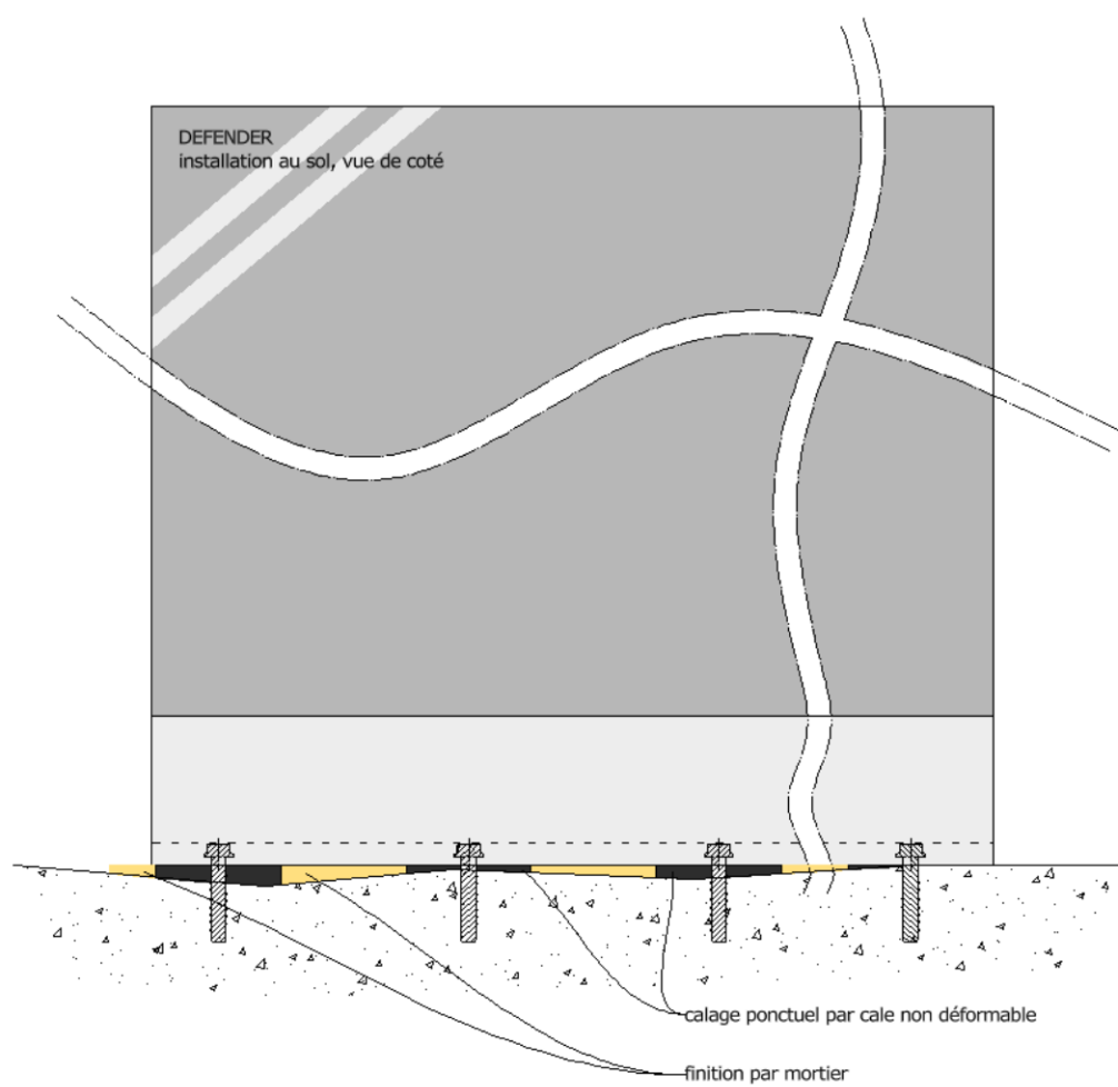
Figure 16 – Calage du système en cas de dalle irrégulière
