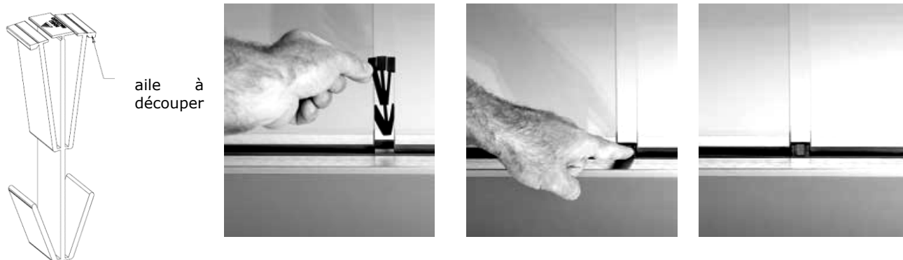
Figure 10 – Joint sapin pour bouchonner l'espace entre plaques de verre
