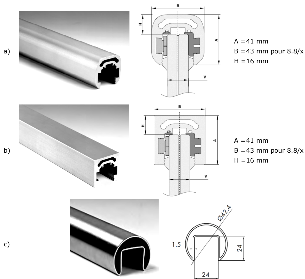
Figure 13 - Typologies de main courantes structurales en aluminium a) arrondi ou b) carré ou c) ronde INOX
