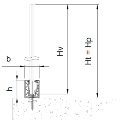
Figure 5 - Schéma en vue latérale du système DEFENDER DF88PICO
