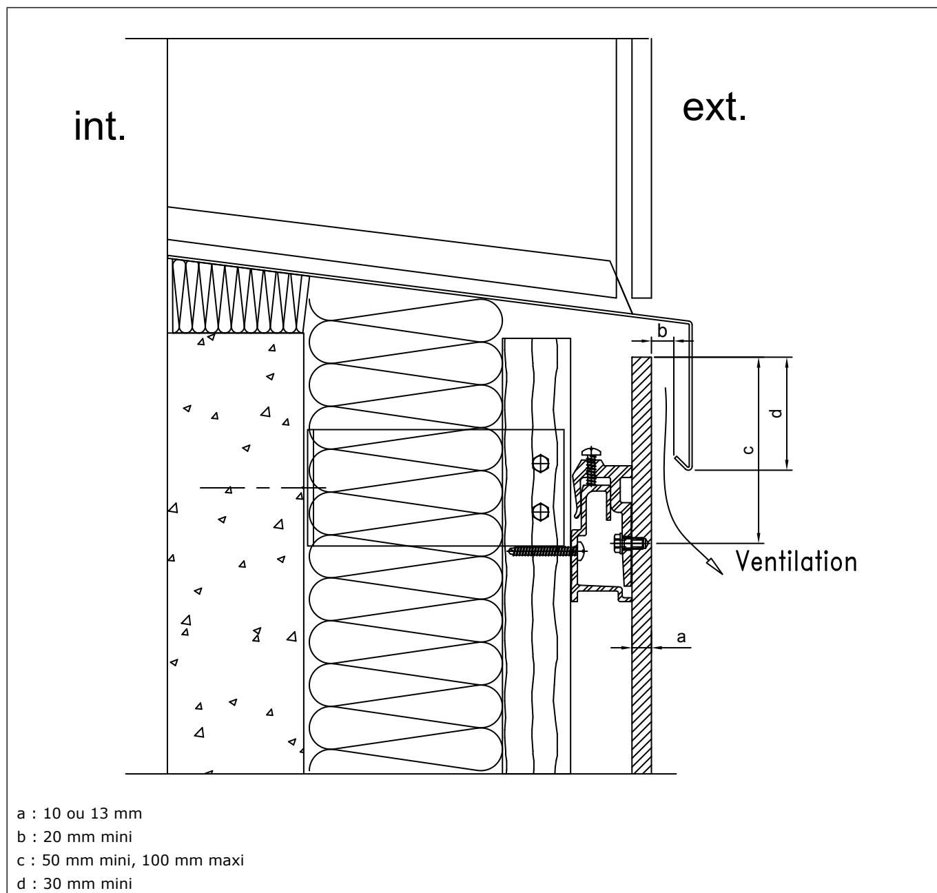
Figure 10 – Coupe sur appui
