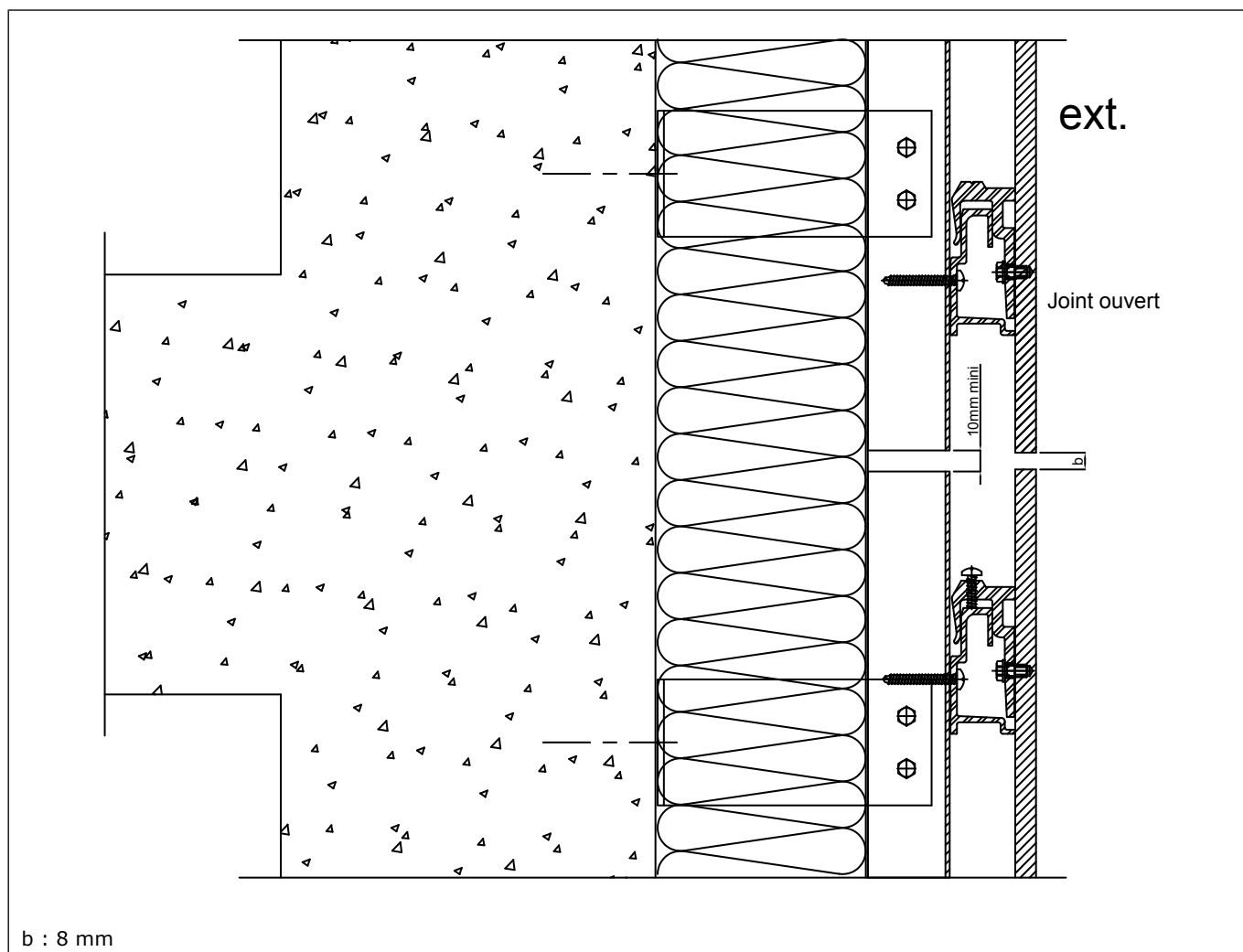
Figure B1 – Fractionnement au droit des planchers – ossature métallique
