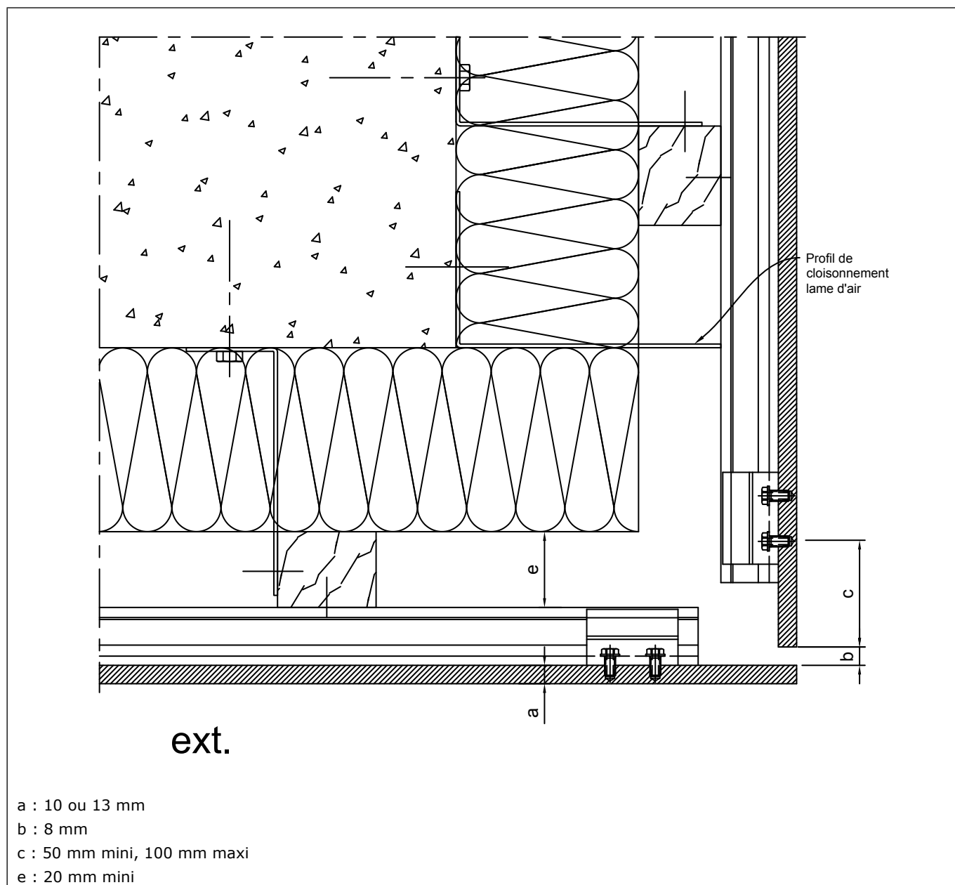
Figure 13 – Coupe sur angle sortant sur ossature bois
