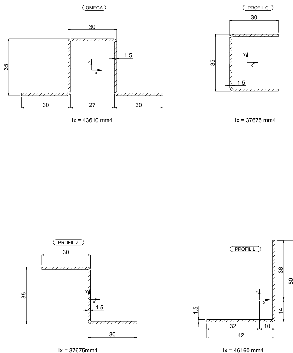
Figure 28 – Profilés en acier galvanisé 15/10 mini
