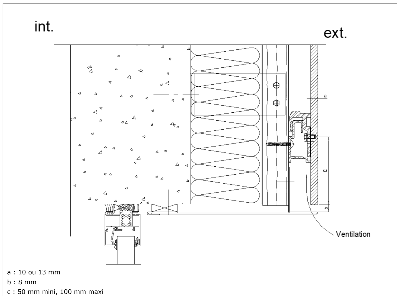
Figure 11 – Coupe sur linteau
