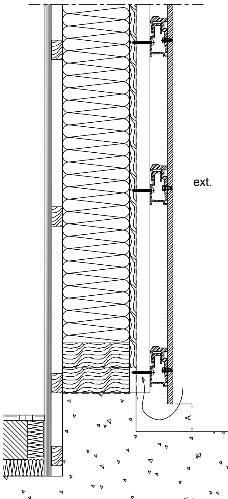
Figure 29 – Coupe verticale sur COB
