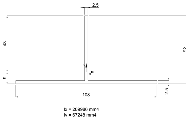
Figure 27 – Profilé aluminium ép. 2.5 mm min
