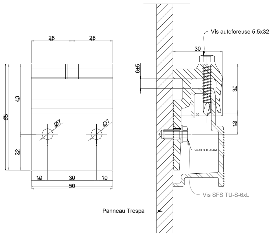
Figure 3 – Patte-agrafe TSP 205 réglable avec taraudage
