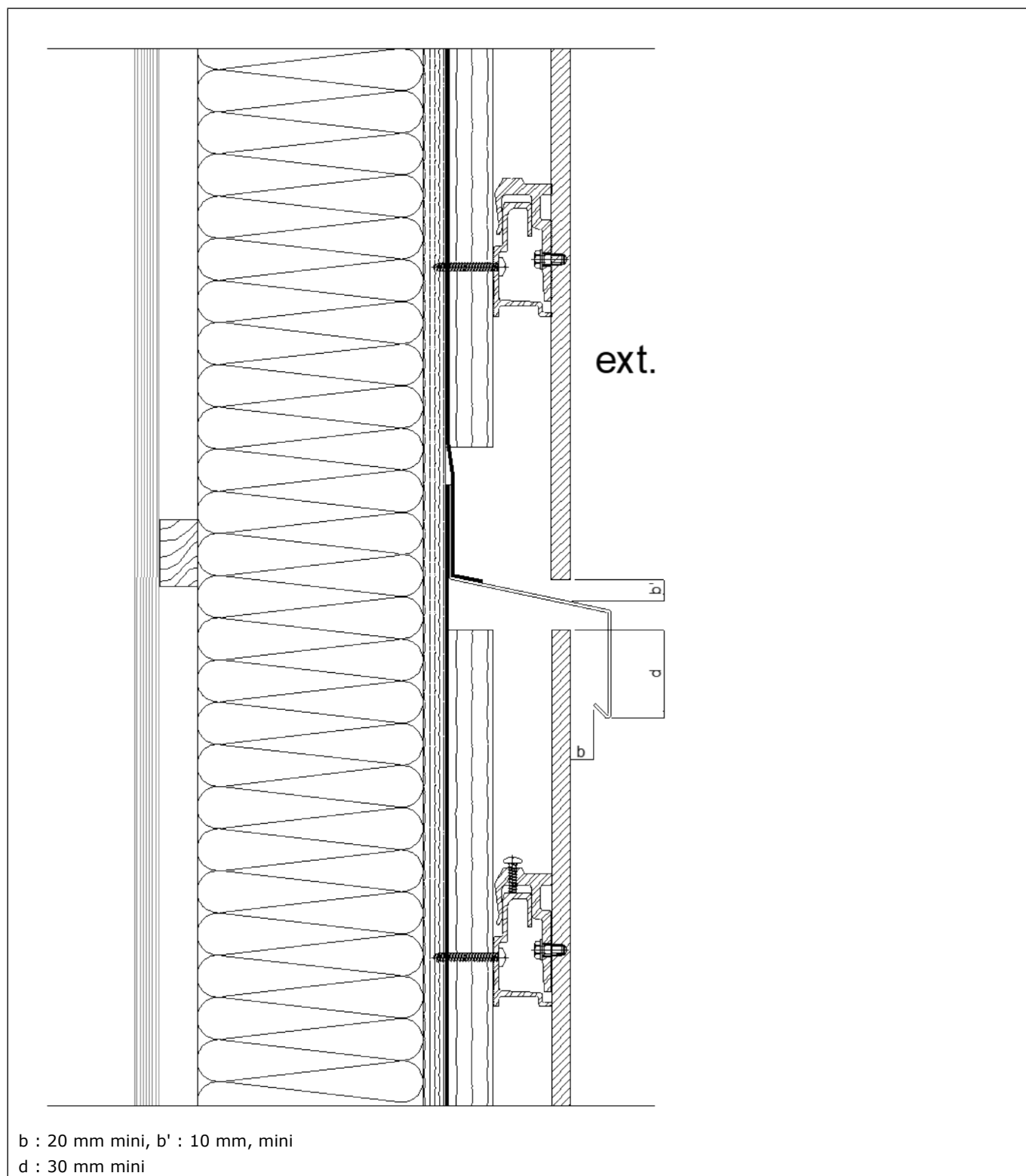
Figure 31 – Recoupement du pare-pluie tous les 6 m
