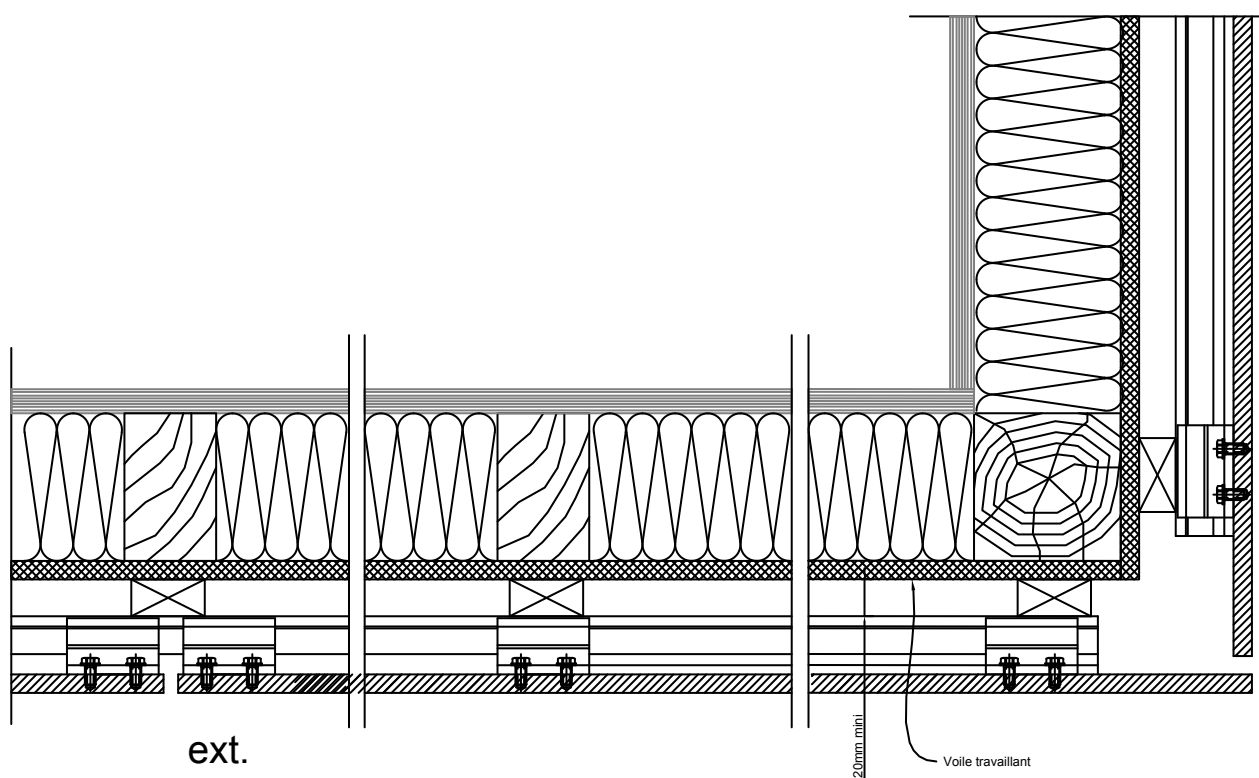
Figure 30 – Coupe horizontale sur COB
