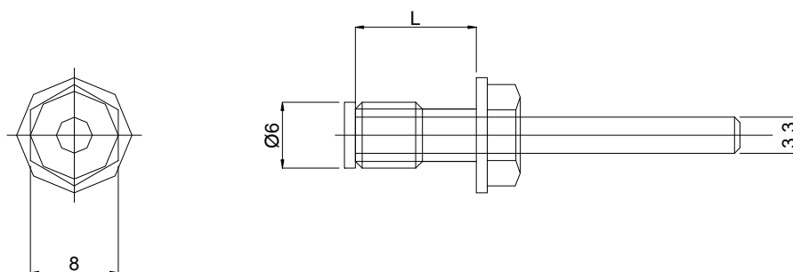
Figure 3 – Patte-agrafe TSP 205 réglable avec taraudage
