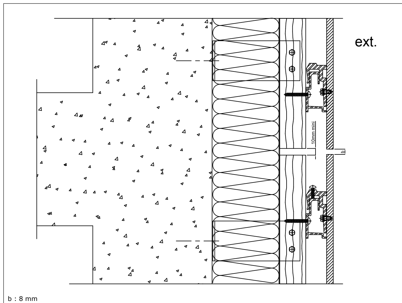
Figure A1 – Fractionnement au droit des planchers – ossature bois
