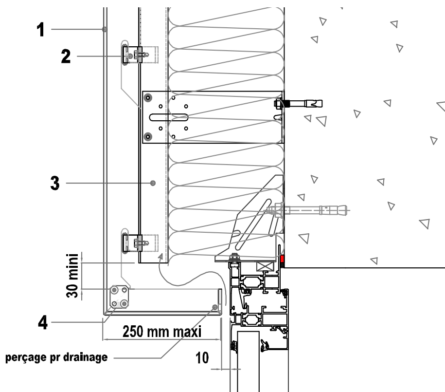
Figure 9 – Linteau de baie – Coupe verticale – Mise en œuvre avec profilé LCH-1
