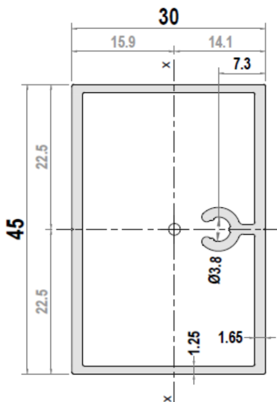
Figure 3b – Fixation déportée rivetée (pour tableau ou JD pour le sismique)
