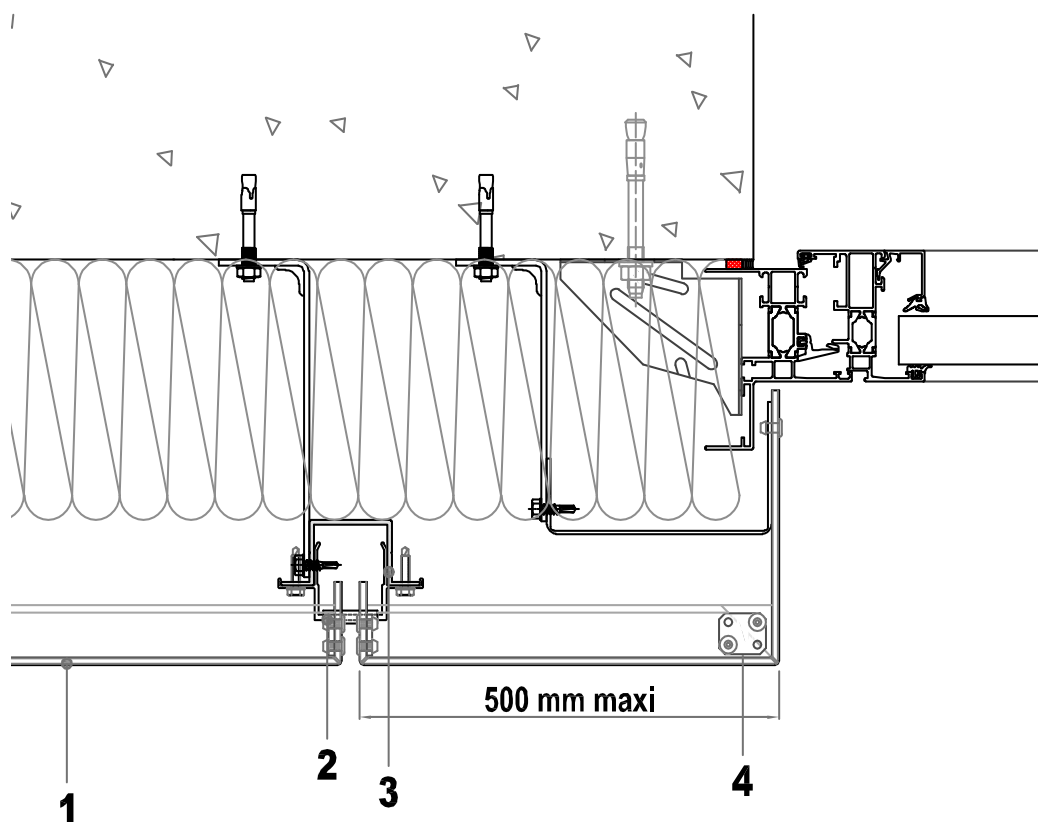
Figure 13b – Tableau de baie – Coupe horizontale – Mise en œuvre avec profilé LCH-1
