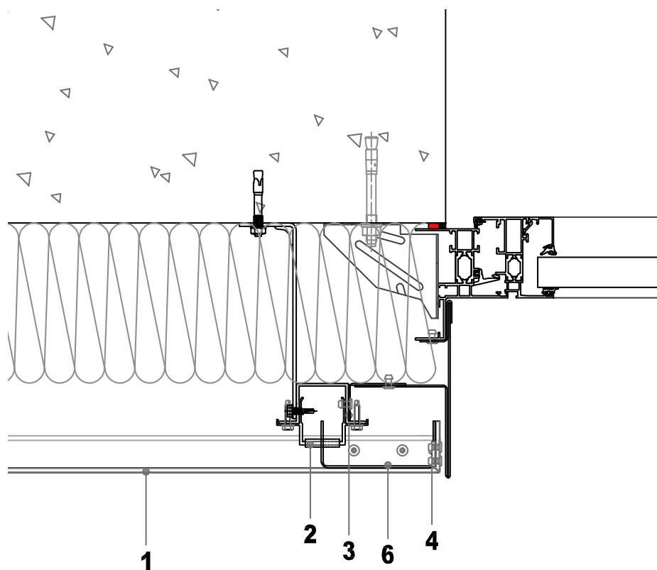
Figure 13a – Tableau de baie – Coupe horizontale – Mise en œuvre avec profilé LCH-1
