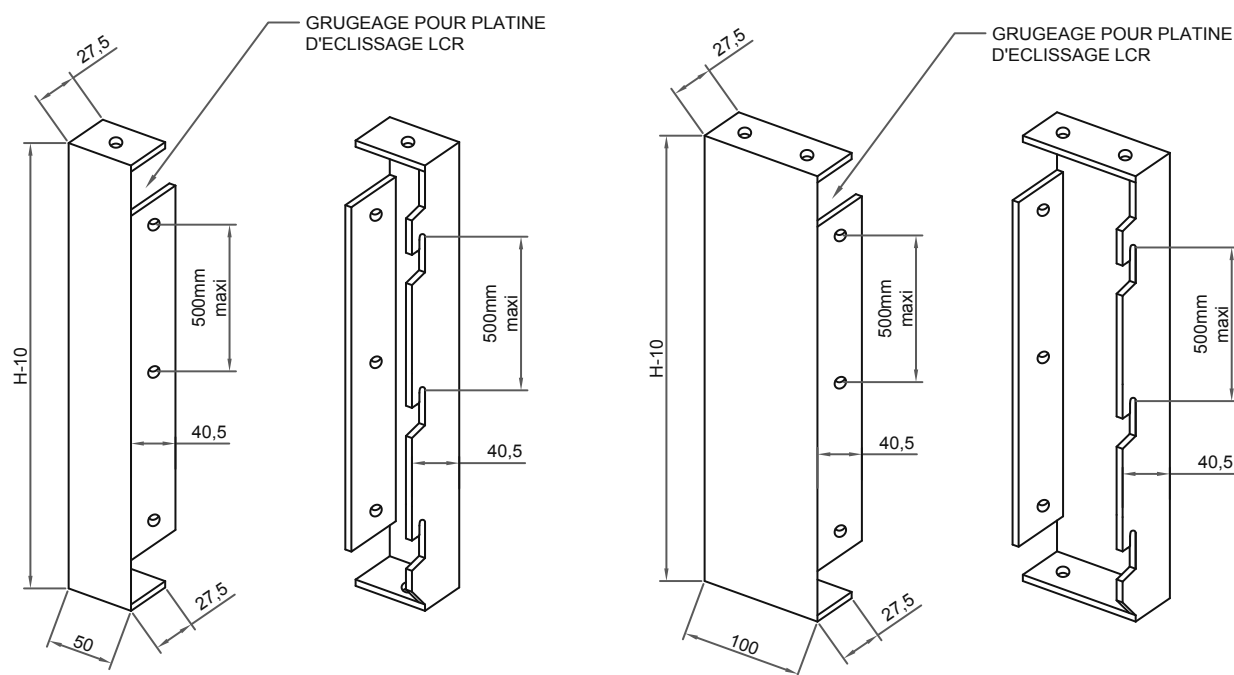
Figure 3b – Fixation déportée rivetée (pour tableau ou JD pour le sismique)
