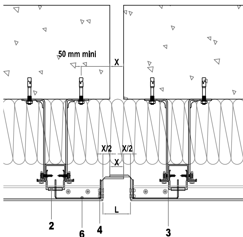
Figure A2 – Joint de dilatation compris entre 12 et 15 cm avec fixation déportée rivetée
