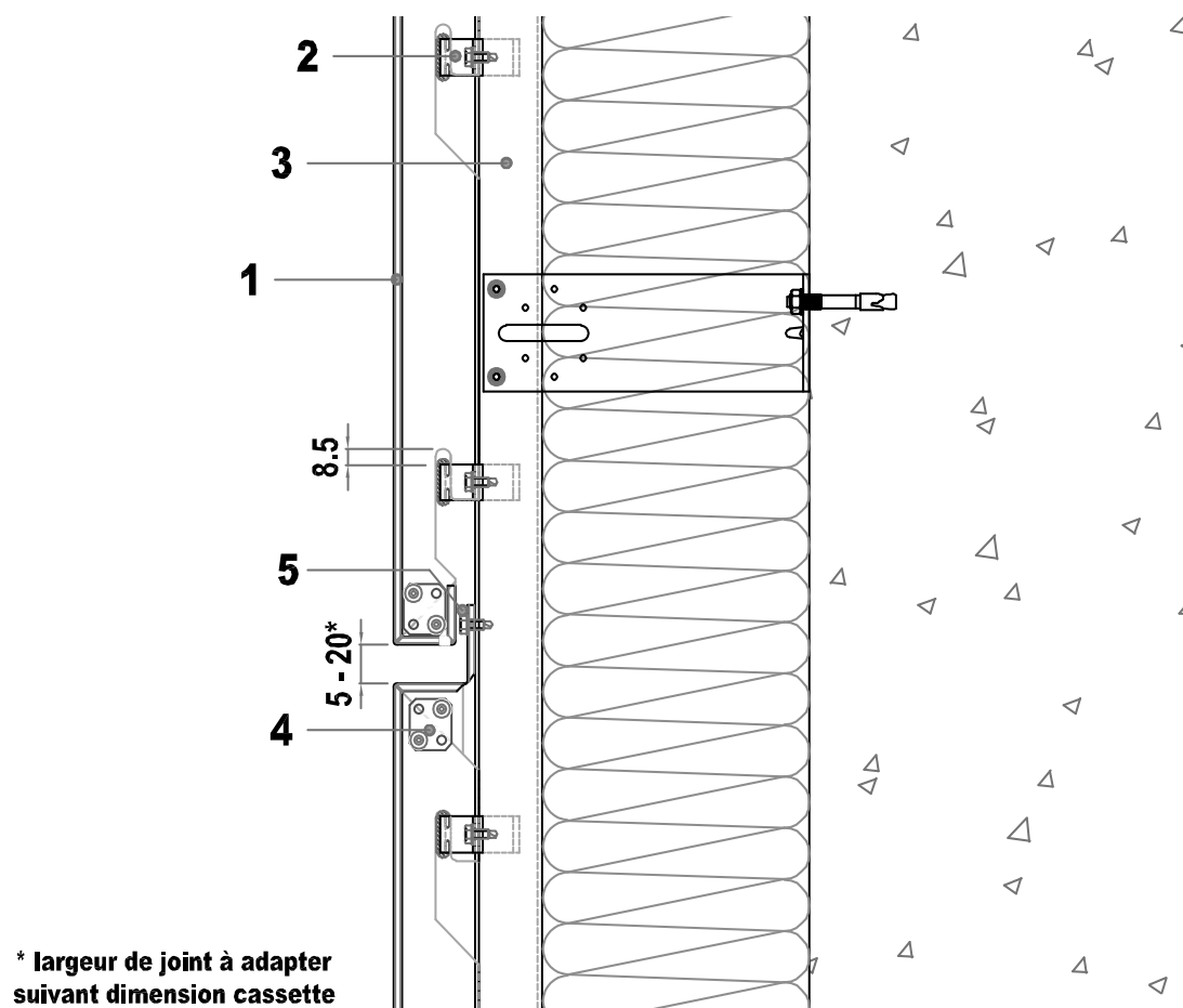
Figure 7 – Joint horizontal - coupe verticale - Mise en œuvre avec profilé LCH-1
