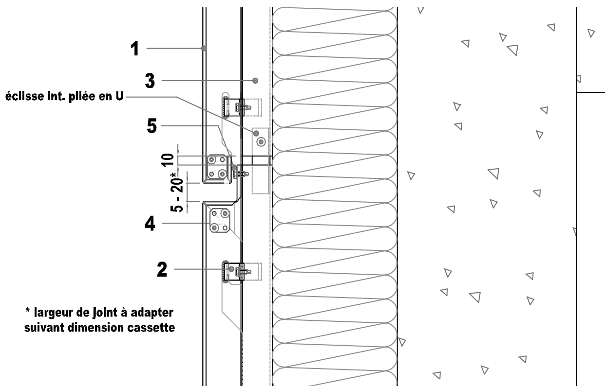
Figure 10 – Fractionnement de l'ossature – Coupe verticale – Mise en œuvre avec profilé LCH-1
