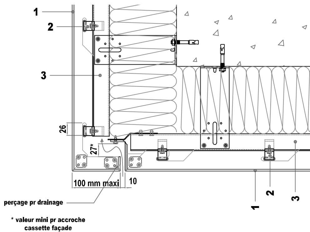
Figure 16 – Jonction bardage / sous-face
