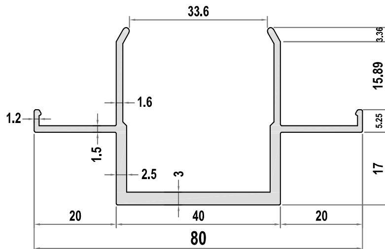
Figure 5c – Description de la pièce de suspension LC-3
