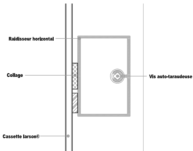
Figure 3c – Raidisseur horizontal LC-RH collé
