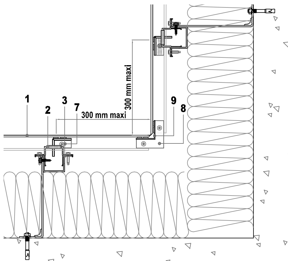
Figure 15b - Angle rentrant – Coupe horizontale – Mise en œuvre avec profilé LCH-1
