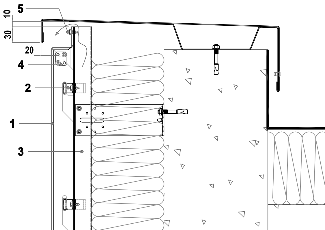
Figure 11 – Acrotère – Coupe Verticale – Mise en œuvre avec profilé LCH-1
