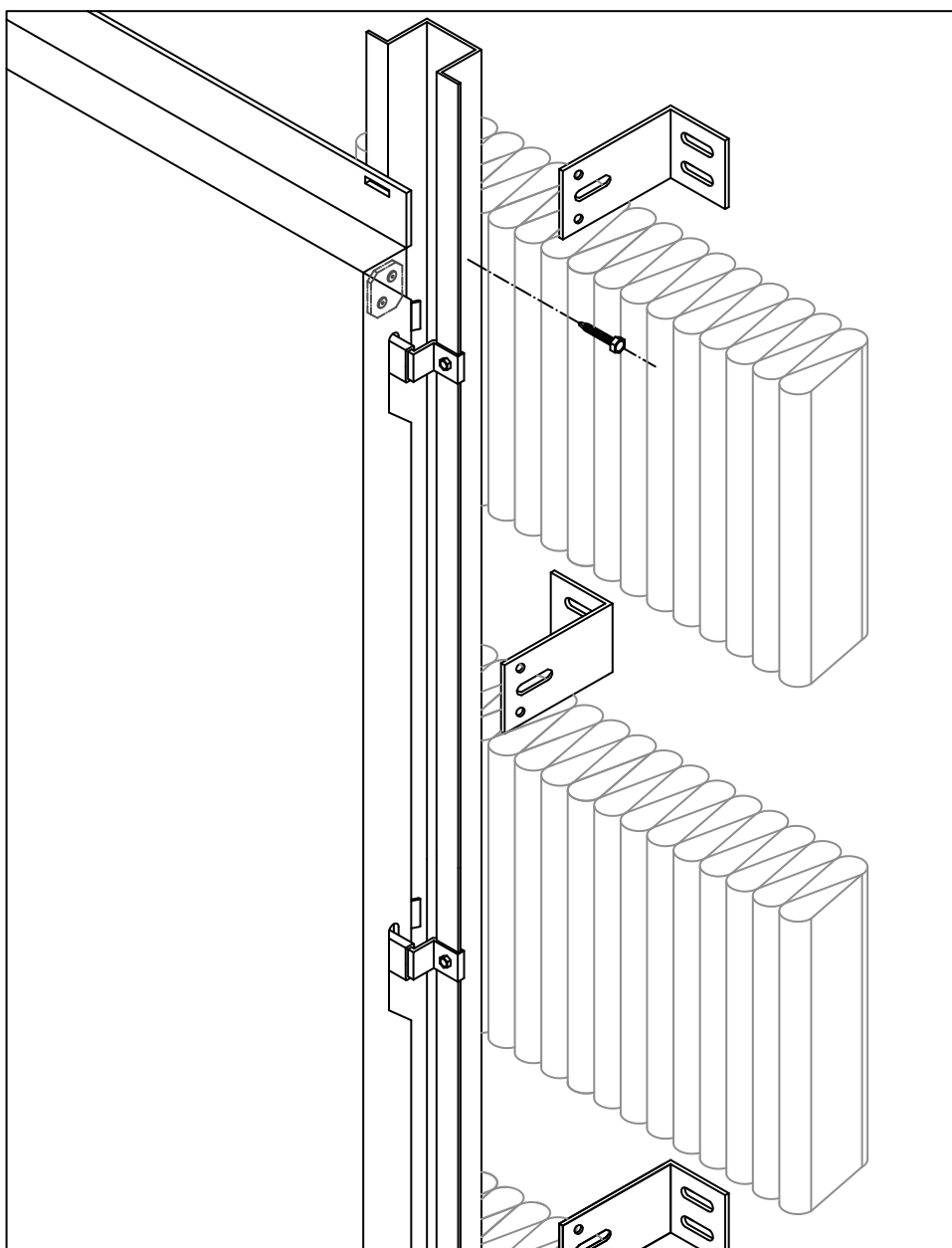
Figure 1 – Présentation générale système LCH-1
