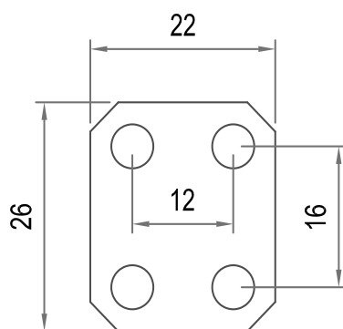
Figure 4a – LCR - Platine d'éclissage
