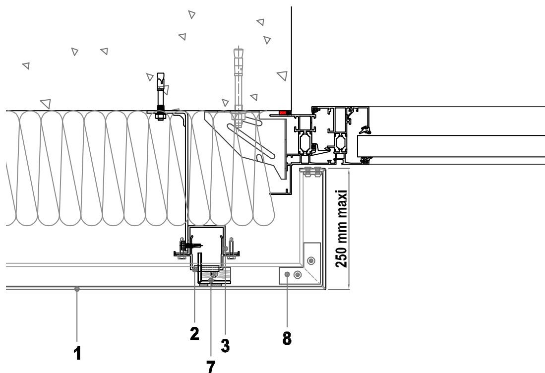
Figure 13c – Tableau de baie – Coupe horizontale – Mise en œuvre avec profilé LCH-1
