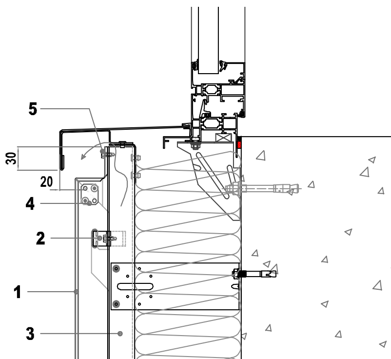
Figure 8 – Appuis de baie – Coupe verticale – Mise en œuvre avec profilé LCH-1
