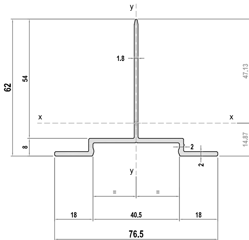
Figure 5c – Description de la pièce de suspension LC-3
