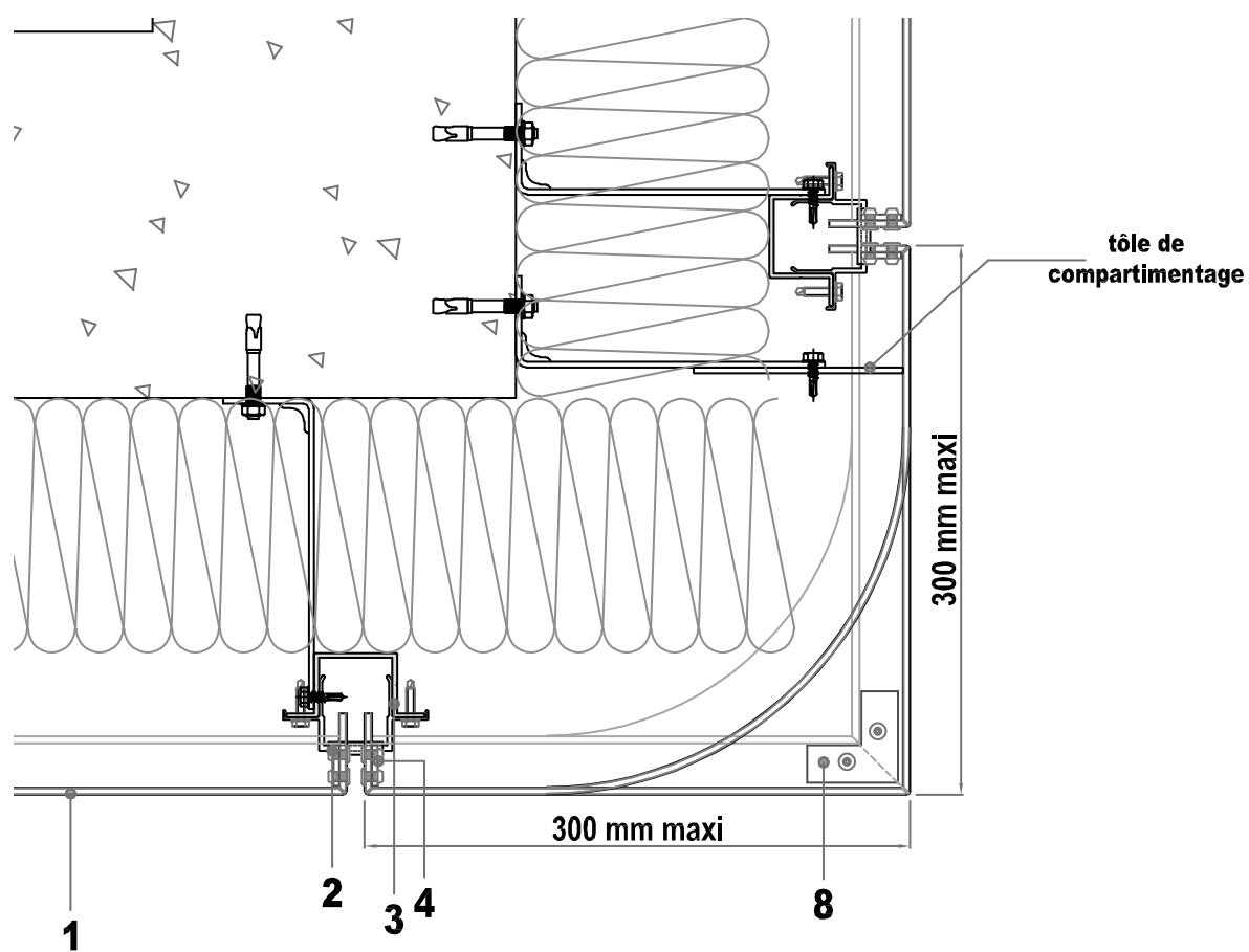
Figure 14a – Angle sortant – Coupe horizontale avec profilé LCH-1
