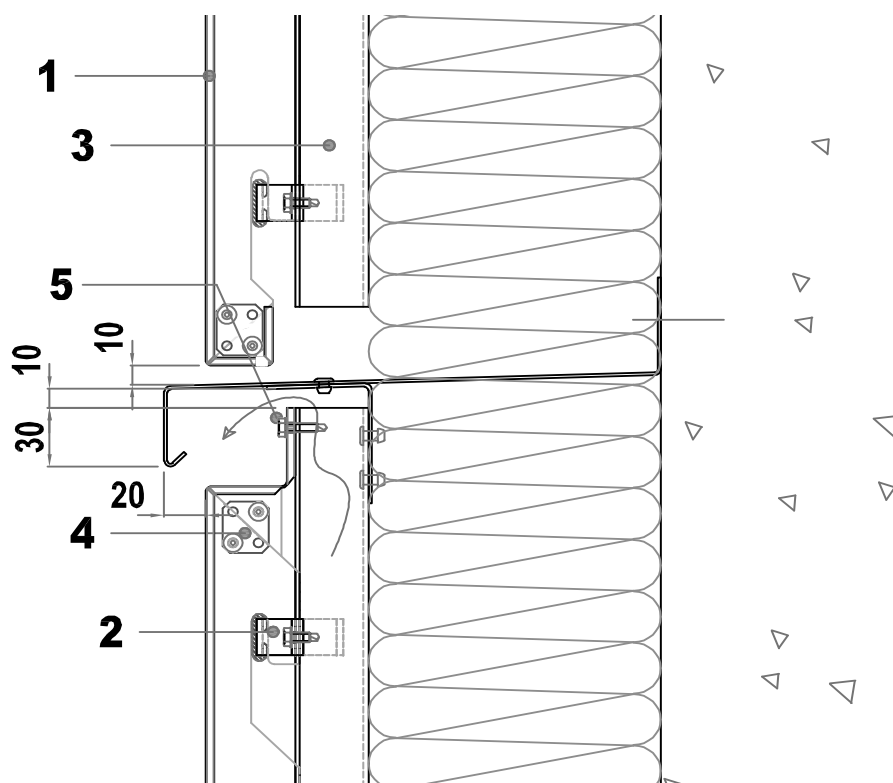
Figure 17 – Recouvrement de la lame d'air
