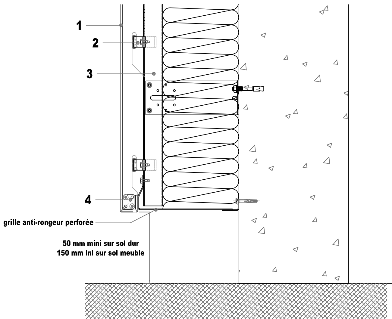
Figure 5e – Description de la pièce de suspension LC-3T
