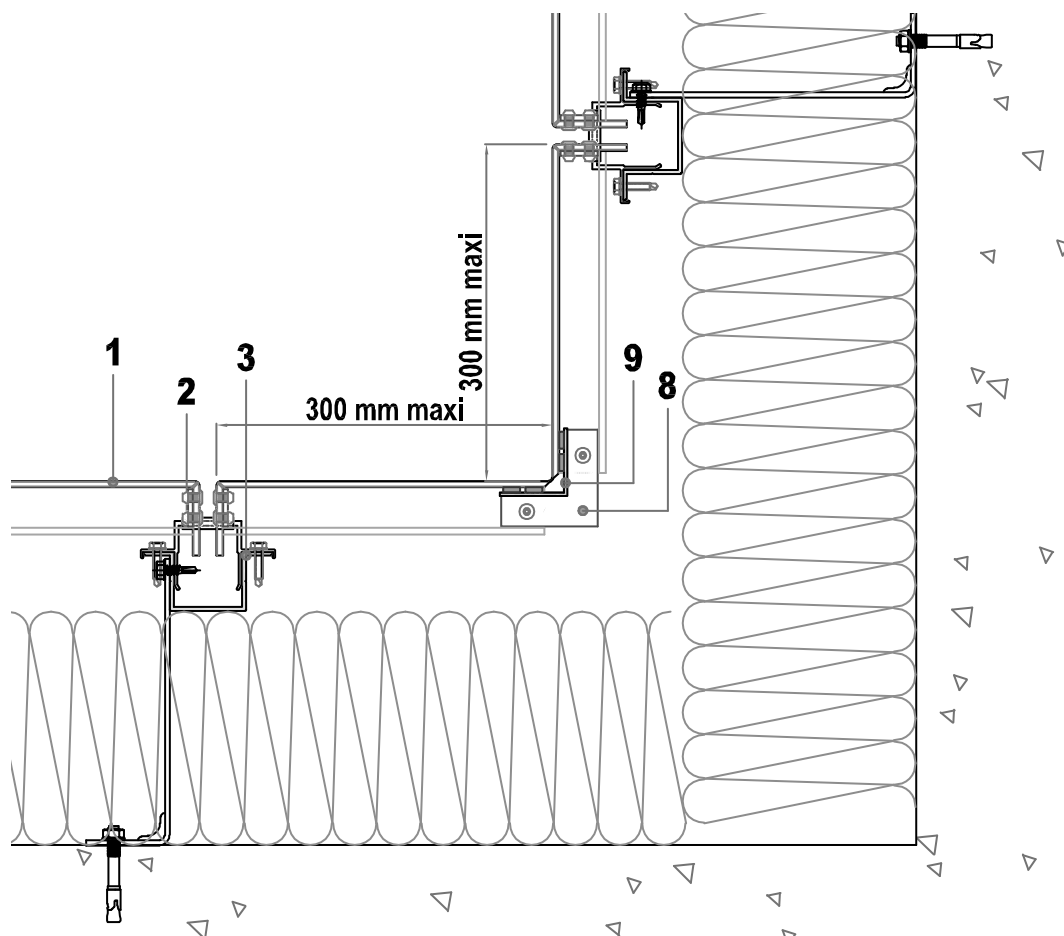
Figure 15a - Angle rentrant – Coupe horizontale – Mise en œuvre avec profilé LCH-1
