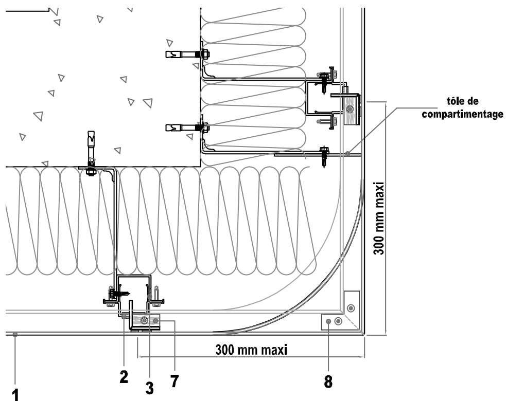
Figure 14b – Angle sortant – Coupe horizontale avec profilé LCH-1
