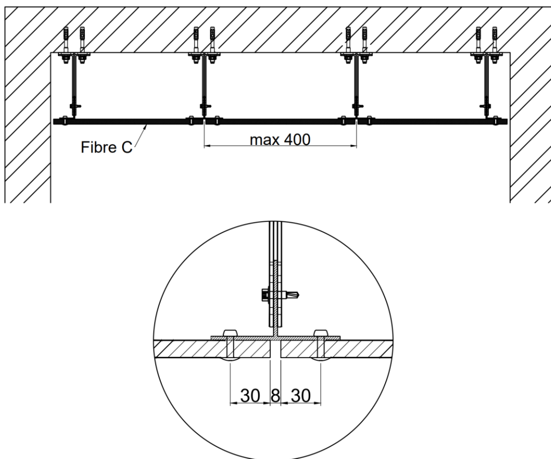
Figure 10bis – Pose en habillage de sous-face
