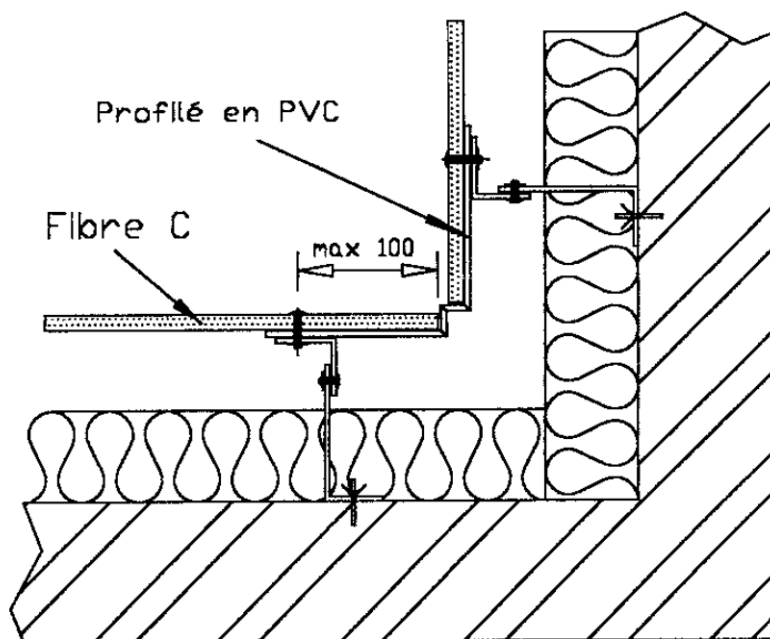
Figure 15bis – Angle rentrant avec profilé en PVC
