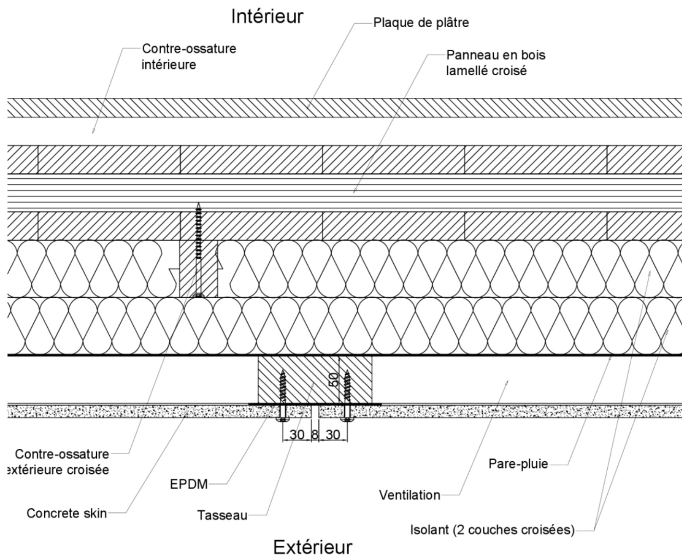
Figure 26 – Pose sur CLT – coupe horizontale
