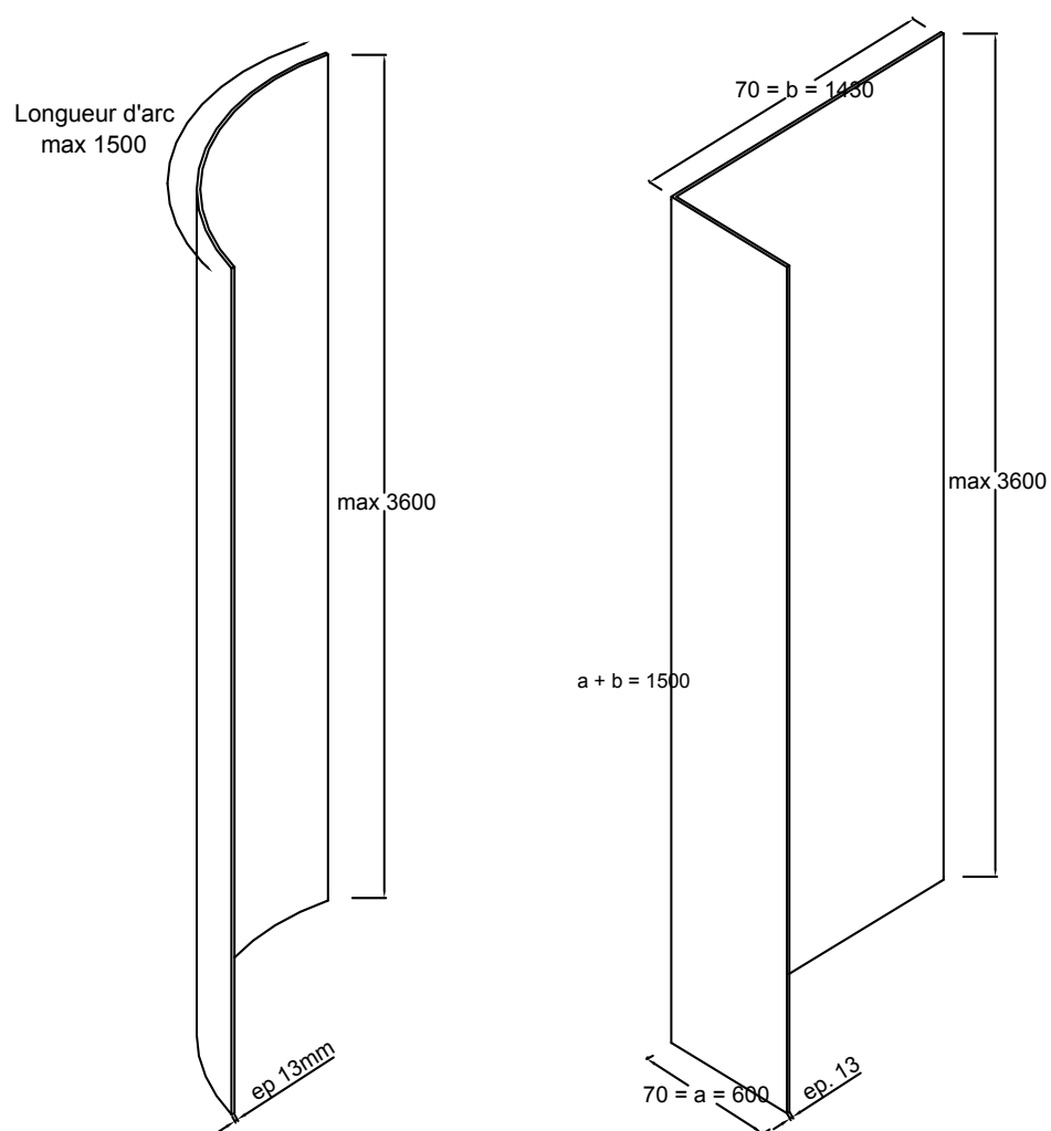
Figure 6 – Exemple de panneaux d'angle Fibre C concrete skin et öko skin formés sur gabarit
