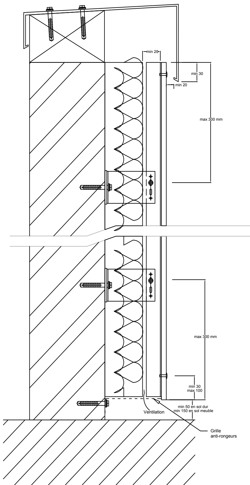
Figure 9 – Rive haute et rive basse
