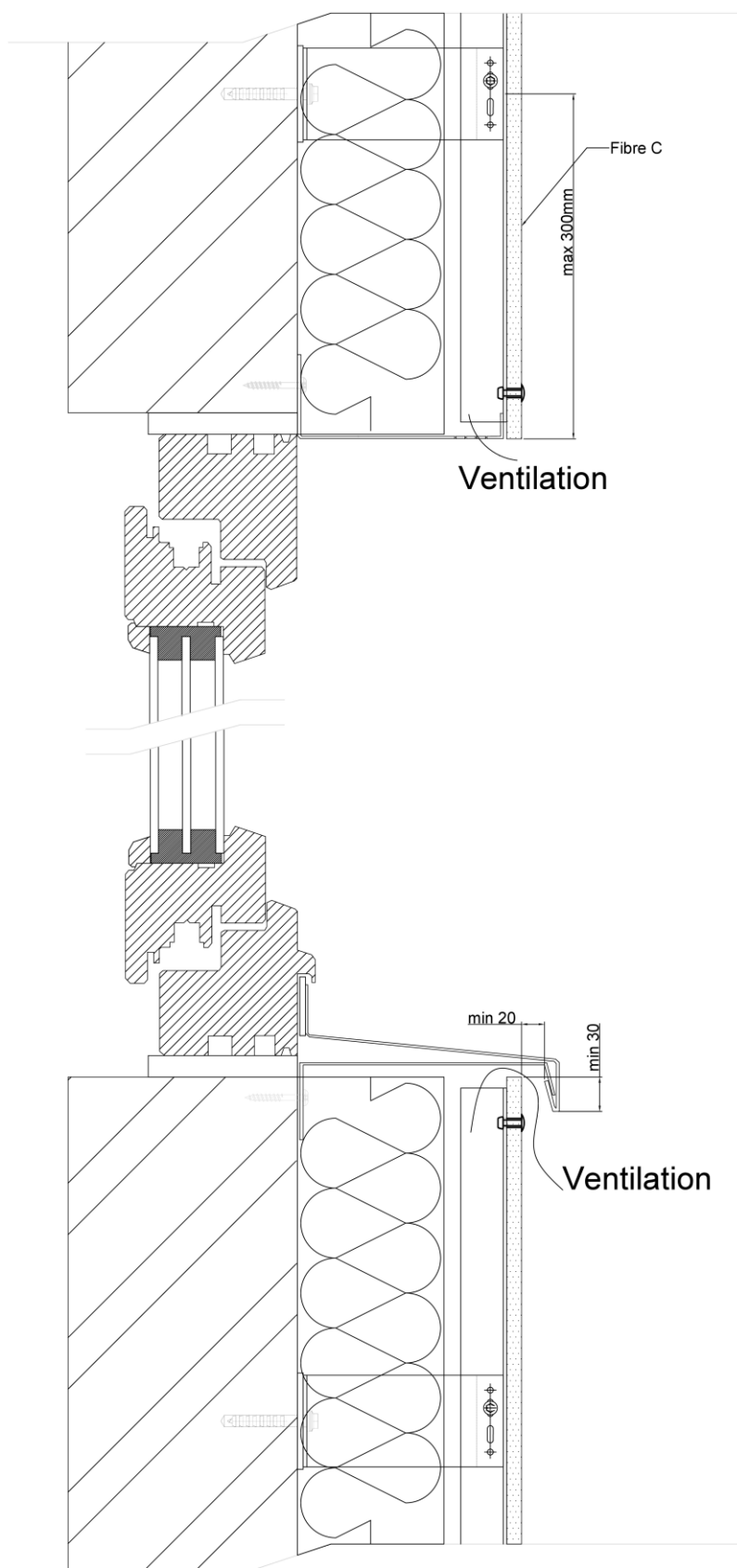
Figure 10 – Encadrement de fenêtre
