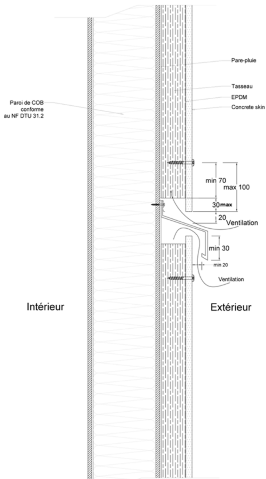
Figure 24 – Pose sur COB – Recouvrement du pare-pluie tous les 6m
