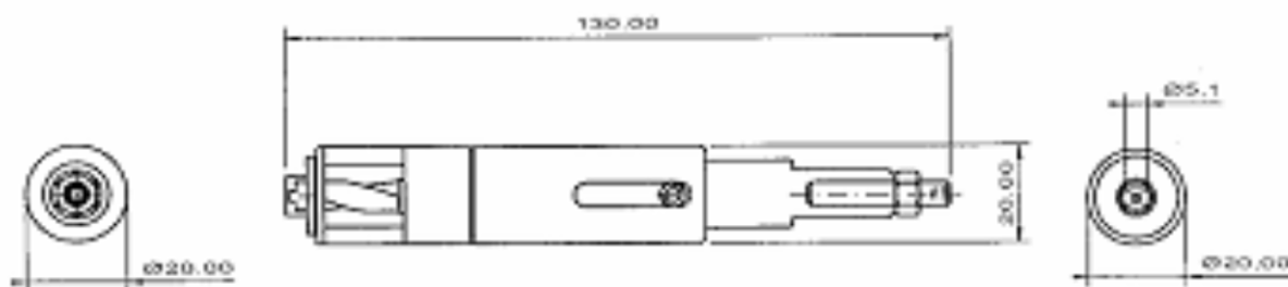
Figure 5 - Outil de centrage pour rivets
