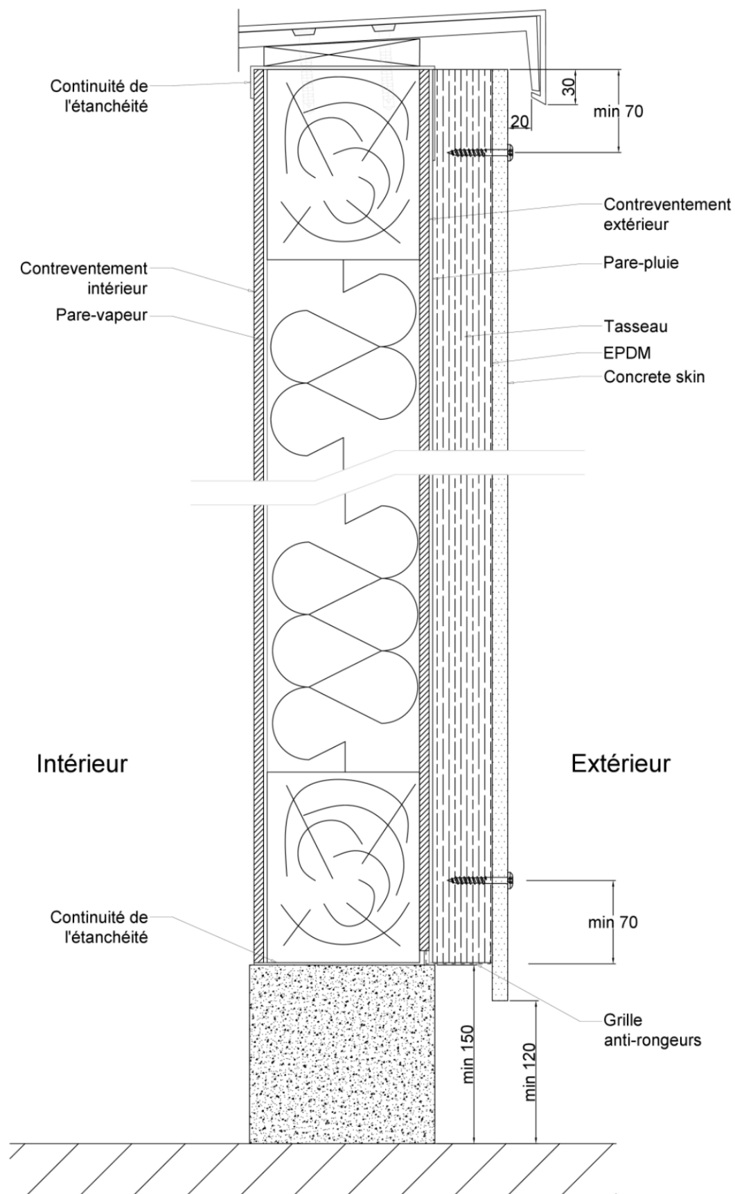
Figure 23 – Pose sur COB – Coupe verticale simple réseau
