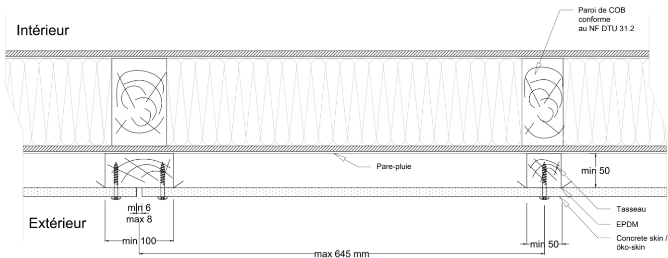
Figure 22 – Pose sur COB – Coupe horizontale avec tasseau
