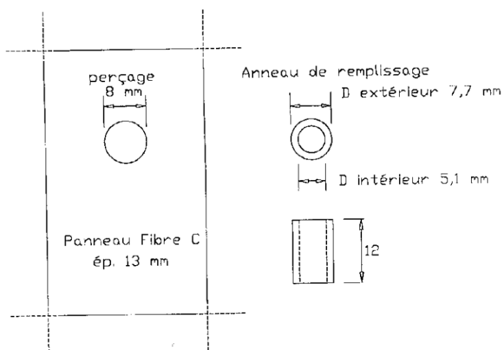
Figure 1ter – Réalisation du point fixe
