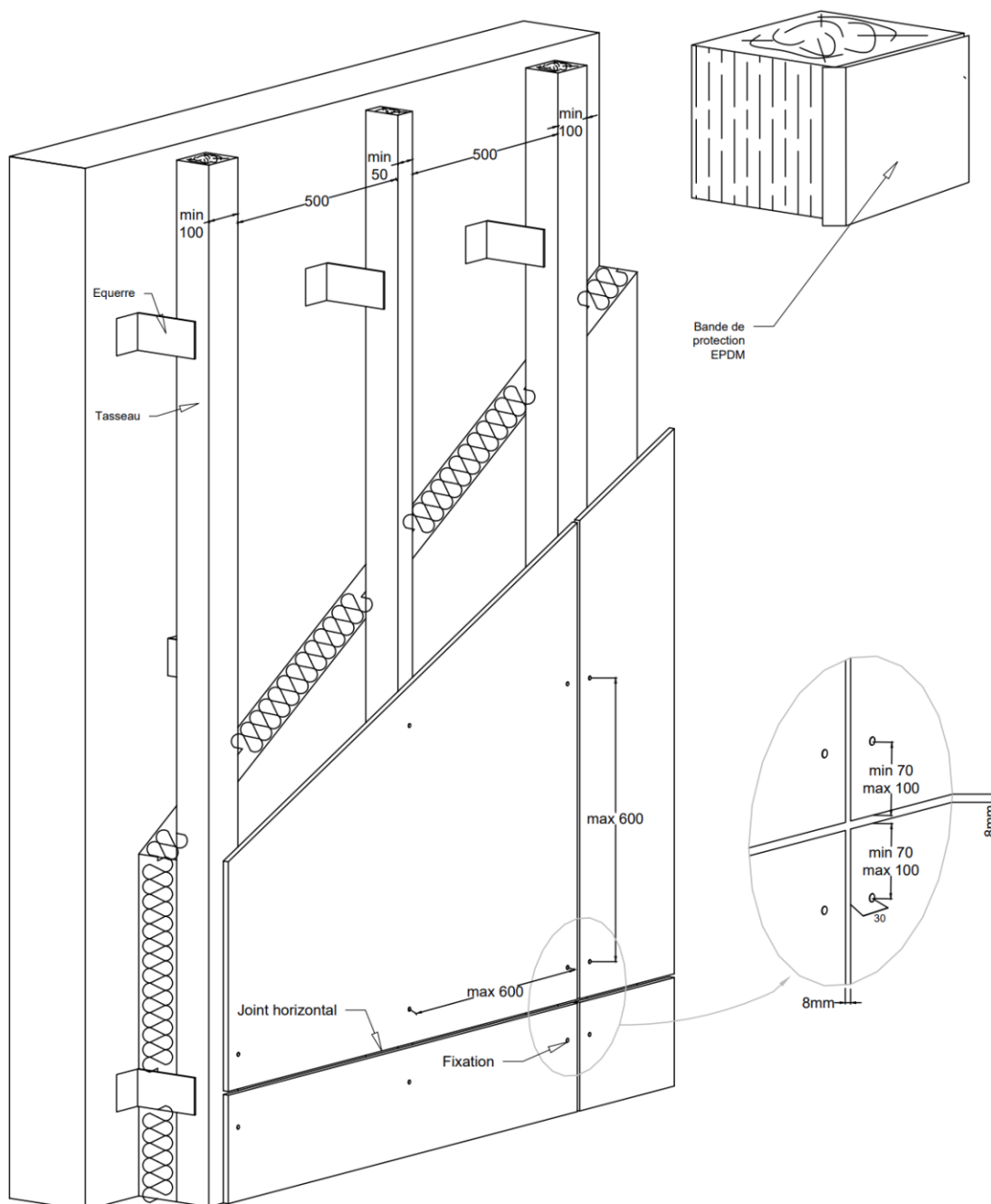
Figure 17 – Principe de mise en œuvre sur ossature bois
