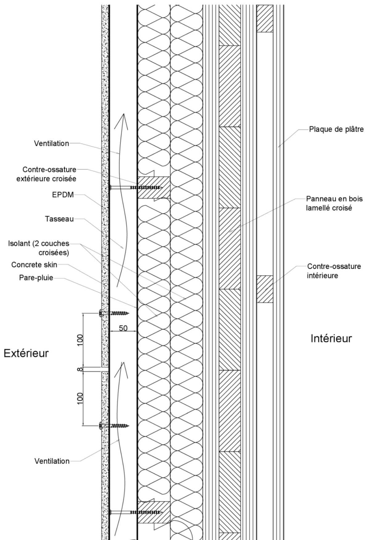
Figure 25 – Pose sur CLT – coupe verticale
