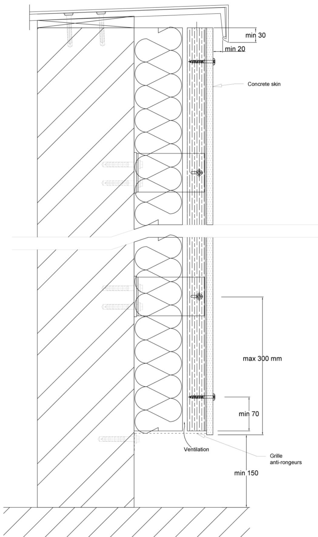
Figure 18 – Rive haute et rive basse ossature bois
