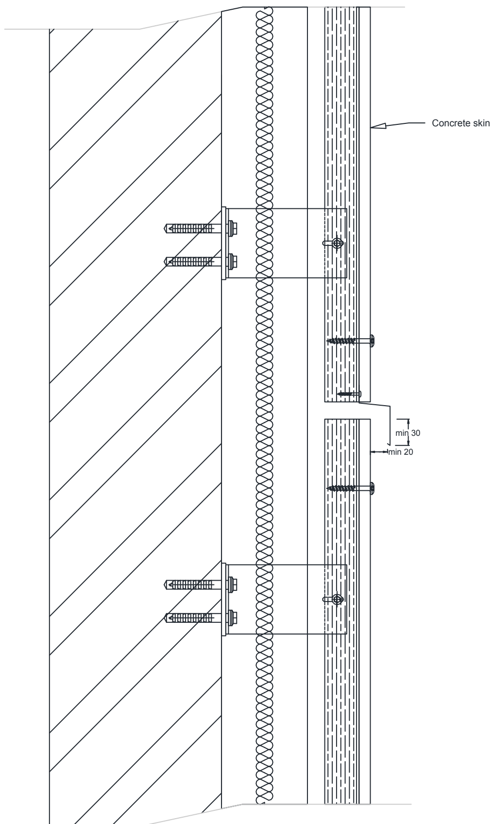
Figure 19 – Fractionnement de l'ossature bois (longueur > 5,4 m)
