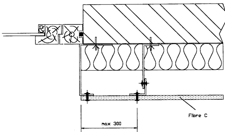
Figure 11 – Encadrement de fenêtre (coupe sur tableau)
