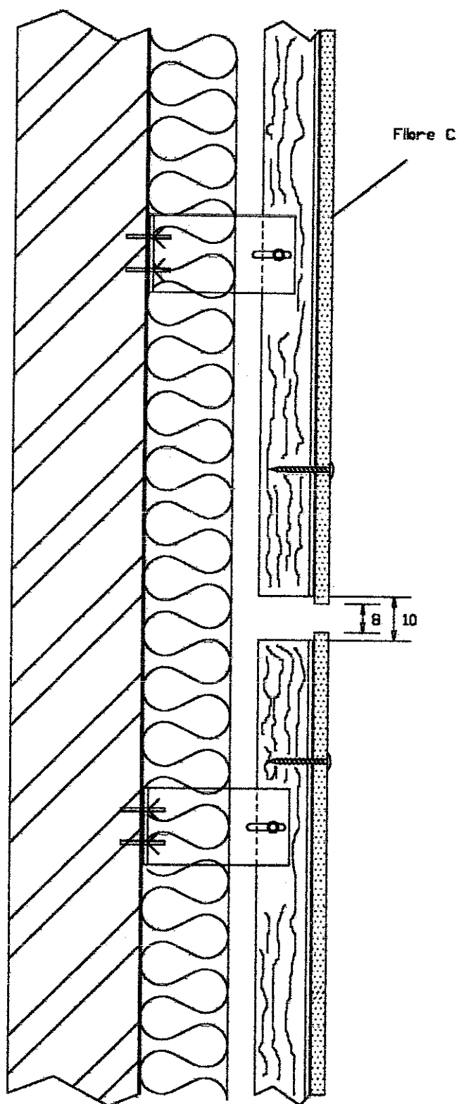
Figure 19bis – Fractionnement de l'ossature bois (longueur \leq 5,4 m)
