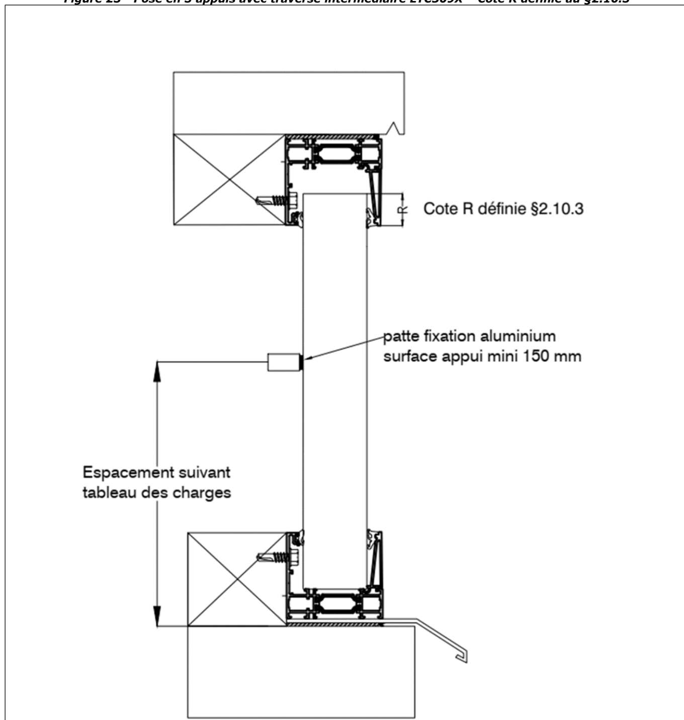
Figure 23 - Pose en 3 appuis avec traverse intermédiaire LTC509X – Côte R définie au §2.10.3
