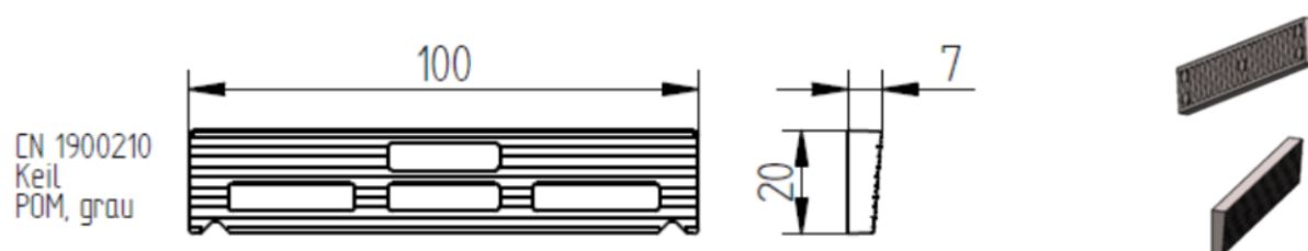
Figure 12 – Cale de serrage POM pour CROSILUX 1.0 CN 1900210
