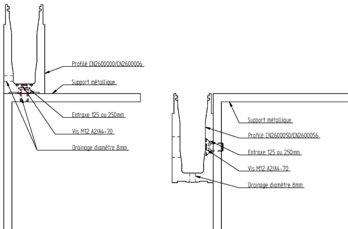
Figure 9 – CROSILUX 2.0 – Montage sur structure métallique
