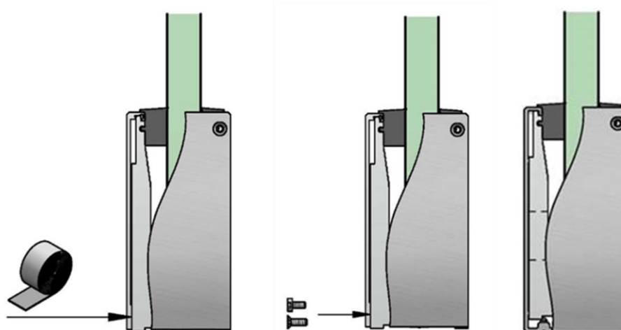
Figure 13b – Fixation de la tôle d'habillage sur le profilé de maintien CROSILUX 2.0 sur dalle et en nez de dalle
