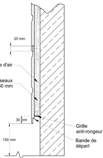
Maçonnerie
