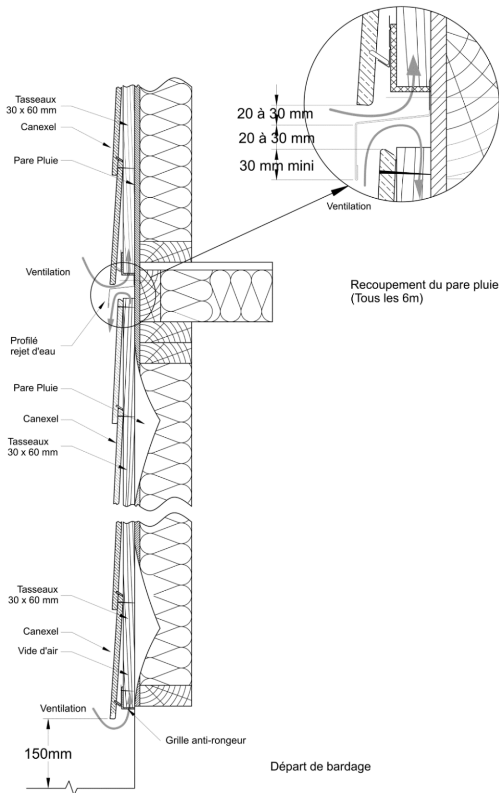
Figure 25 – Coupe verticale sur COB
