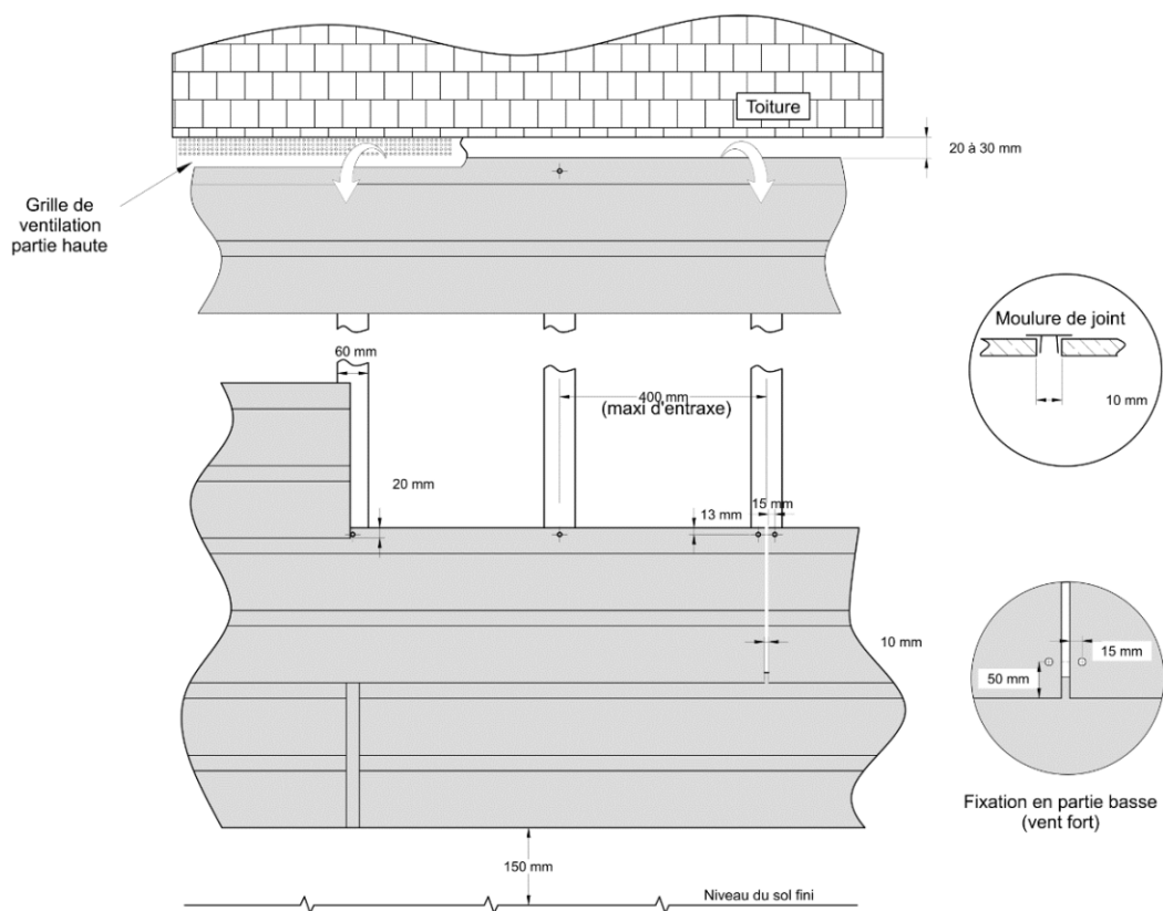
Maison Ossature Bois (Pose en double réseau)
