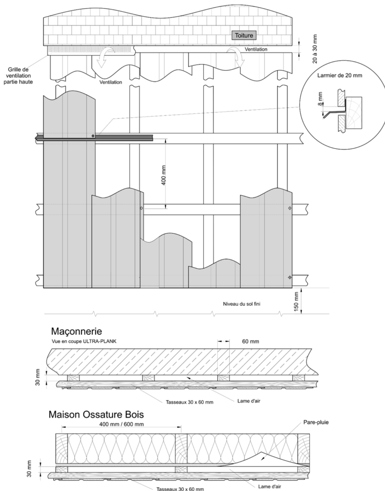
Figure 6 – Pose verticale ULTRA-PLANK® / RIDGEWOOD® / VSTYLE® Ossature double réseau avec larmier
