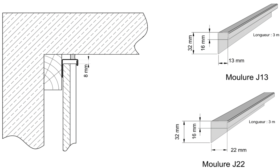
Figure 11 – Arrêt latéral sur revêtement – Moulure J
