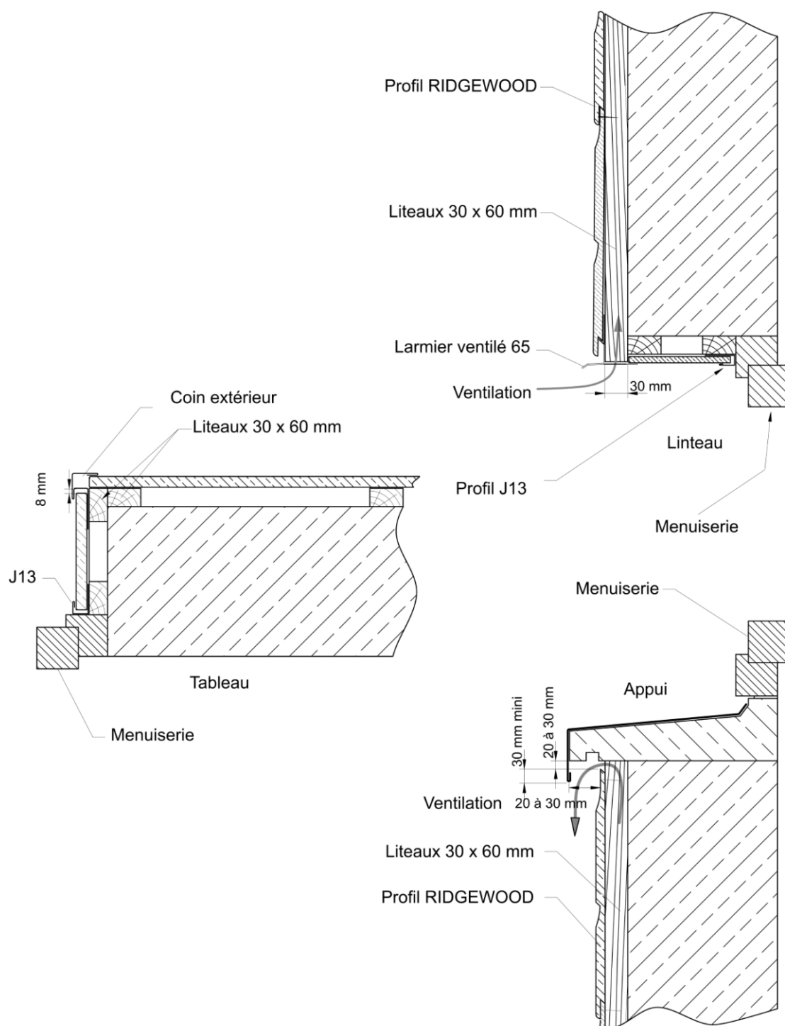
Figure 23 – Coupe sur menuiserie avec tableaux sur maçonnerie
