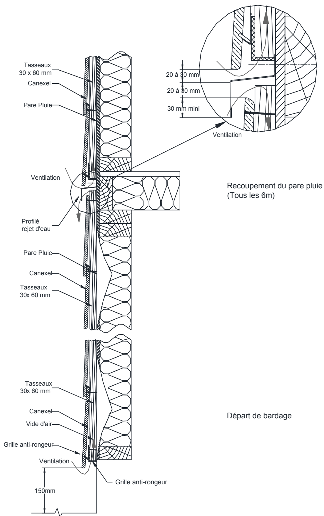
Figure A2 – Fractionnement de l'ossature à chaque plancher sur COB
