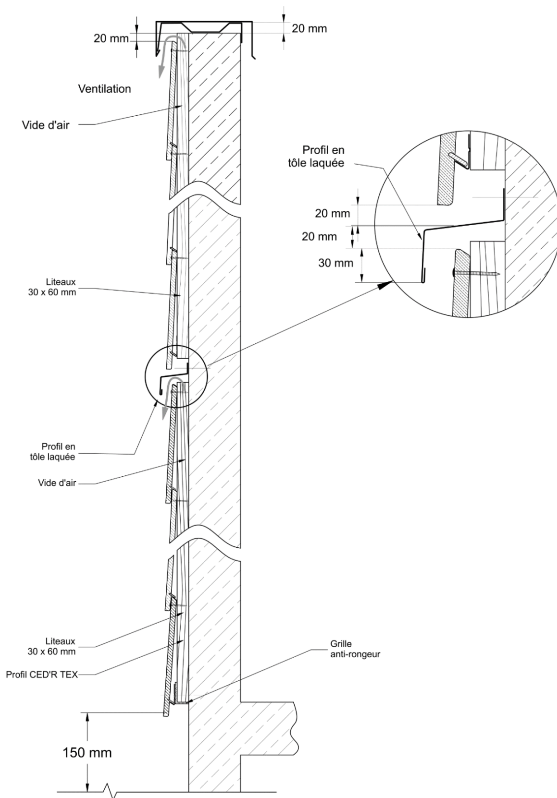
Figure 19 – Détails joint de fractionnement et acrotère (chevrons de longueur = 5,4 m)
