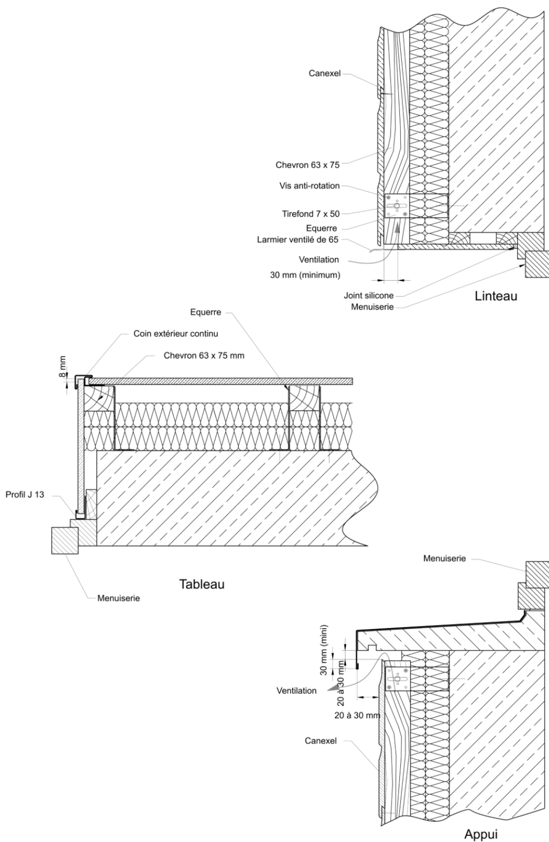
Figure 24 – Coupe sur linteau, tableau et appui Pose sur maçonnerie avec isolant
