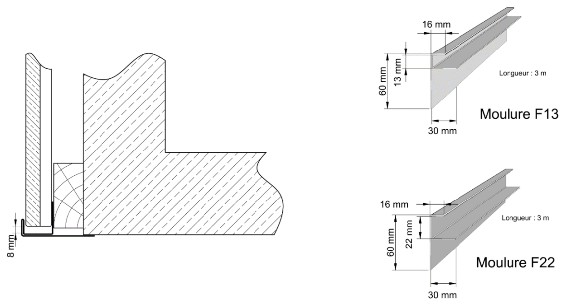
Figure 12 – Arrêt latéral sur revêtement – Moulure F
