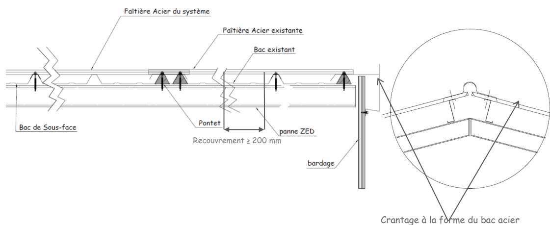
Figure 28 – Mise en œuvre au faîtage en toiture partielle
