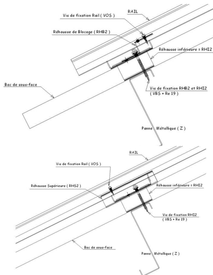
Cas de fixation avec 1 vis VBS et 1 vis VOS
