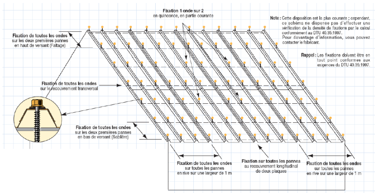
Figure 16 – Principe de répartition des fixations des bacs de sous-face
