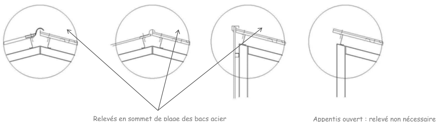
Cas avec Bavette d'étanchéité supérieure « Fibrociment » ou « sous coiffe »
