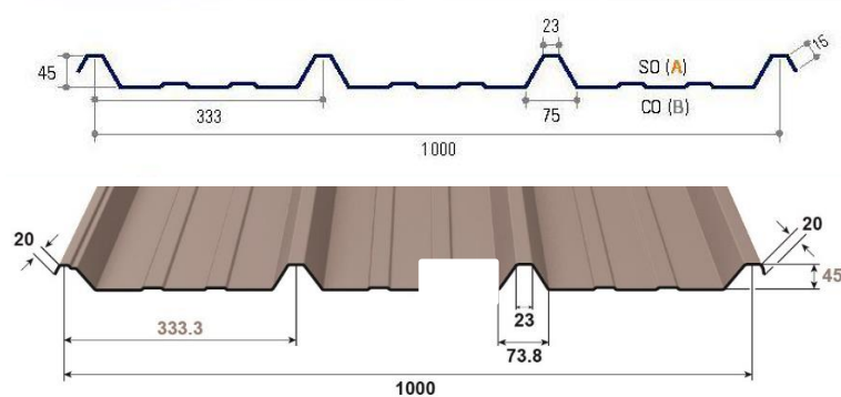
Figure 3 – Bacs de sous-face
