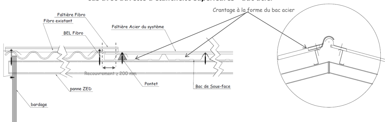
Cas avec Bavette d'étanchéité supérieures «Bac acier»
