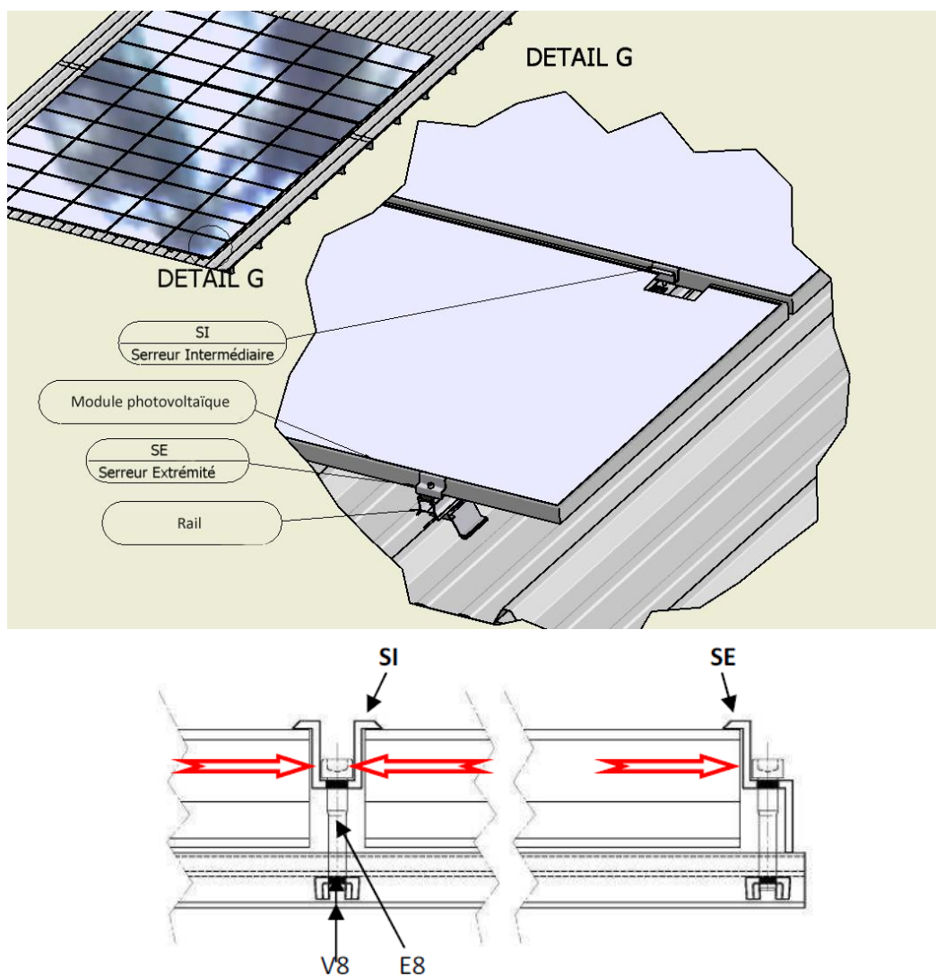
Figure 26 – Mise en place des modules avec les serreurs intermédiaires (SI) ou d'extrémité (SE)
