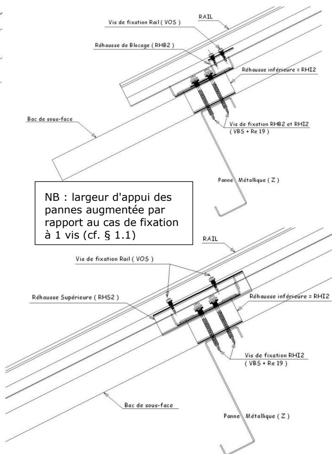
Cas de fixation avec 2 vis VBS et 2 vis VOS
