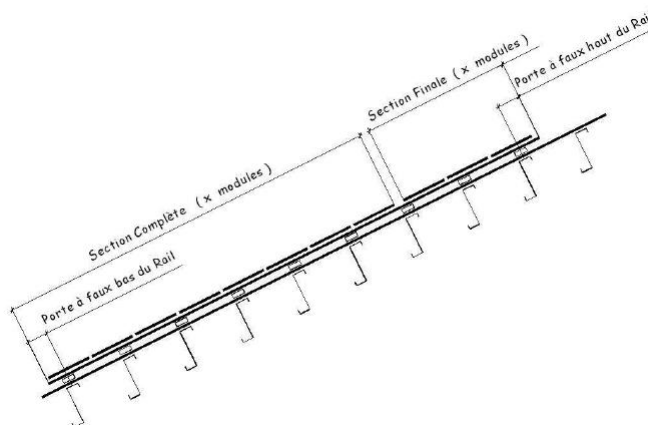
Cas de fixation avec 2 vis VBS et 2 vis VOS
