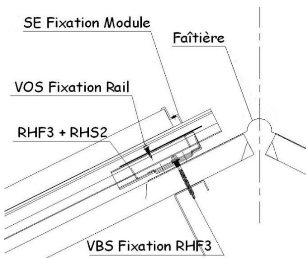
Positionnement des rehausses de faîtière : une seule par colonne de rails
