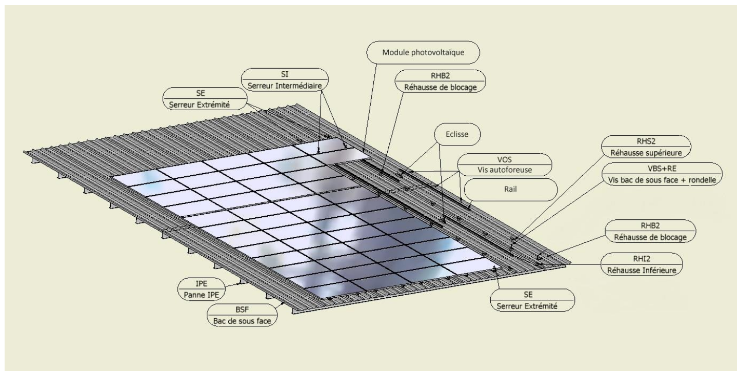
Figure 1 – Schémas éclaté et coupe générale du procédé
