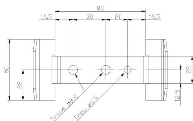
Figure 7 – Rehausse de faitage
