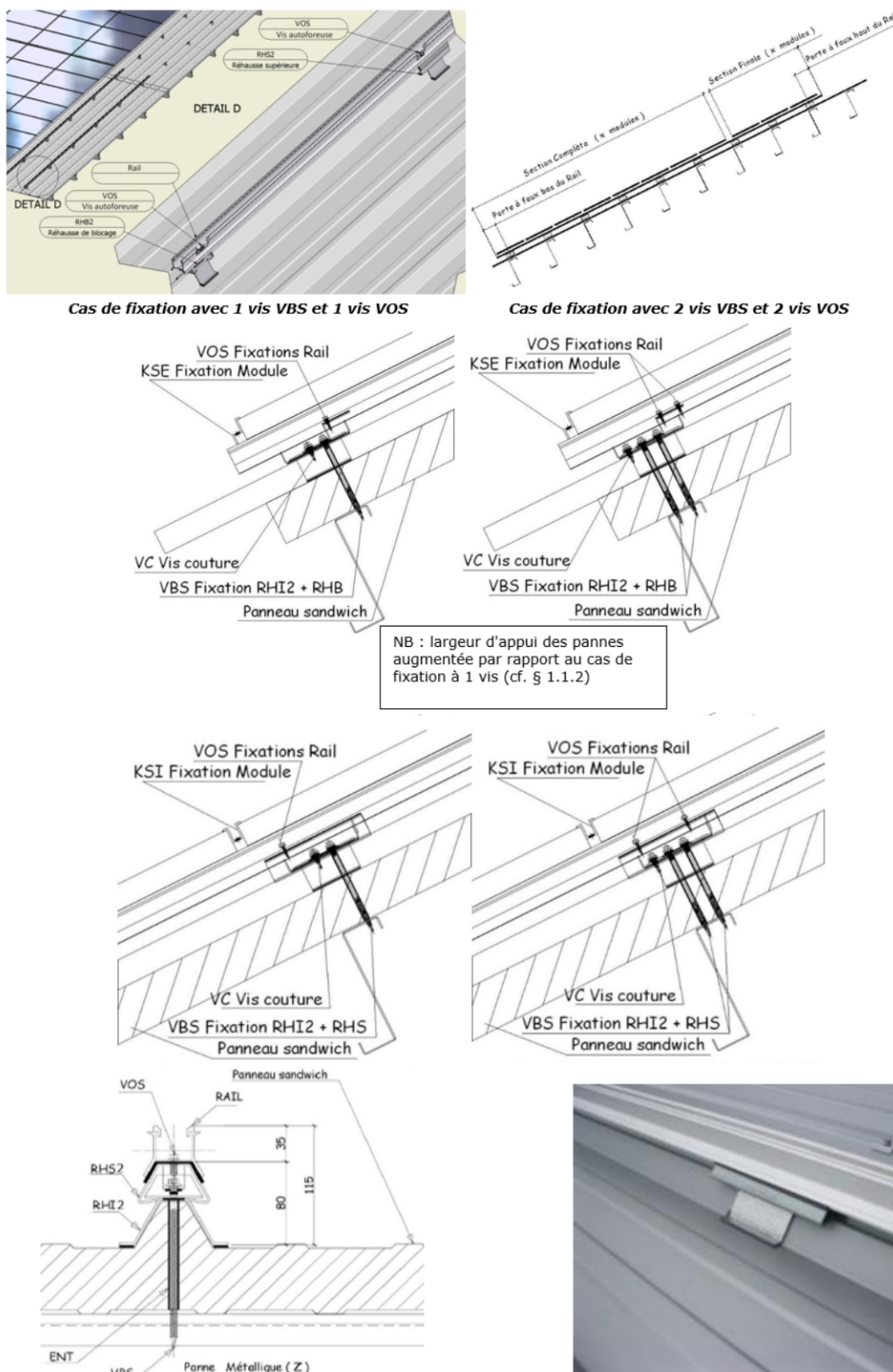
Figure 20 - Fixation du rail sur la rehausse de blocage ou la rehausse supérieure (L'entretoise n'est pas partout représentée sur ces sections)
