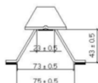
Réhausse Inférieure
