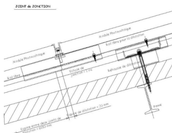
Figure 23 – Éclissage à la jonction de deux rails
