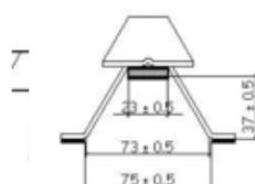
Réhausse Inférieure
