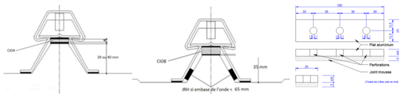
Figure 15 - Mise en place de la cale (L'entretoise n'est pas représentée sur ces sections)
