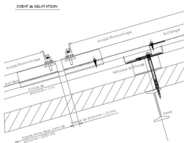
Figure 24 – Éclissage au joint de dilatation (L'entretoise n'est pas représentée sur ces sections)
