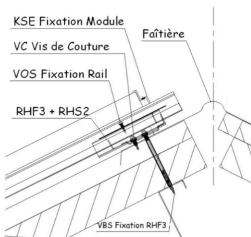
Figure 18 - Illustration de l'utilisation de la rehausse de faîtière (L'entretoise n'est pas représentée sur ces sections)
