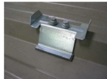
Figure 16 - Illustration de la fixation du perçage des panneaux sandwich et de la pose de l'entretoise (Cas simple vis ; pour le cas double vis cf. Figure 20)
