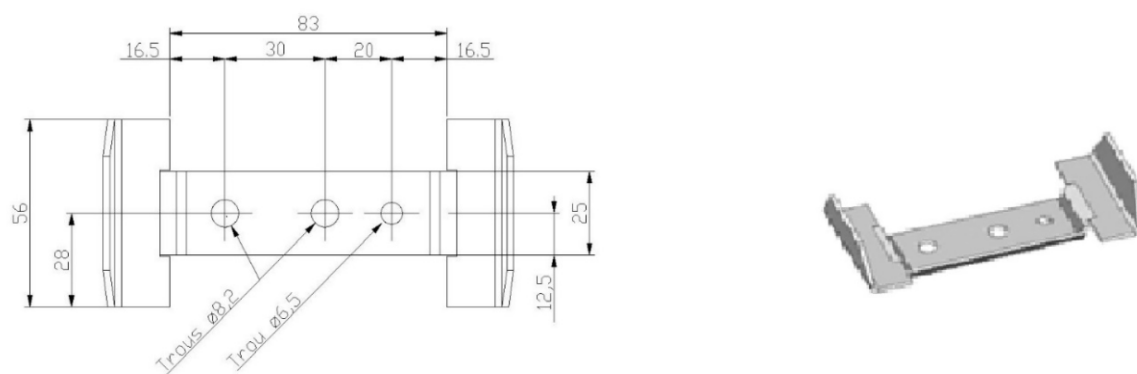
Figure 6 – Rehausse de faitage
