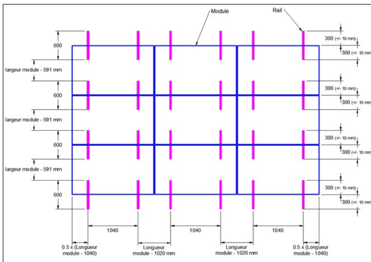
Figure 35 - Implantation des rails / modules à plat
