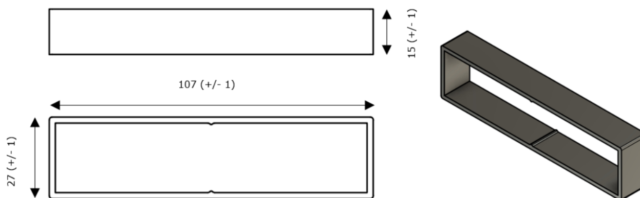
Figure 20 - Cale rotule du kit d'inclinaison du procédé ROOF-SOLAR BITUME TAN DTU – Plat & Incliné
