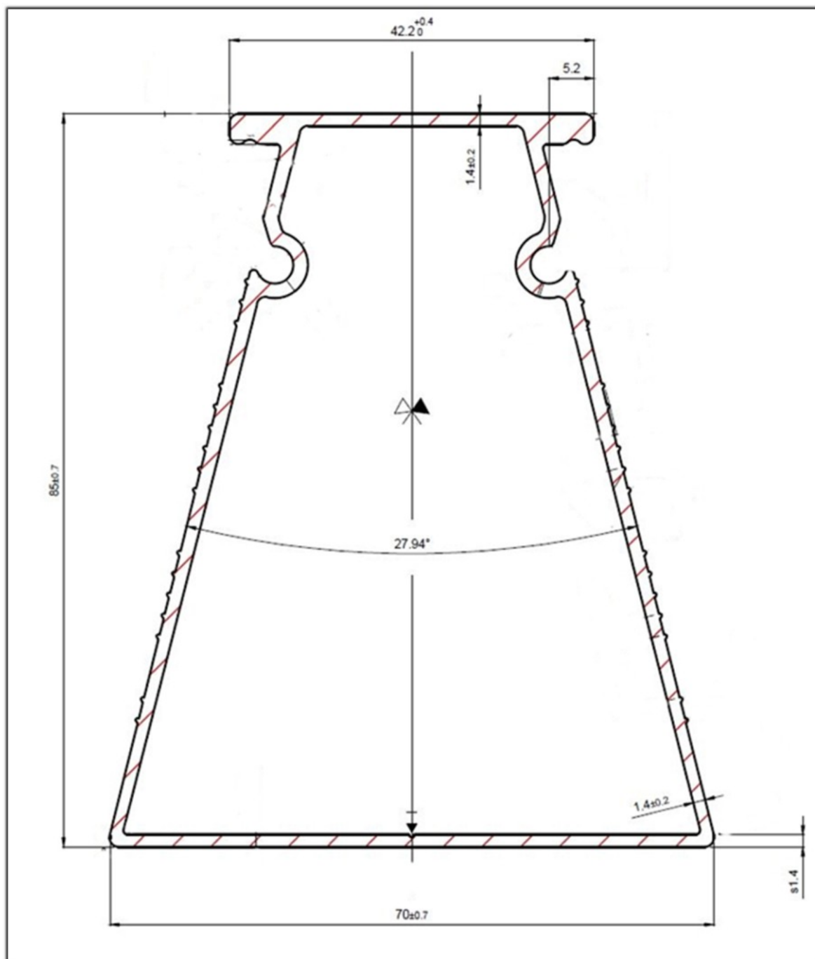
Figure 6 – Profil trapézoïdal
