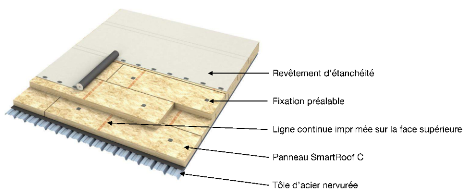
Figure 21 - Sens de pose des panneaux SmartRoof C
