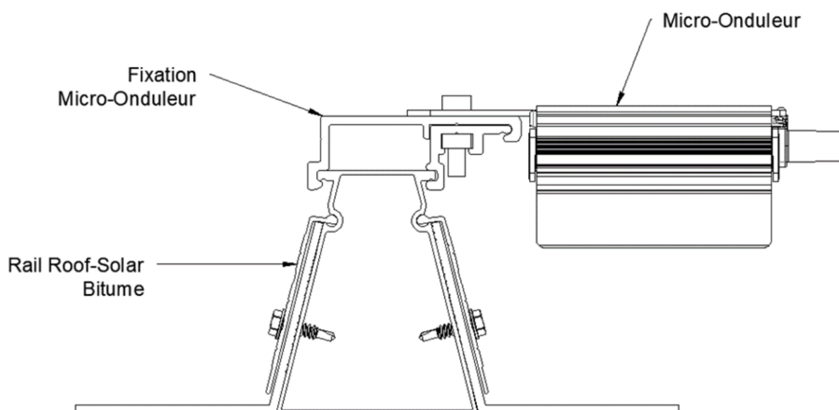
Figure 26 - Micro-onduleurs
