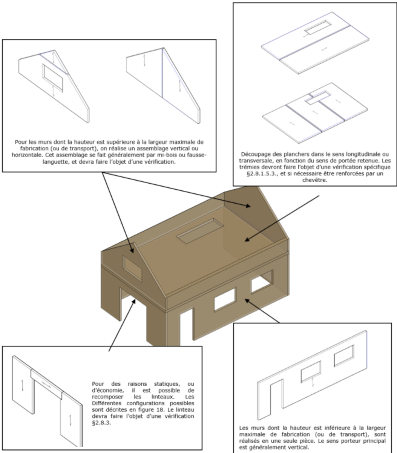
Figure 11 : exemple de calepinage à partir de panneaux PFEIFER CLT
