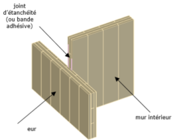
Figure 14: assemblage de panneaux muraux en angle
