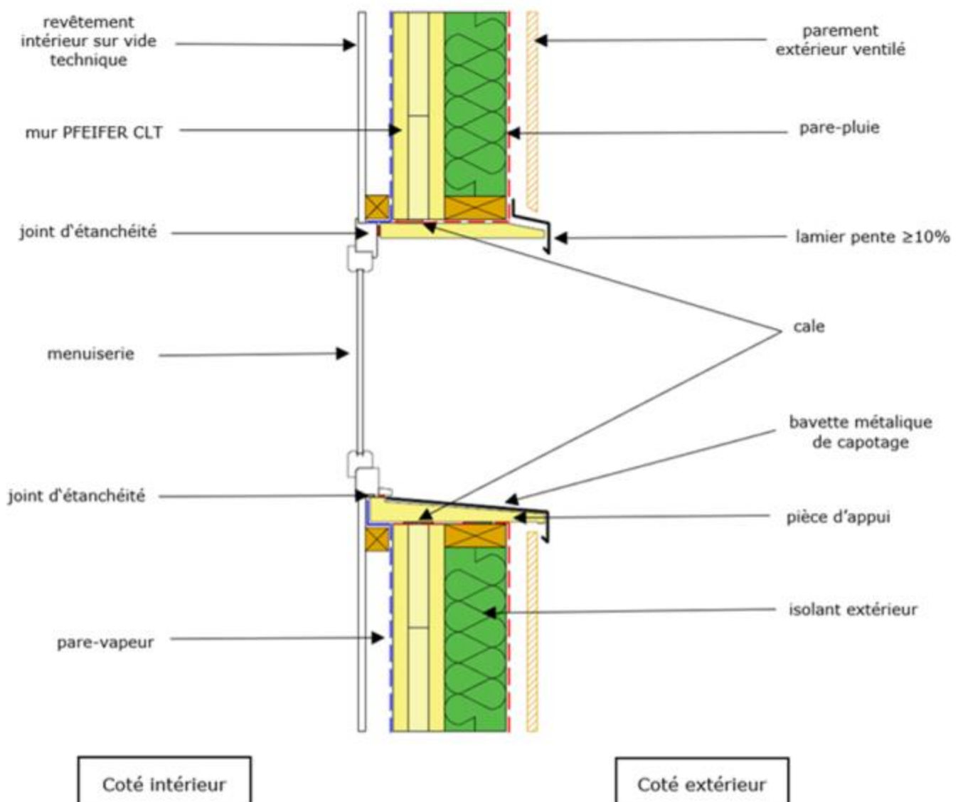
Figure 23: exemple d'intégration de menuiserie extérieure
