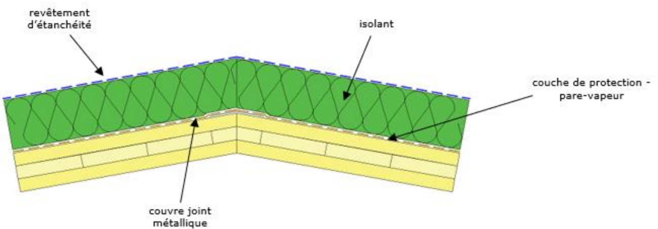
Figure A.13b – Exemple de jointement au faitage non appuyé
