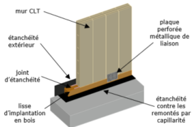
Détail 4 : fixation par plaque perforée sur lisse d'implantation
