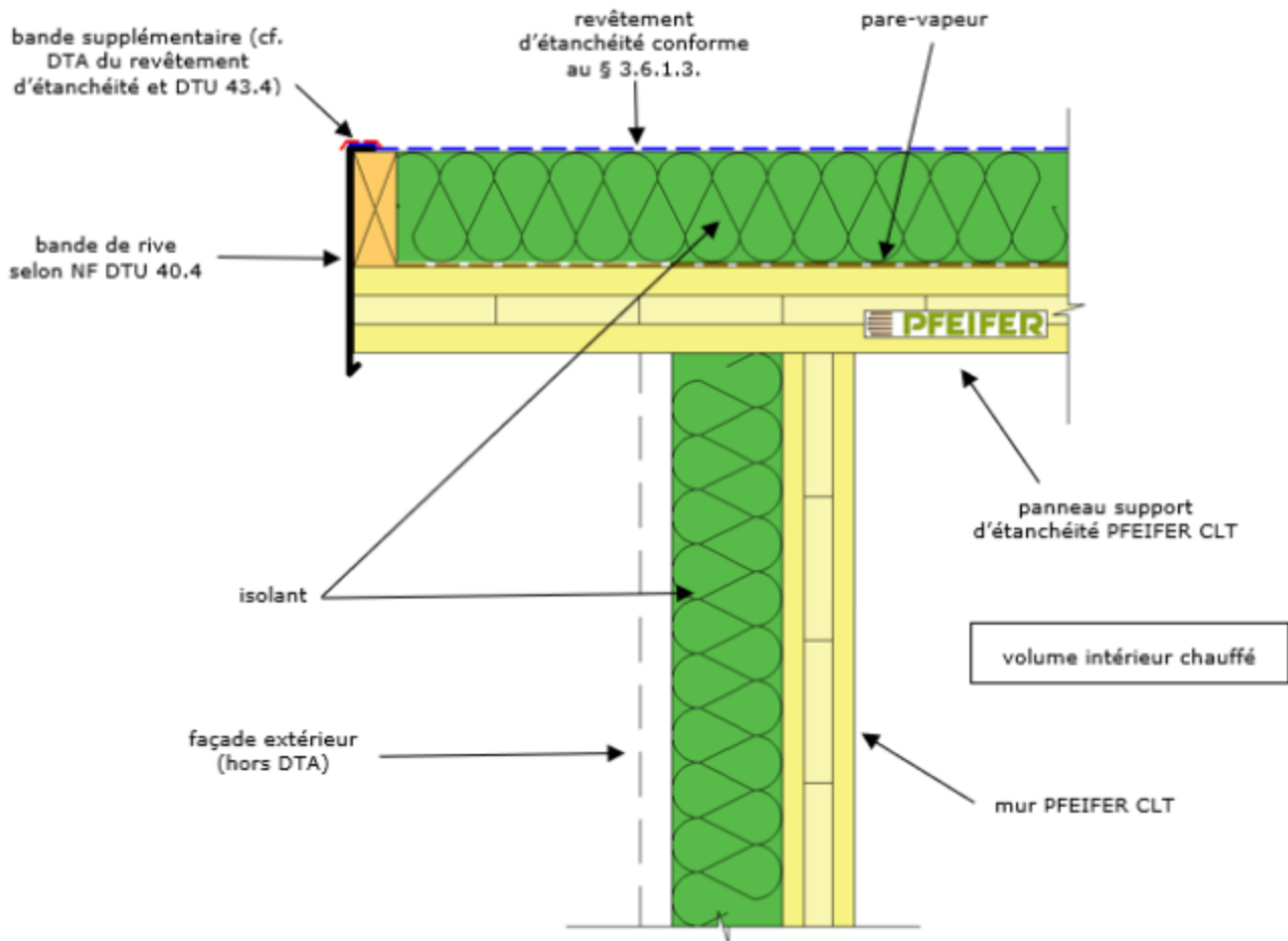
Figure A.7c – Costière de rive selon le NF DTU 43.4 P1 - Bâtiment chauffé avec toiture isolée
