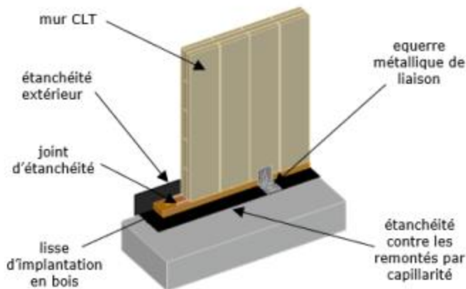
Détail 5 : fixation par équerre haute sur talonnette béton
