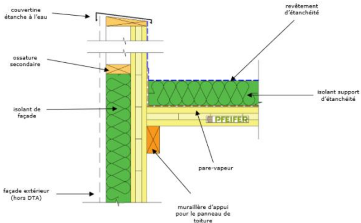
Figure A.8b – Exemple de relevé sur panneau PFEIFER CLT avec costière métallique (selon NF DTU 43.4. P1) en toitures inaccessible, technique ou végétalisée
