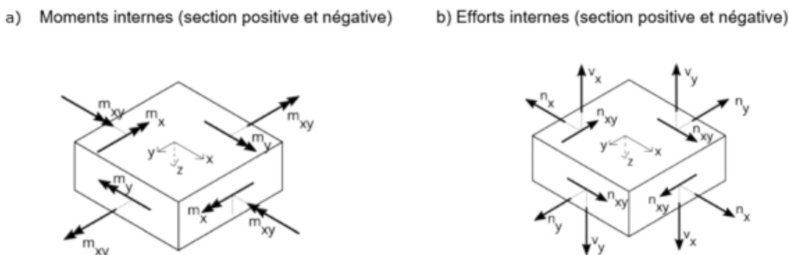
Figure 7 - sollicitations internes des sections opposées
