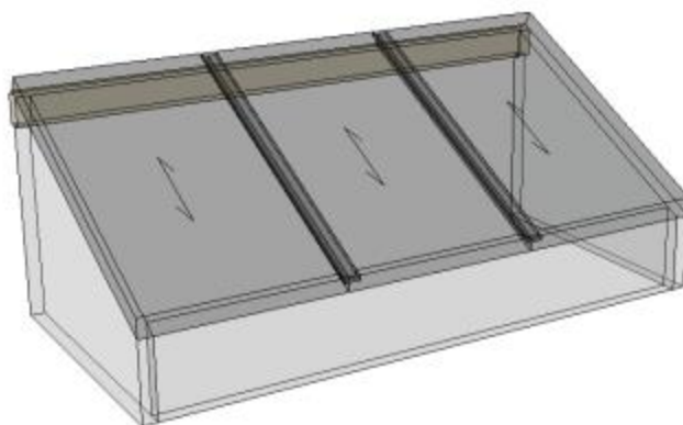
Figure A.14b – Pose dite « lambourde » avec sens de portée des panneaux parallèle au faitage
