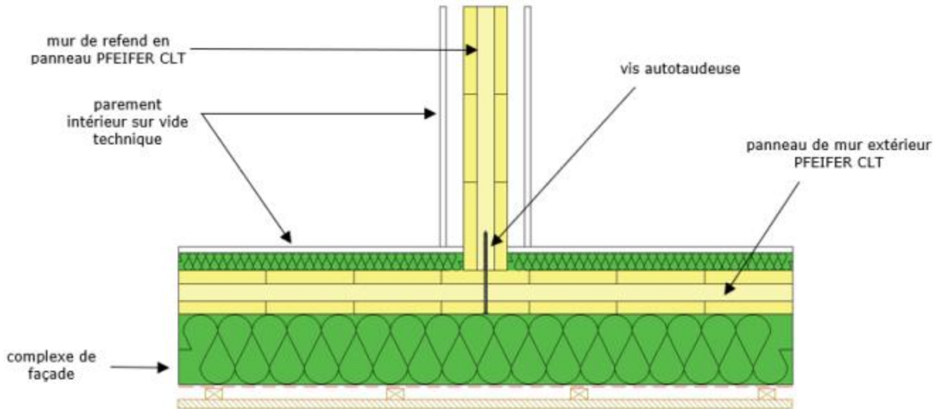
Figure 15: exemples de liaisons entre un mur extérieur et refend intérieur (vue en plan)
