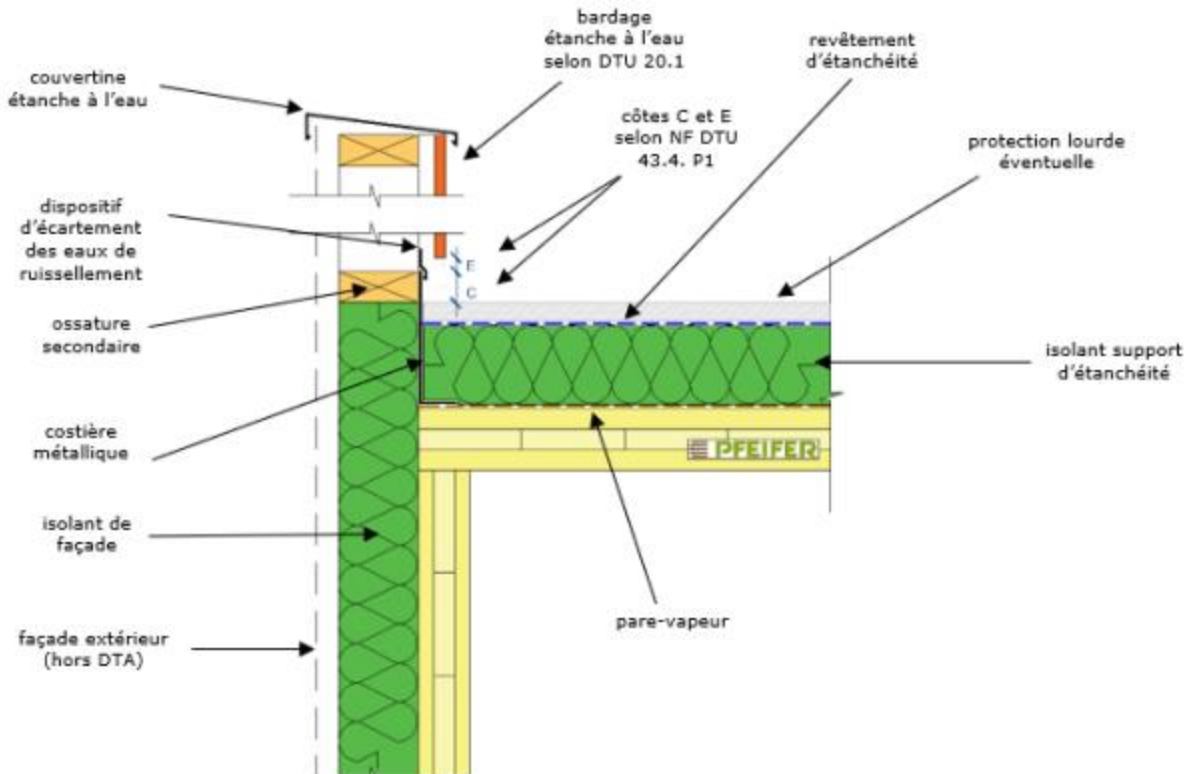
Figure A.8b – Exemple de relevé sur panneau PFEIFER CLT avec costière métallique (selon NF DTU 43.4. P1) en toitures inaccessible, technique ou végétalisée
