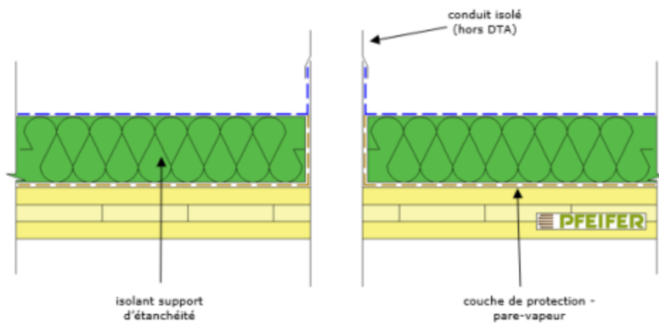
Figure A.11 – Traversée ponctuelle
