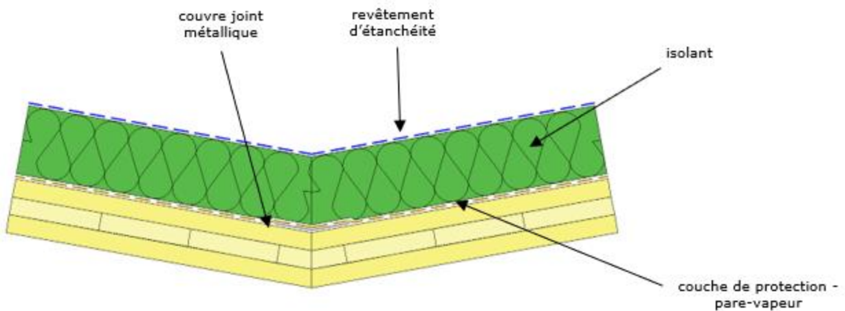
Figure A.13a – Exemple de jointement au faitage sur appui simple
