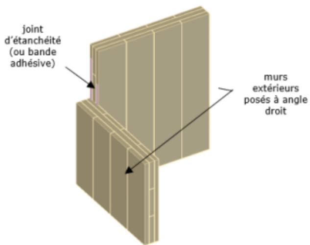
Figure 14: assemblage de panneaux muraux en angle
