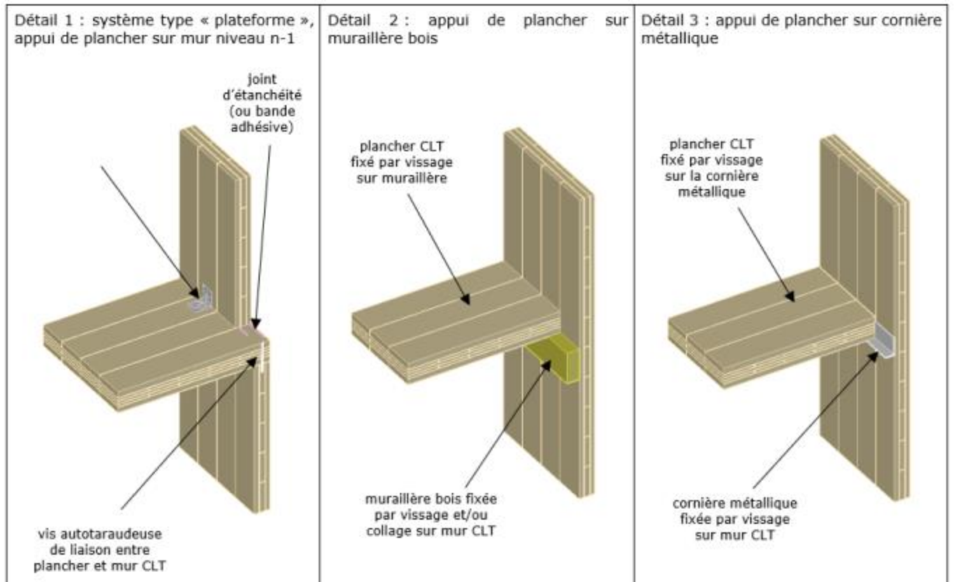
Figure 16: exemples de liaisons entre panneau de mur et plancher intermédiaire CLT
