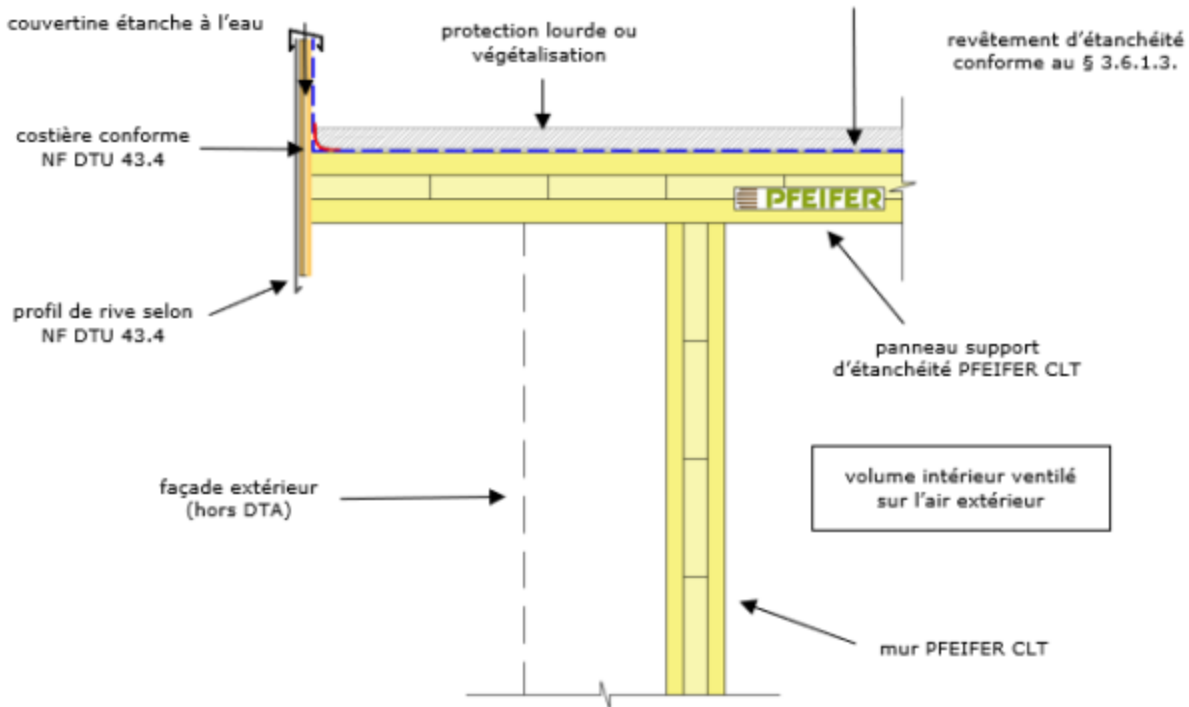
Figure A.7b – Bande de rive métallique – Bâtiment chauffé avec toiture isolée
