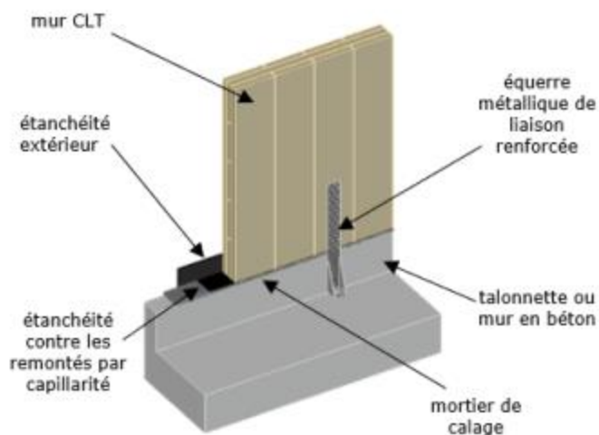
Détail 5 : fixation par équerre haute sur talonnette béton
