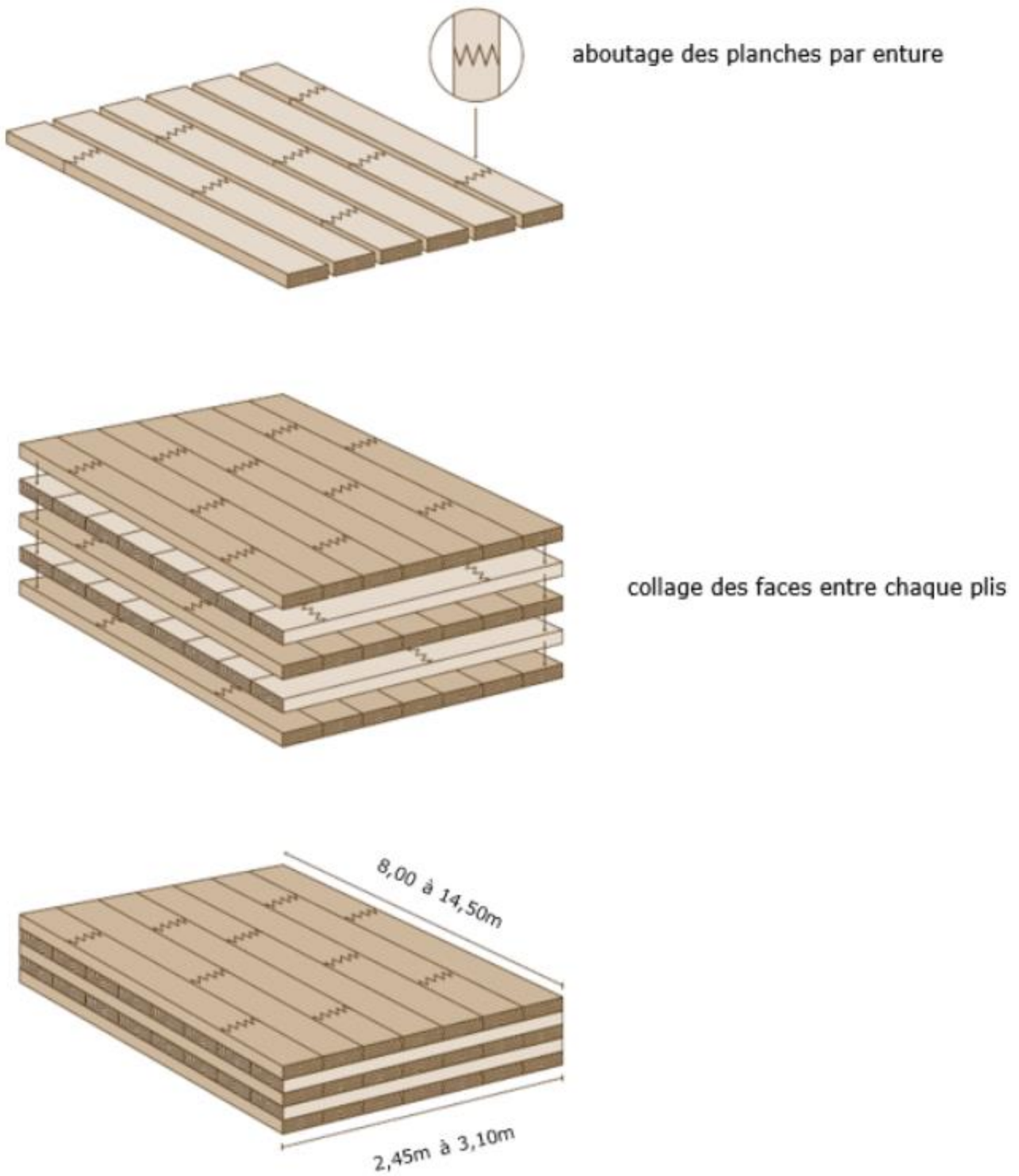
Figure A.5 – Exemple de composition des panneaux PFEIFER CLT
