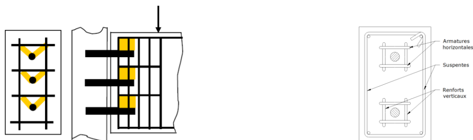
Figure 1 : Exemple de disposition des armatures de l'about de poutre
