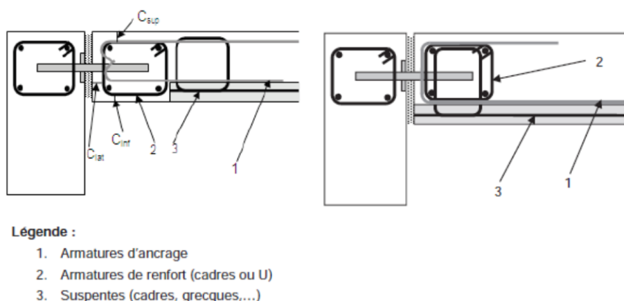
Figure 3 : Exemples de ferrailages dans le cas d'appuis sur goujons (prédalles BA à gauche et prédalle BA ou BP à droite), le goujon est à mi-hauteur ( H/2 ) de la hauteur totale de la dalle et de calcul H
