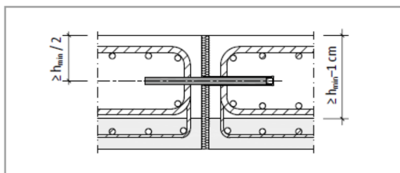
Figure 5 : Dalle avec prédalle - Hauteur h_{min} (épaisseur minimale d'une dalle coulée en place de la dalle de compression).
