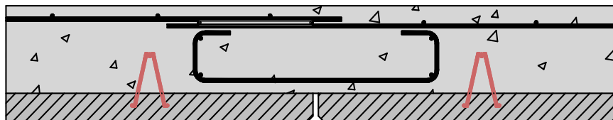
FIGURE 24 Liaison droite (couturée)
