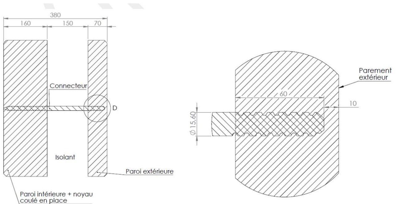
Figure 4 : Vue en coupe du connecteur composite en fibres de verre AR
