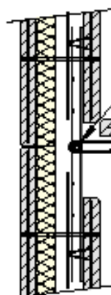
Liaison verticale avec refends
