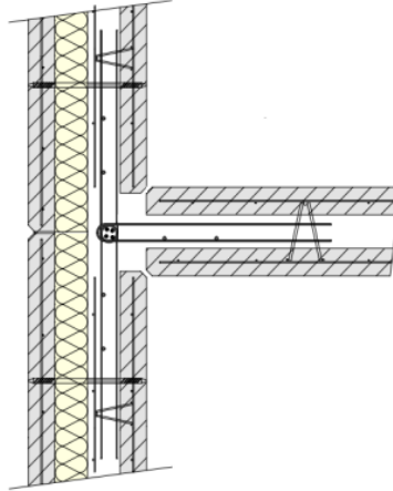
Schéma 8 - Coupe de principe d'une liaison paroi / refend
