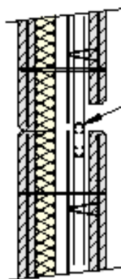
Liaison verticale (variante)
