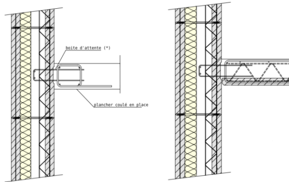
Schéma 4 - Coupes de principes de liaison paroi/dalle avec prédalle suspendue (non adaptée au sismique) ou dalle coulée en place
