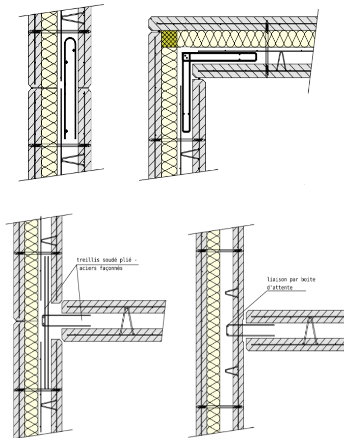
Schéma 7 - Coupes de principes des joints verticaux rotulés
