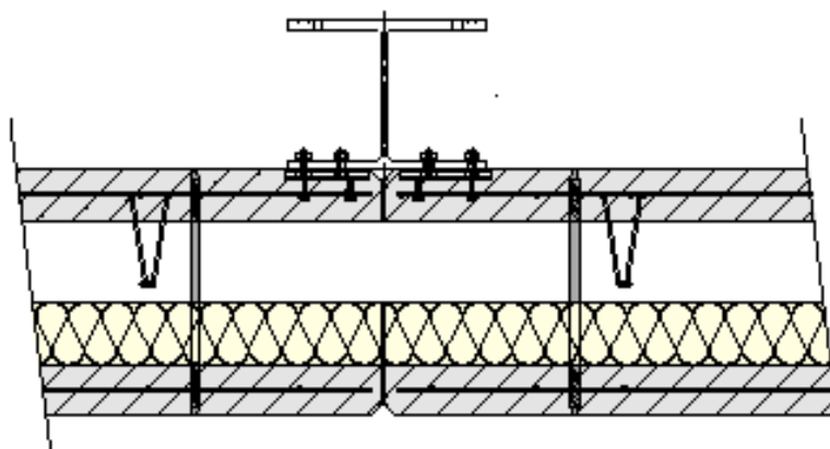
COUPE A-A
