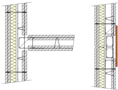
Schéma 5 - Coupes de principes des joints verticaux encastrés
