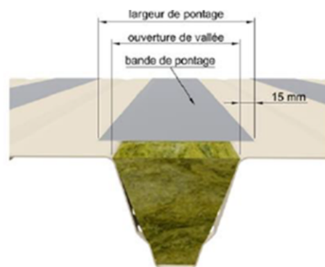
Positionnement de la bande de pontage
