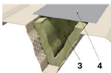
Schéma avec matelas souple en laine de verre 3 feutre acoustique 4 bande de pontage
