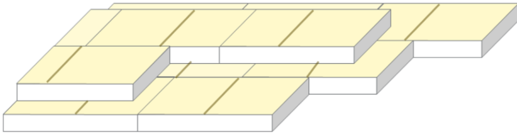
Figure 4 – Pose en quinconce des panneaux ALPHATOIT - ALPHATOIT 36 en deux lits avec joints décalés
