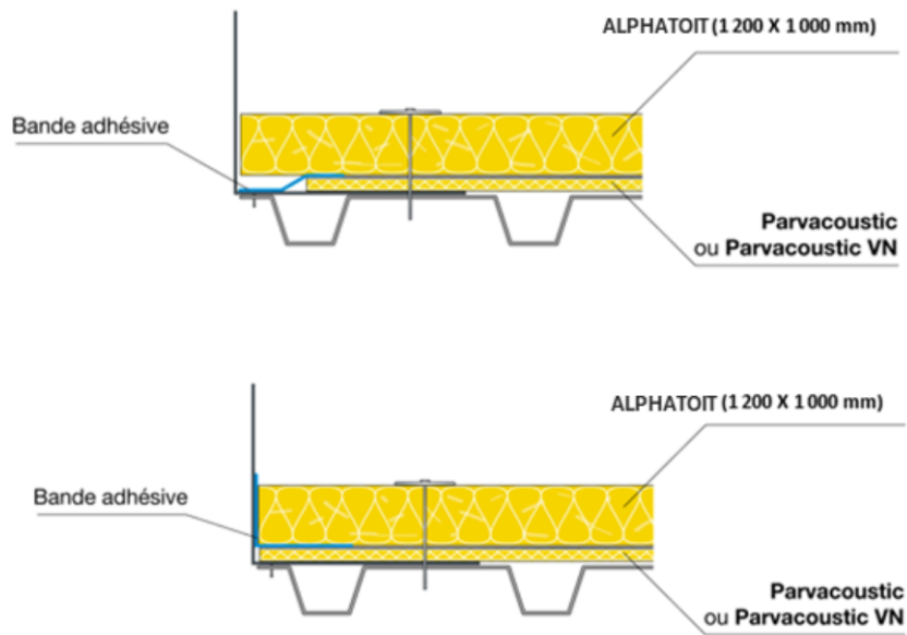
Figure 9 – Principe du traitement en rive du pare-vapeur PARVACOUSTIC
