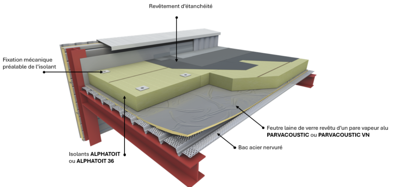
Figure 6 – Principe de mise en œuvre en système ALPHATOIT ou ALPHATOIT 36/PARVACOUSTIC 4 fixations mécaniques préalables par panneaux
