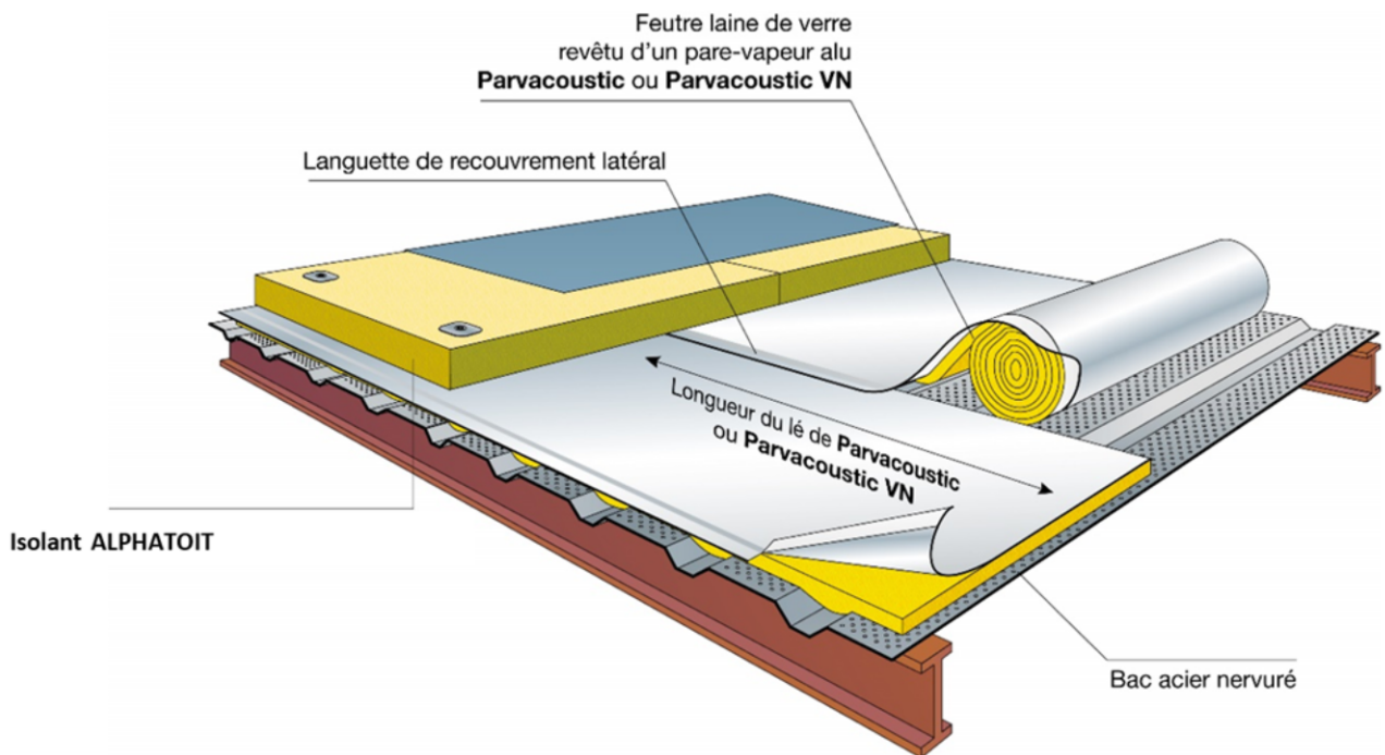
Figure 8 – Principe de déroulage du pare-vapeur PARVACOUSTIC
