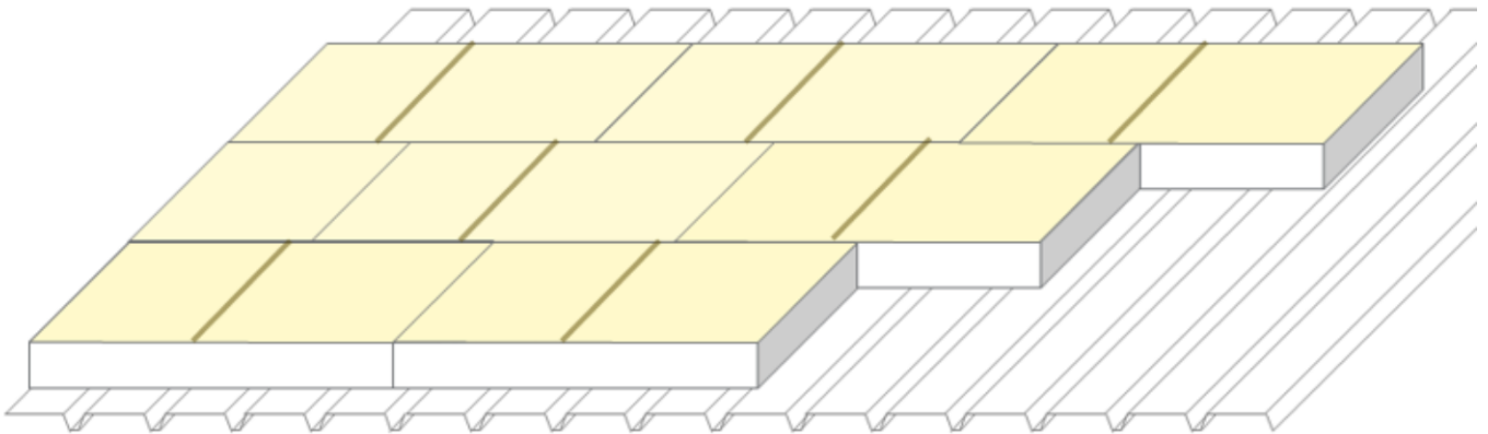
Figure 5 – Pose des panneaux ALPHATOIT et ALPHATOIT 36 avec la ligne de marquage parallèle aux nervures des TAN conformes au NF DTU 43.3 ou conformes aux Cahier du CSTB 3537 de janvier 2009 ((Ohn) > 70 mm et \leq 200 mm pour l'ALPHATOIT 36 uniquement).
