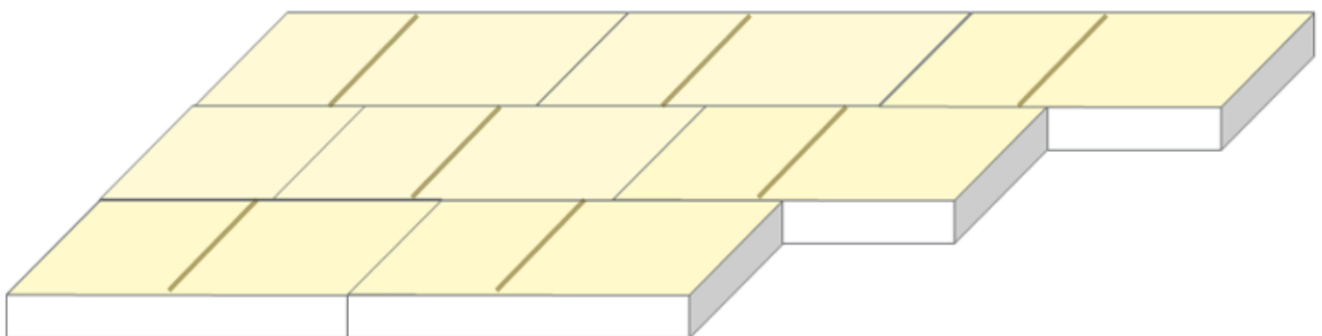
Figure 3 – Pose en quinconce des panneaux ALPHATOIT - ALPHATOIT 36
