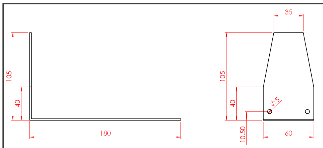
ZEA 4040 : Equerre pour de retenue pour Connect 25 et Connect 40 avec connecteur renforcé
