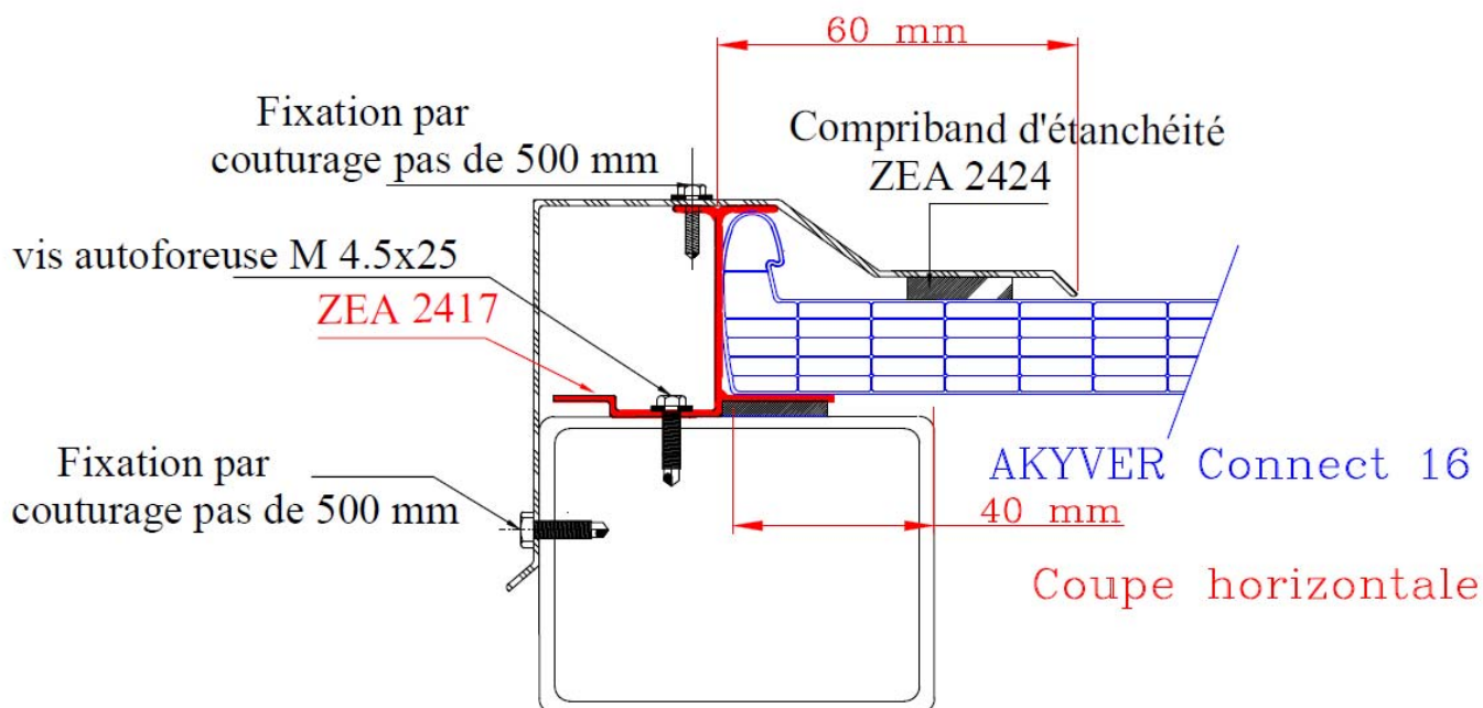
Figure 19 – Détail de rive avec crochet
