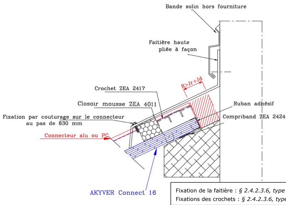
Figure 19 – Détail de rive avec crochet
