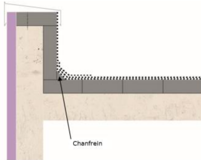
Figure 6 – Exemple de traitement d'acrotère sur élément porteur béton avec chanfrein
