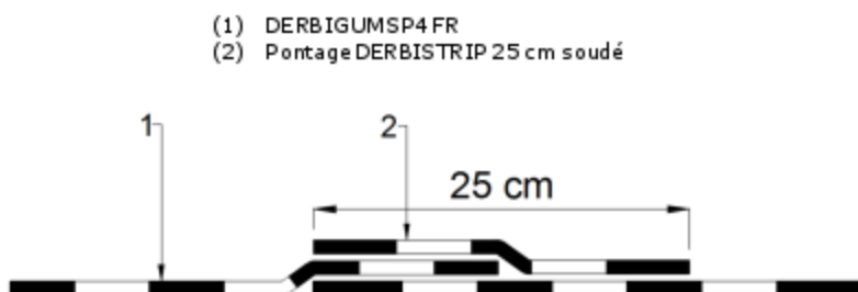
Figure 7 - Pontage des recouvrements, en pente nulle sur maçonnerie
