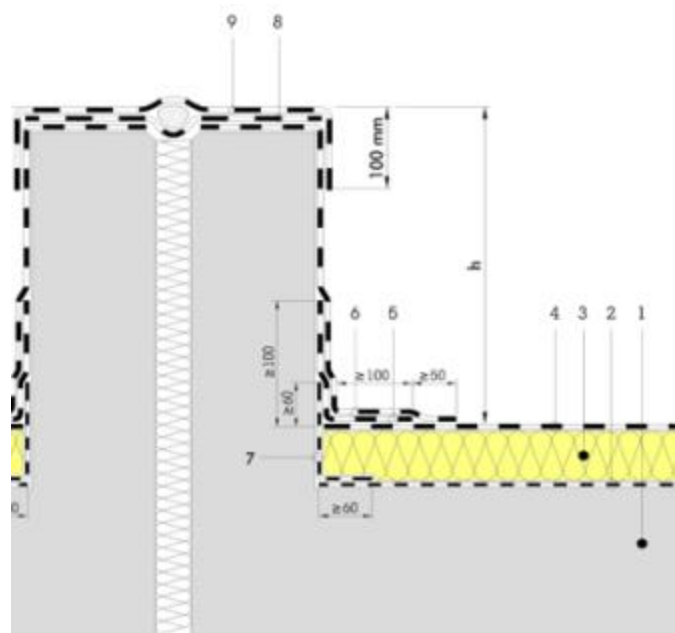
Figure 3 – Exemple d'entrée d'eaux pluviales
