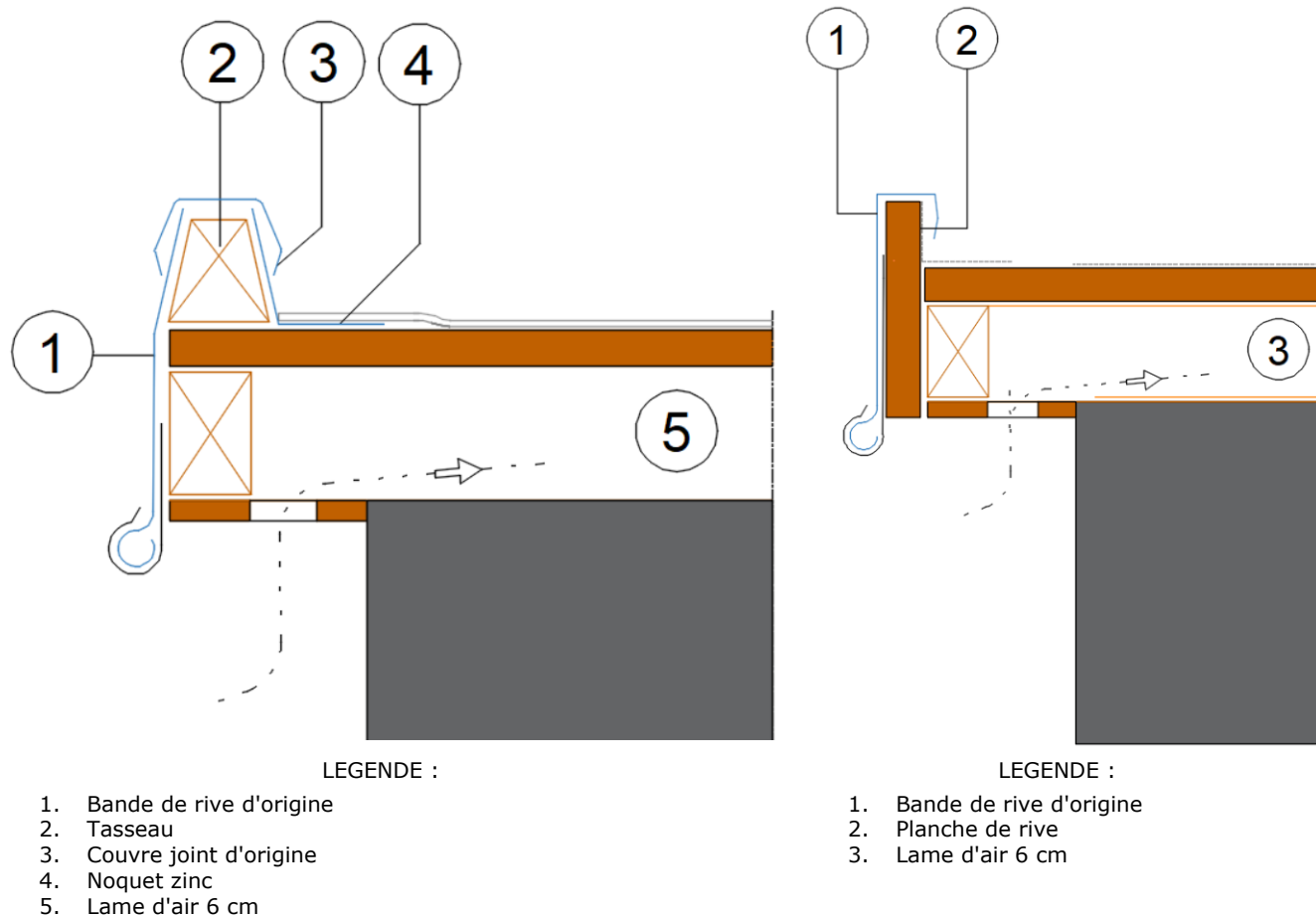
Figure 29 – Rive avec relevé latéral, couverture d'origine
