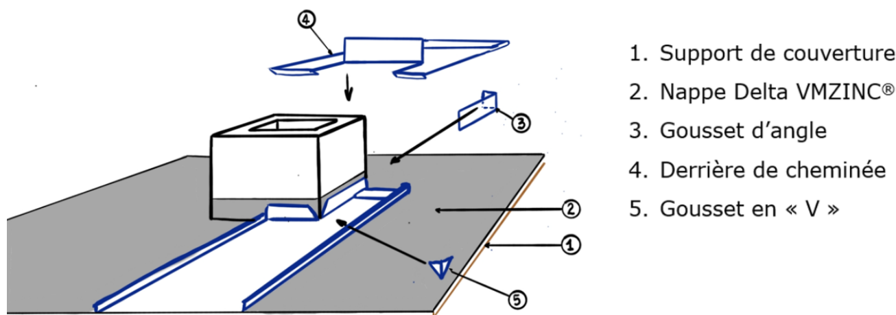
Figure 23 – Exemple de pénétration sur plusieurs bacs
