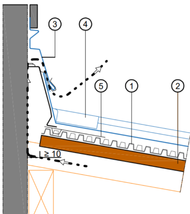
Figure 13 - Faîtage mono-pente ventilé
