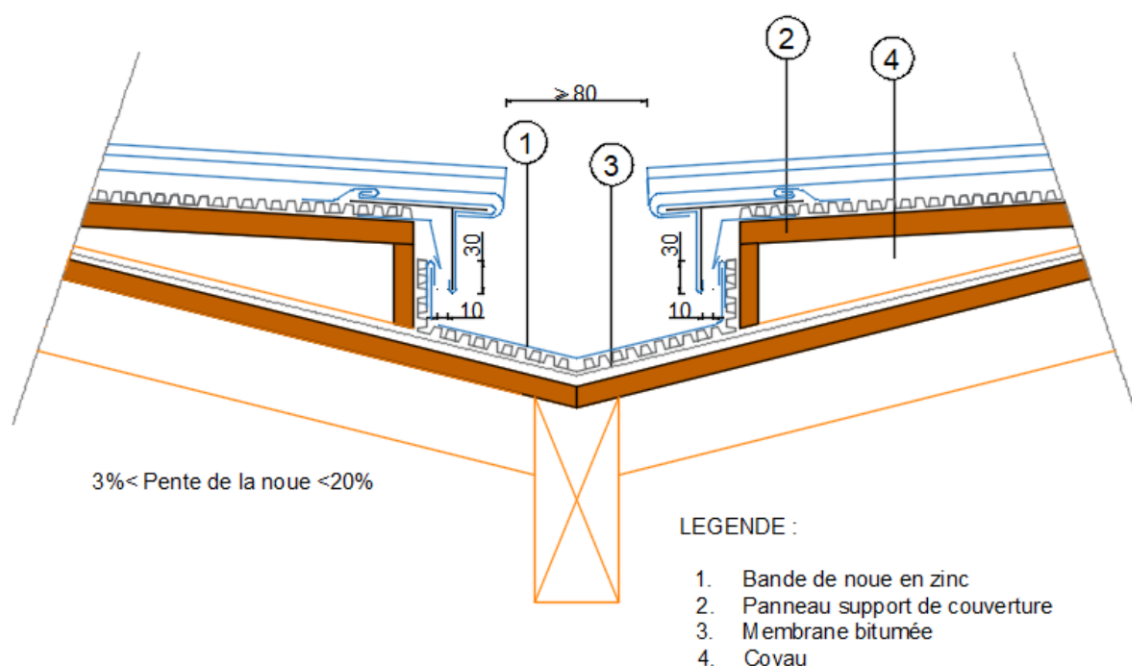
Figure 34 – Noue encaissée avec coyau
