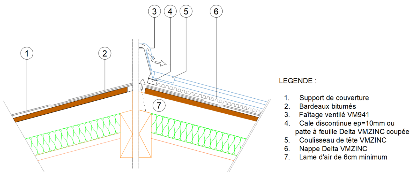
Figure 27 – Faîtage ventilé
