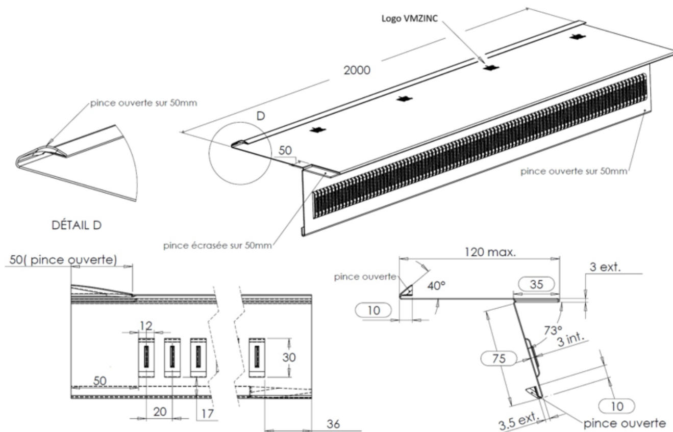
Figure 6 – Kit d'égout ventilé
