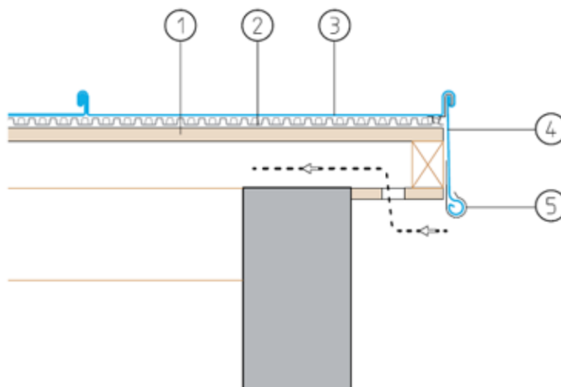
Figure 18 - Rives façonnées sans planche de rive
