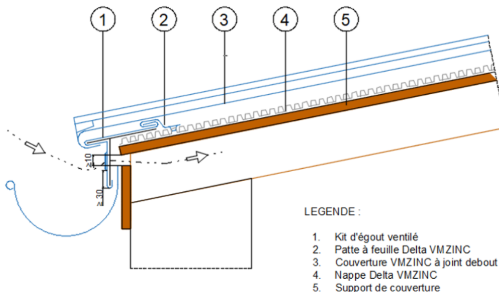
Figure 10 – Egout avec gouttière pendante
