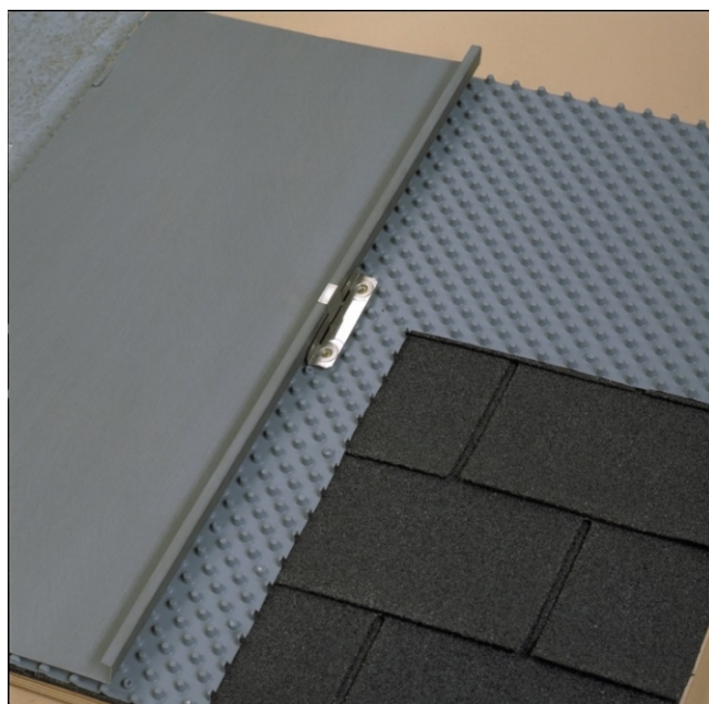
Figure 2– Représentation du système Delta VMZINC® sur bardeaux bitumés
