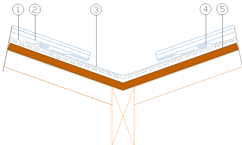
Figure 19 – Noue avec pente > 20%
