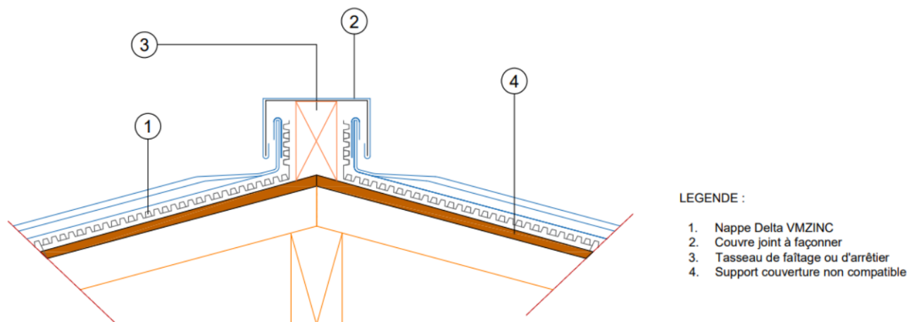
Figure 16 – Faîtage non ventilé, arêtier
