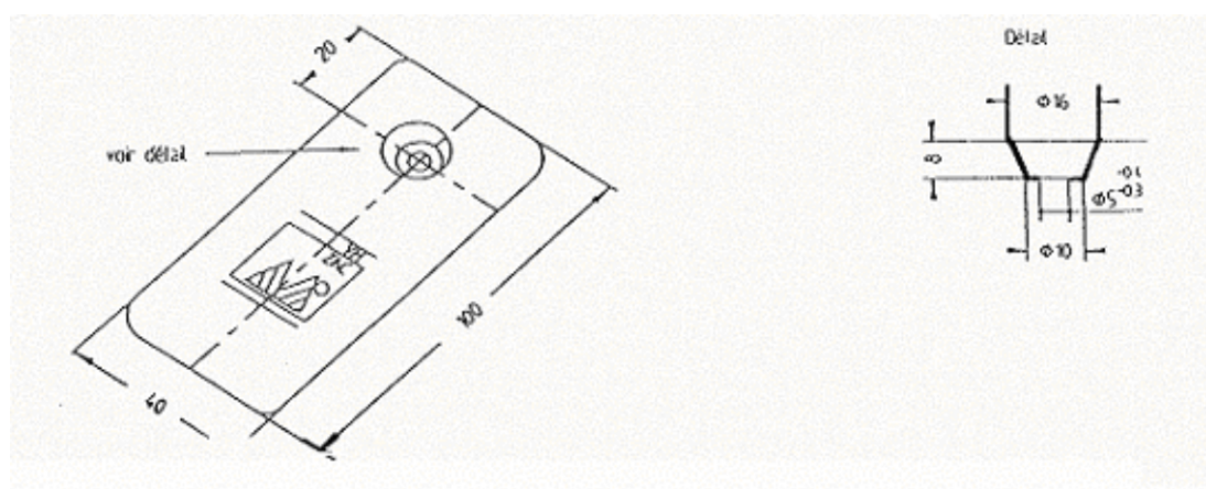
Figure 5 – Patte à feuille Delta VMZINC®
