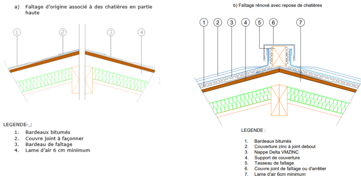
Figure 26 – Faîtages non ventilés
