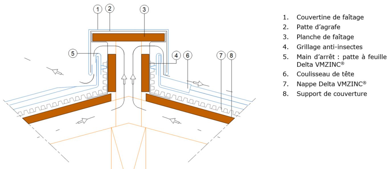
Figure 14 – Faîtage traditionnel
