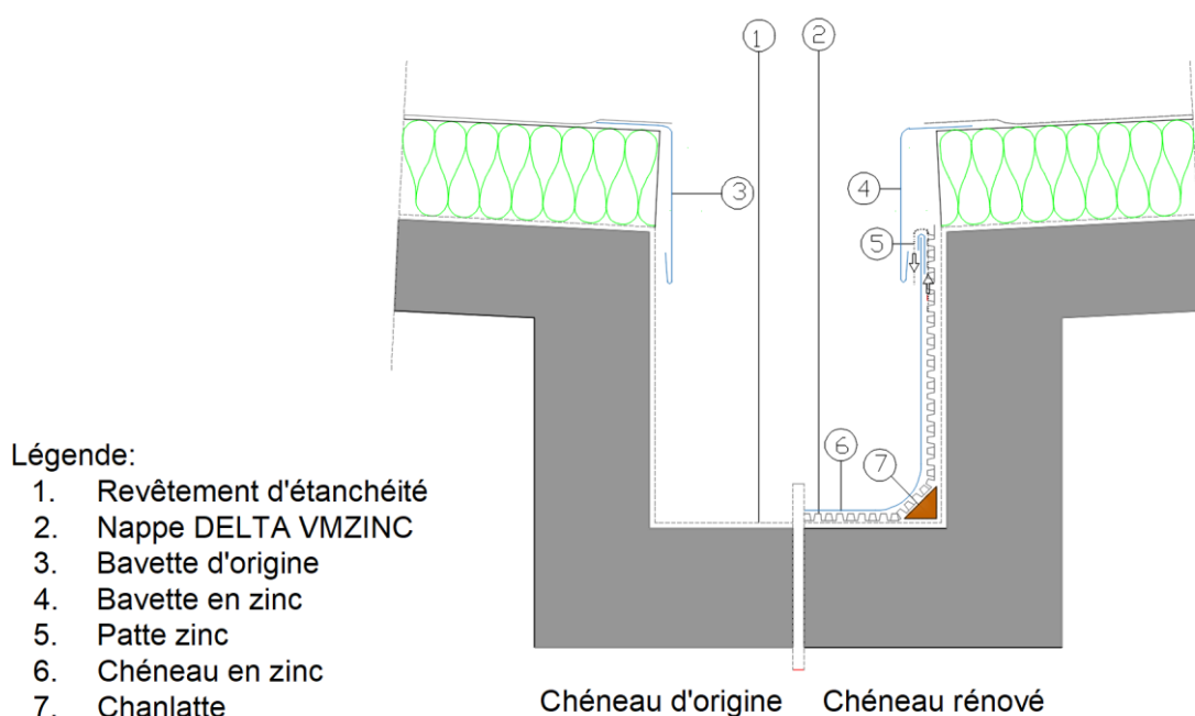
Figure 36 – Chéneau étanchéité sur béton
