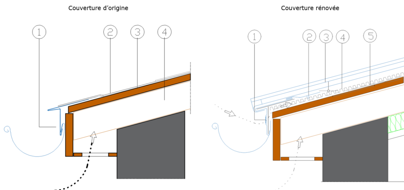
Figure 24 – Egout, couverture en réfection sur bardeaux bitumés
