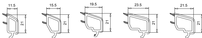
107 215 Parclose
