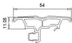
109 682 Battue extérieure Bouchon 109 686
