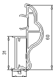
109 533.3 Moulure 60mm pour aile de 13mm
