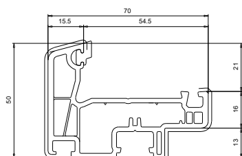
103 368 Battement Monobloc 50 mm
