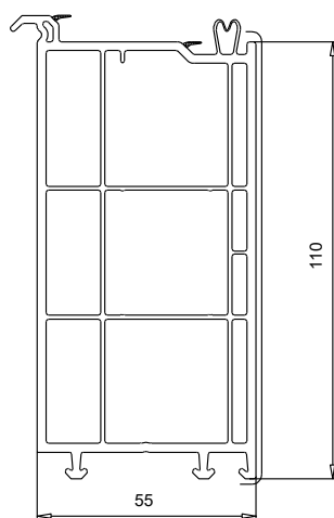
109 121 Elargisseur 110 mm
