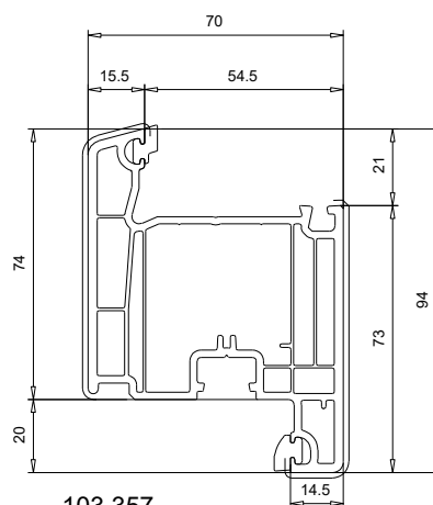
103 357 Ouvrant 94 mm
