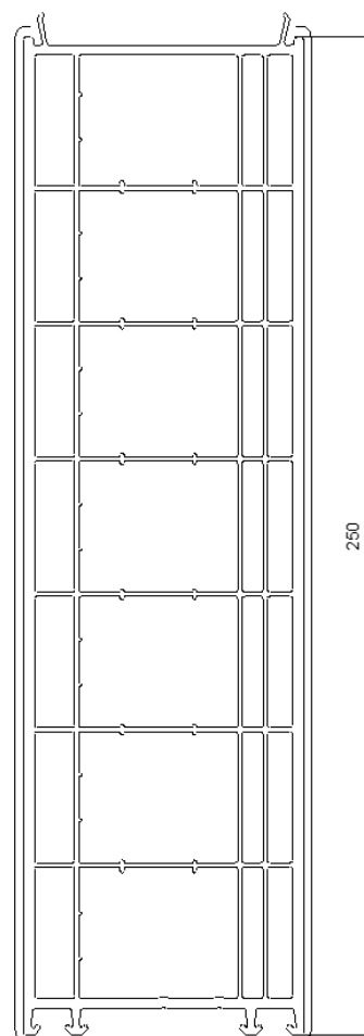
114 205 Elargisseur 250 mm
