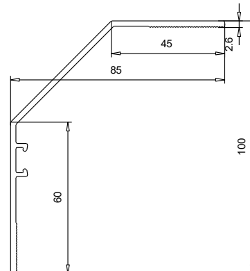
109 373 Cornière
