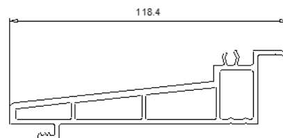
110 063 Pièce d'appui 105.5 mm
