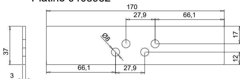
Lisse filante 3mm ACIER INOX
