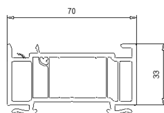
114 035 Elargisseur 33 mm
