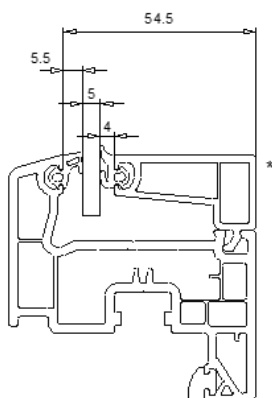
volume mini avec joint spécifique 112053
