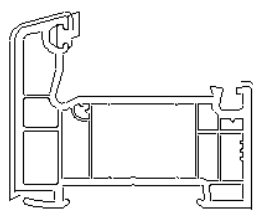
101 249 Dormant 57 mm
