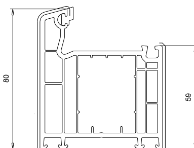
101 214 Dormant 80 mm
