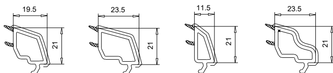
107 128 Parclose
