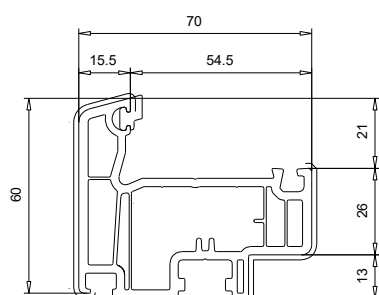
103 293 Battement Monobloc 60 mm
