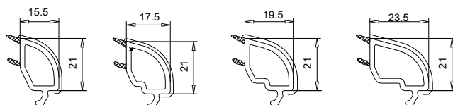
107 238 Parclose
