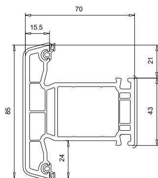
102 218 Traverse / Meneau 85 mm
