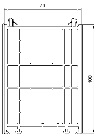
114 203 Elargisseur 100 mm
