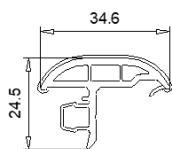
109 654 Battue extérieure Bouchon 109 687
