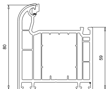
101 235 Dormant 80 mm
