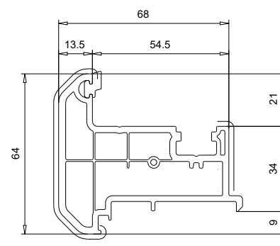
102 236 Battement rapporté 64 mm Bouchon 109 508
