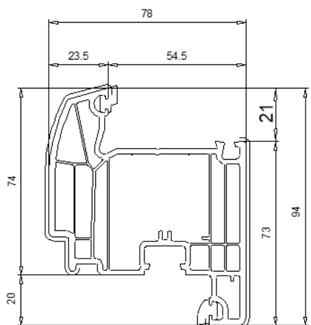
103 333 Ouvrant 94 mm
