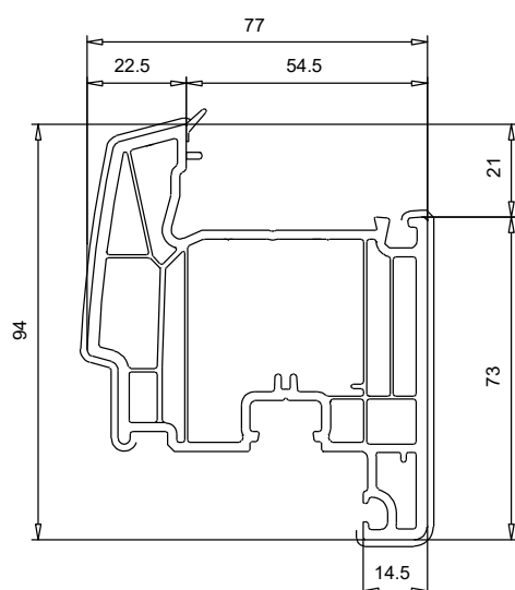
103 337 Ouvrant Serrure 94 mm
