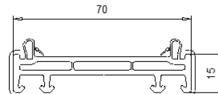
114 200.2 Elargisseur 15 mm
