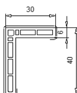
109 070 Cornière
