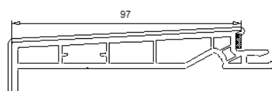
110 092 Pièce d'appui 97 mm
