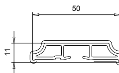
109 627 Battue 50 mm Bouchon 109 625
