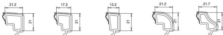
107 190 Vitrage 28mm
