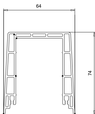
114 031 Profil d'appoint
