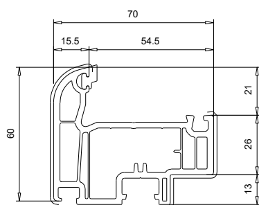
103 295 Battement Monobloc 60 mm
