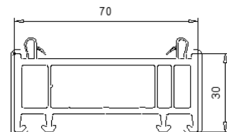
114 201 Elargisseur 30 mm
