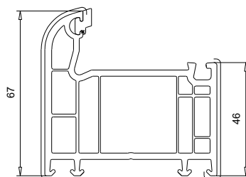
101 233 Dormant 67 mm
