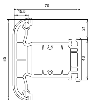
102 233 Traverse / Meneau 85 mm
