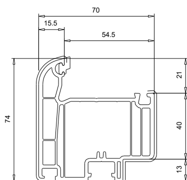
103 288 Battement Monobloc 74 mm
