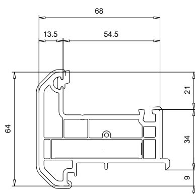
102 215 Battement rapporté 64 mm Bouchon 109 520
