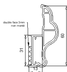
109 533.4 Moulure 60mm pour aile de 13mm
