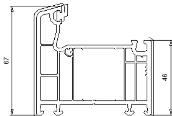
101 266 Dormant 67 mm
