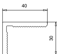
111 007 Cornière
