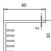
111 021 Cornière
