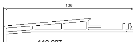
110 007 Pièce d'appui 90 mm
