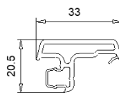
109 031 Battue extérieure Bouchon 109 032
