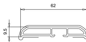
109 499 Battue 62 mm Bouchon 109 500
