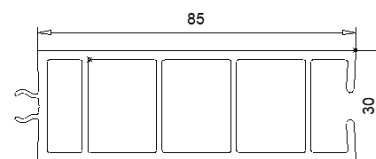
109 210 Tapée 30 mm
