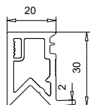
109 272 Tapée 20 mm
