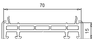
114 200 Elargisseur 15 mm
