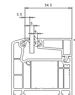
volume mini avec joint spécifique 112053
