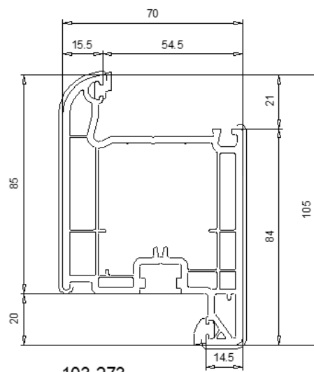
103 273 Ouvrant Serrure 105 mm
