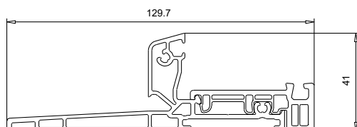
104 455 Seuil mixte aluminium - PVC 1.0
