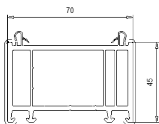
114 202 Elargisseur 45 mm
