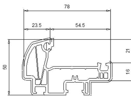
103 334 Battement monobloc 50 mm
