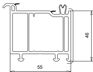
109 126 Elargisseur 46 mm
