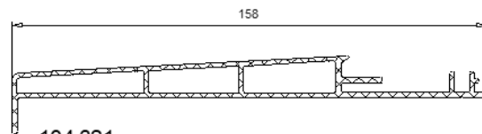
104 321 Pièce d'appui alu 112 mm
