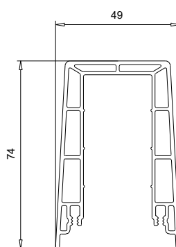
114 051 Profil d'appoint
