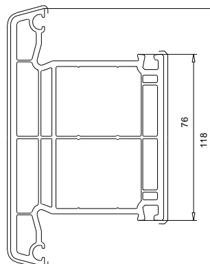
102 238 Traverse / Meneau
