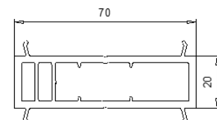
116 201 Epine - Elargisseur 20mm
