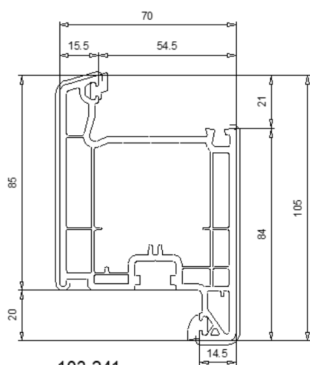
103 241 Ouvrant Serrure 105 mm
