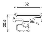
109 031.9 Battue extérieure Bouchon 109 032
