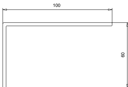
109 002 Cornière
