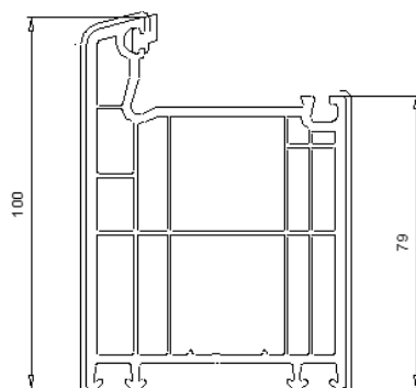
101 215 Dormant 100 mm
