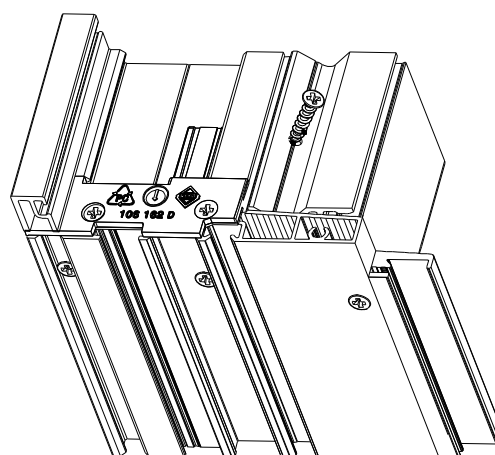
Délignage à la pose : détail en face inférieure
