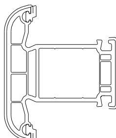
102 235 Traverse / Meneau 85 mm
