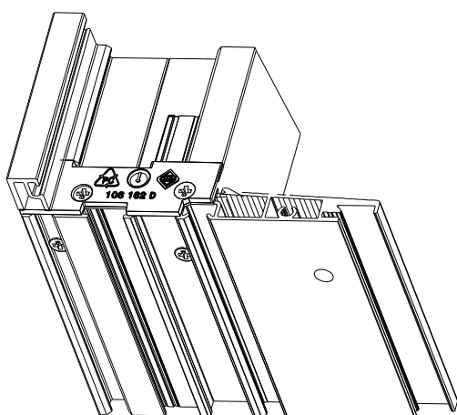
3-Vissages du dormant
