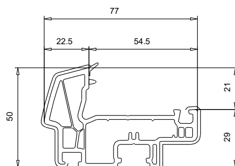
103 338 Battement monobloc fenêtre
