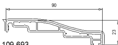
109 693 Moulure 90 mm
