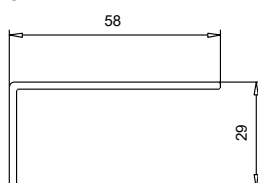
109 013 Cornière
