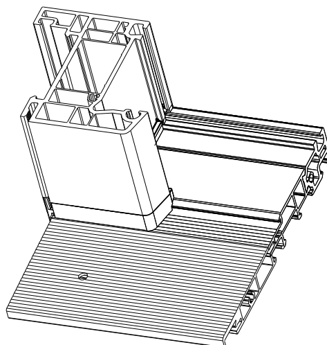
2-Montage embout et dormant
