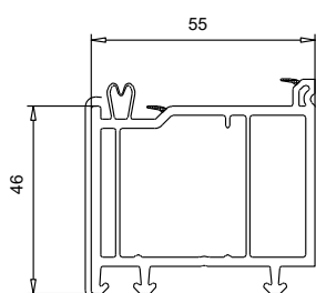
109 126.2 Elargisseur 46 mm
