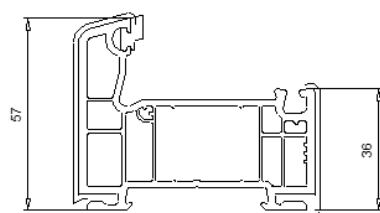
101 247 Dormant 57 mm
