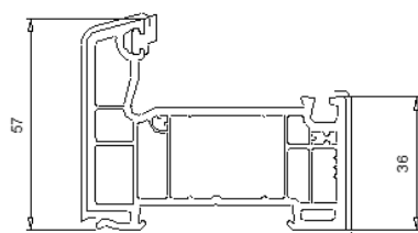
101 256 Dormant 57 mm
