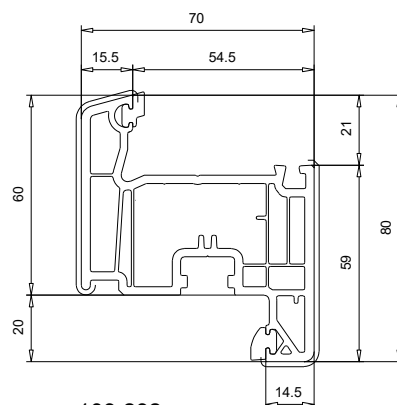
103 232 Ouvrant 80 mm
