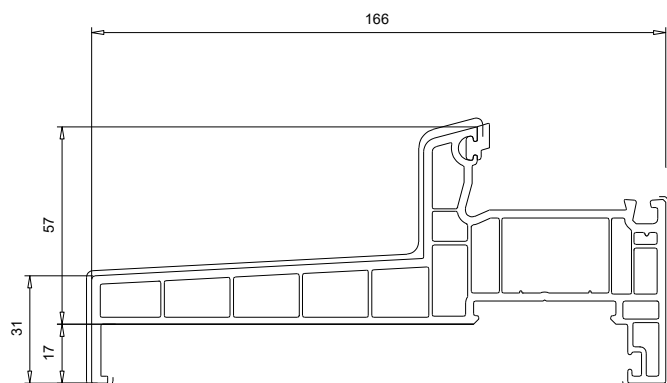
101 244 Dormant 74 x 166 mm (Iso 160)
