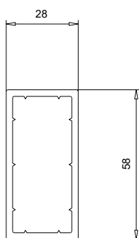
109 082 Profil d'appoint
