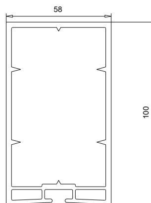
114 003 Profil d'appoint
