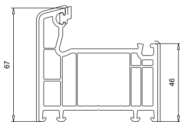
101 246 Dormant 67 mm
