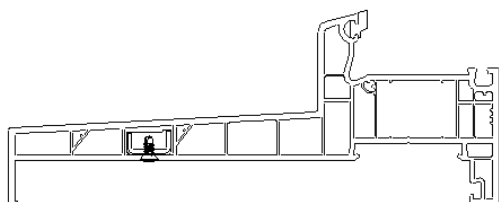
Mise en oeuvre renfort 113 430
