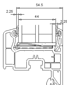
volume maxi avec joint spécifique 112376
