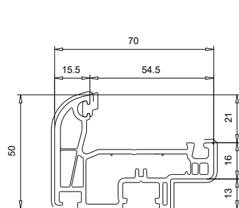
103 369 Battement Monobloc 50 mm
