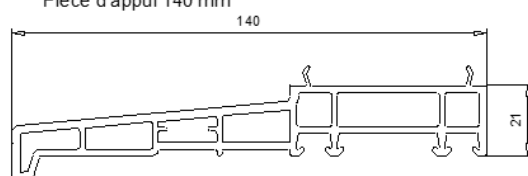
110 080 Pièce d'appui 140 mm
