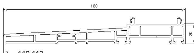
110 112 Pièce d'appui 180 mm
