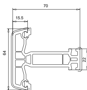
102 237 Traverse / Meneau
