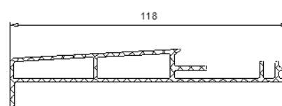
104 320 Pièce d'appui alu 72 mm
