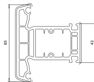
102 241 Traverse / Meneau 85 mm
