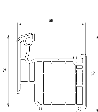
103 206 Elargisseur 72 mm
