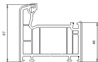
101 208 Dormant 67 mm
