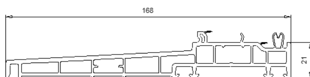
110 127 Pièce d'appui 110 mm
