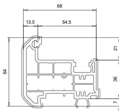
102 234 Battement rapporté 64 mm clipable pour tête de 16 Bouchon 109 598
