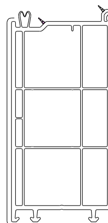
109 121.2 Elargisseur 110 mm
