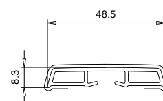
109 522 Battue 48 mm Bouchon 109 523
