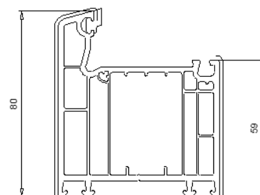
101 252 Dormant 80 mm
