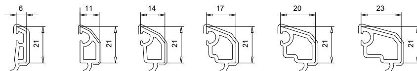
107 208 Parclose
