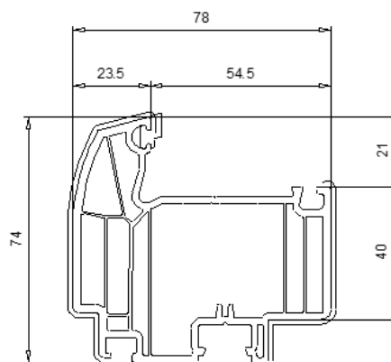
103 332 Battement monobloc 74 mm
