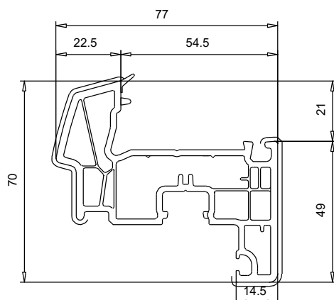
103 339 Ouvrant fenêtre
