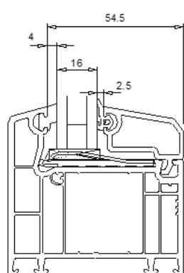
volume mini avec joint spécifique 112053
