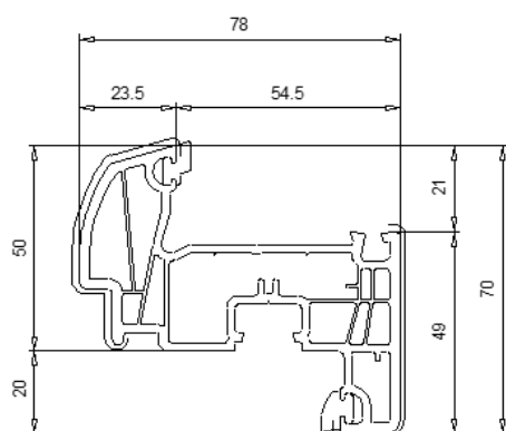
103 335 Ouvrant 70 mm
