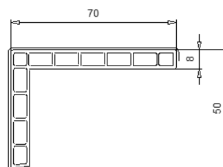
111 031 Cornière
