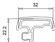
109 680 Battue 32mm Bouchon 109 684
