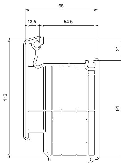
105 130 Elargisseur 112 mm
