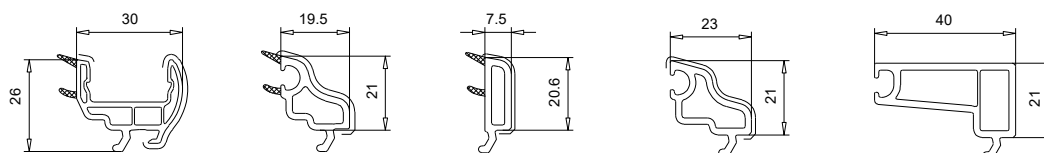
107 172 Parclose
