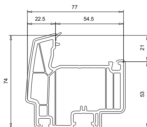
103 336 Battement monobloc ouvrant serrure
