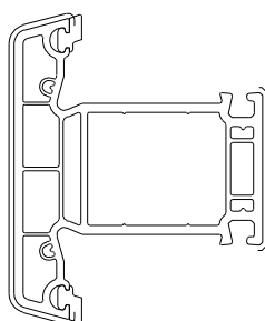
102 287 Traverse / Meneau 85 mm
