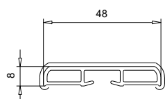
109 432 Battue 48 mm Bouchon 109 551
