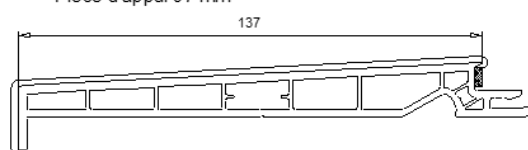
110 093 Pièce d'appui 137 mm
