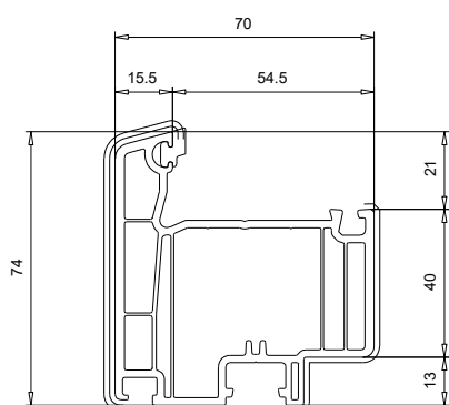
103 318 Battement Monobloc 74 mm
