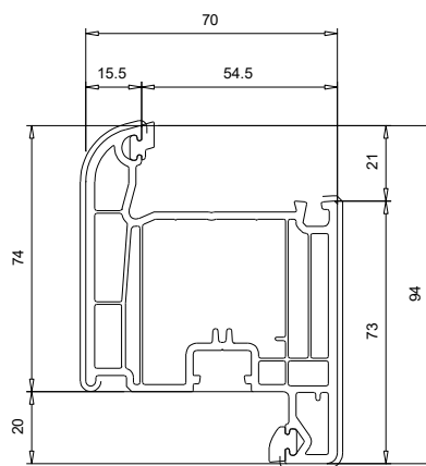
103 289 Battement Ouvrant 94 mm
