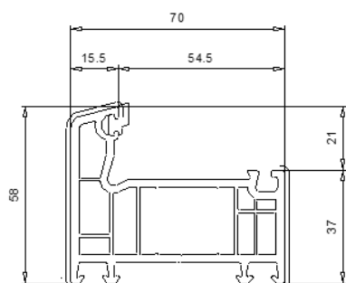
101 207 Dormant 58 mm
