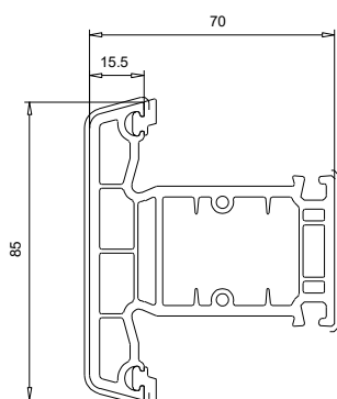
102 288 Traverse / Meneau 85 mm
