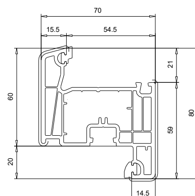
103 317 Ouvrant 80 mm
