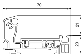
104 286 Seuil mixte aluminium - PVC 1.0
