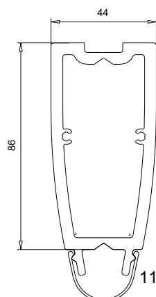
104 325 Clavette aluminium
