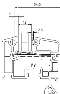
volume mini avec joint spécifique 112053
