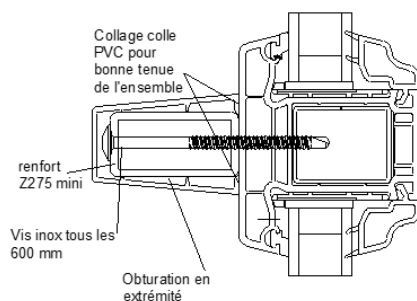
Assemblage renforcement extérieur meneau/traverse
