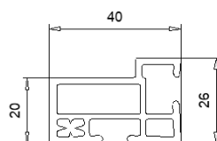
109 073 Tapée 20 mm
