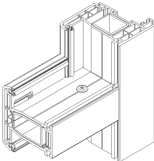
Elément de remplissage sensible à l'humidité
