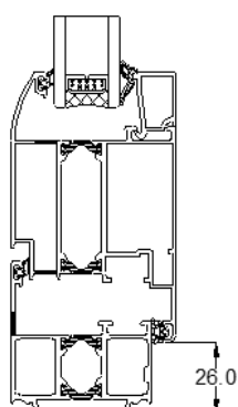
Section 2 SANS SEUIL
