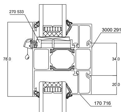
Traverse intermédiaire
