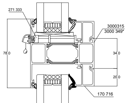
Traverse basse avec seuil PMR
