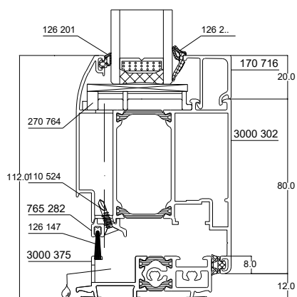
Traverse basse avec seuil PMR
