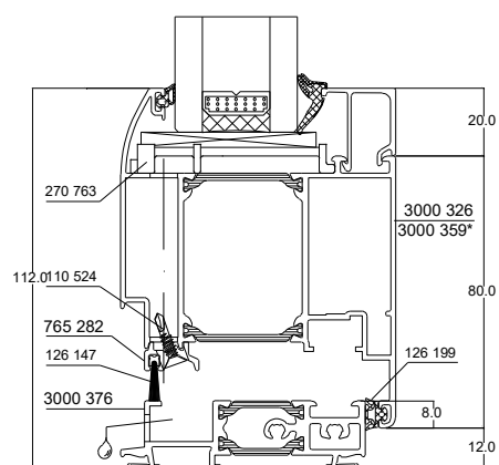
Traverse basse avec seuil PMR
