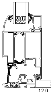
Section 2 bis AVEC SEUIL
