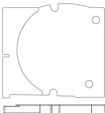
Isolation embout - coffre 195 16,5 mm G 11171799
