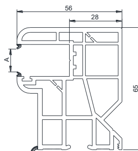
coulisse tapée 65
