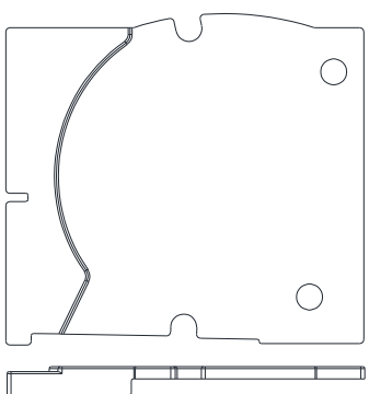
Isolation embout - coffre 195 6 mm G 11171599
