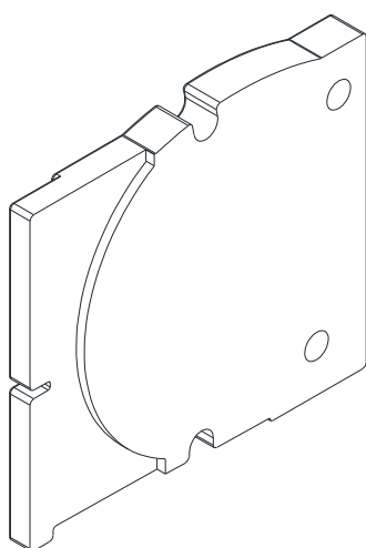
Isolation embout - coffre 195 6 mm G 11171599
