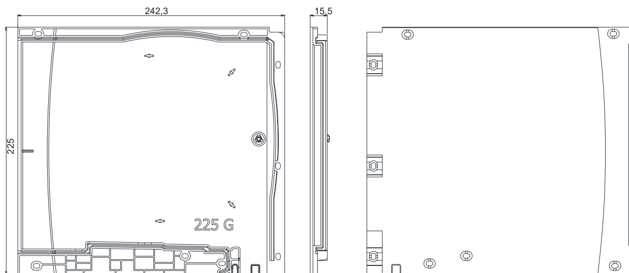
EMBOUT 225 G : 111727 EMBOUT 225 D : 111728
