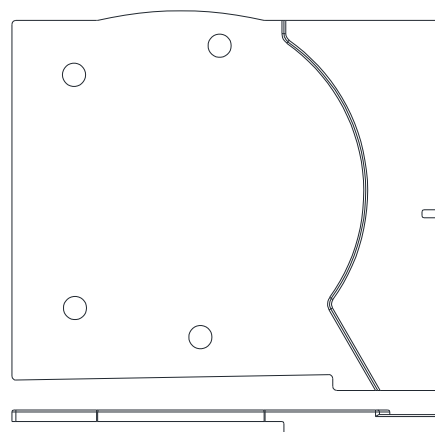
ISOLATION EMBOUT 225 6 D : 11172099
