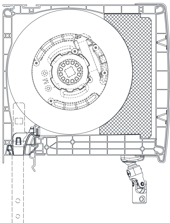
Treuil
