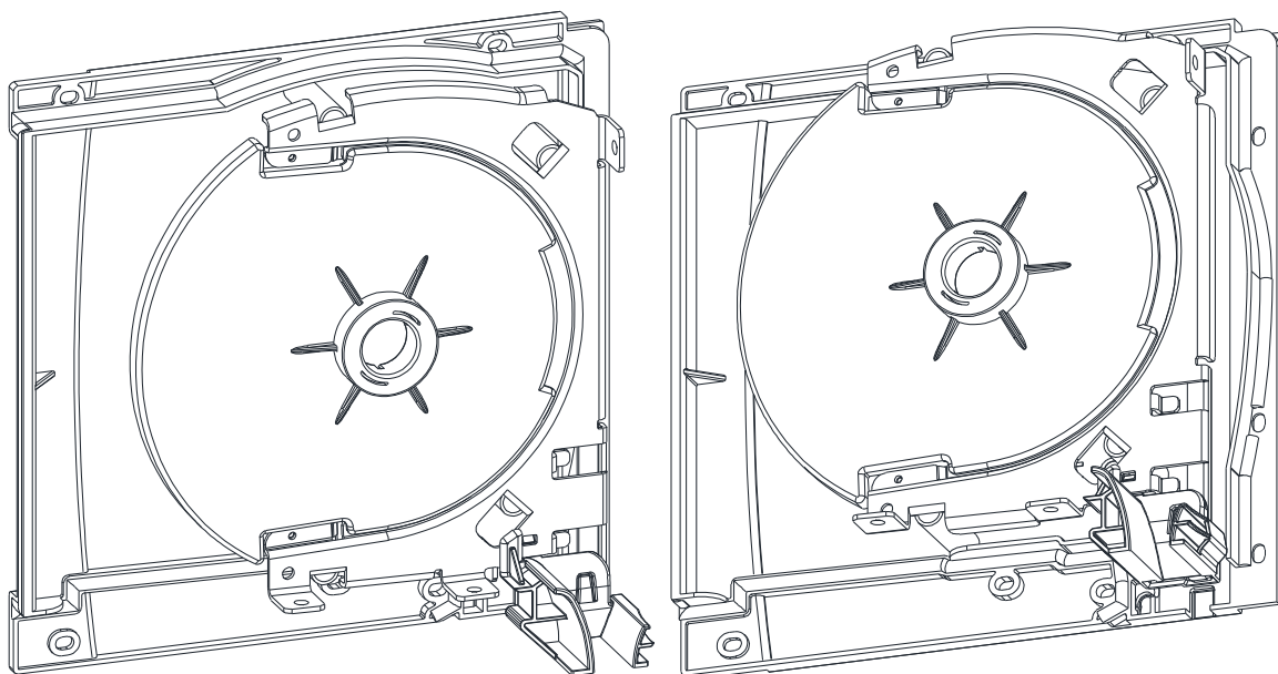
PRE MONTAGE DE LA TULIPE SUR L'EMBOUT
