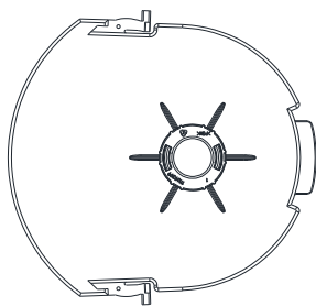
TIROIR PALIER 195 : 11173799-11283299 TIROIR PALIER 225 : 11173899
