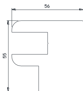
PLAQUETTE PE POUR COULISSE TAPEE 55 11029399
