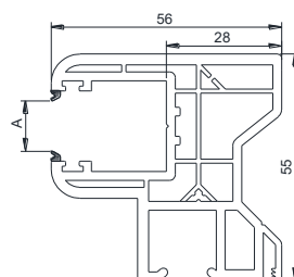
coulisse réno 40
