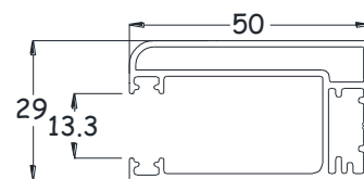
COULISSE ALUMINIUM ASB50 03036
