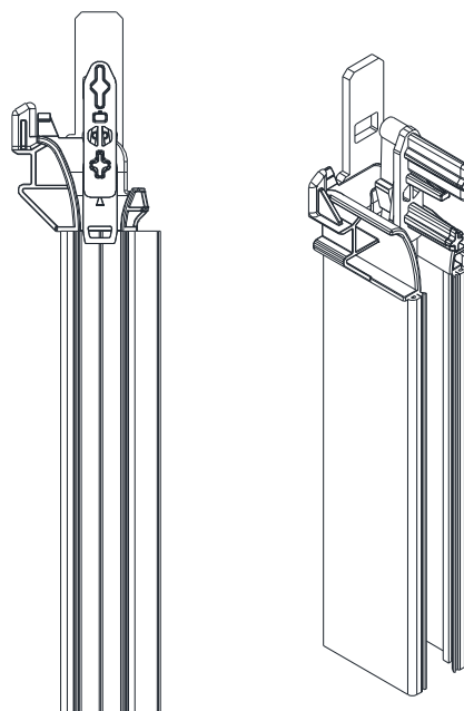
NON ARRET DE LA BUTEE SUR LA TULIPE EN SAV
