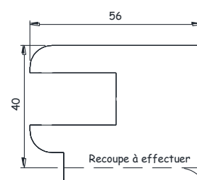
PLAQUETTE PE POUR COULISSE TAPEE 40 11029199
