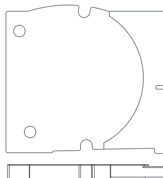
Isolation embout - coffre 195 16,5 mm D 11171899
