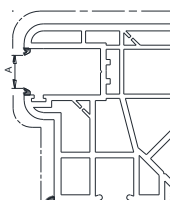
coulisse tapée 65
