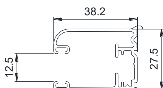
Coulisse monobloc passage réduit aluminium 0333
