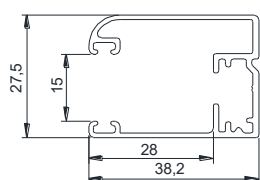
COULISSE MONOBLOC SANS BECQUET ALUMINIUM 0323
