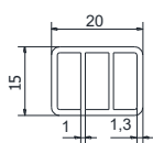
Calage de 20 x 15 DV0074
