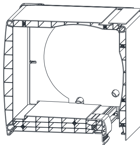
Coffre 195 : isolant 16,5 mm
