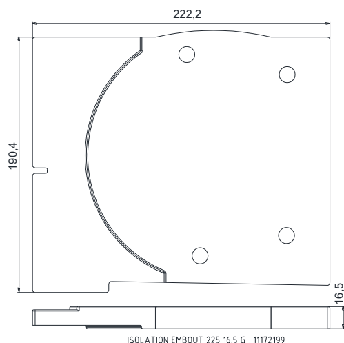
ISOLATION EMBOUT 225 16.5 G : 11172199
