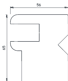
PLAQUETTE PE POUR COULISSE TAPEE 65 11029299
