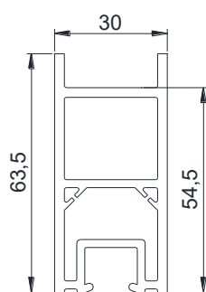
meneau 63X30 RC0003
