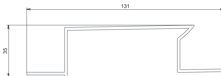
Renfort screen alu supérieur 03040
