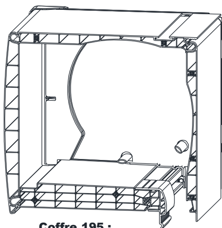
Coffre 195 : isolant 6 mm
