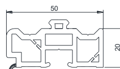
Calage tapée CT0099
