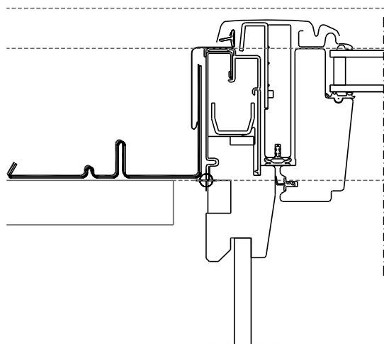
FENETRE ET POSITION GENERATION 1992 ET ANTERIEURE
