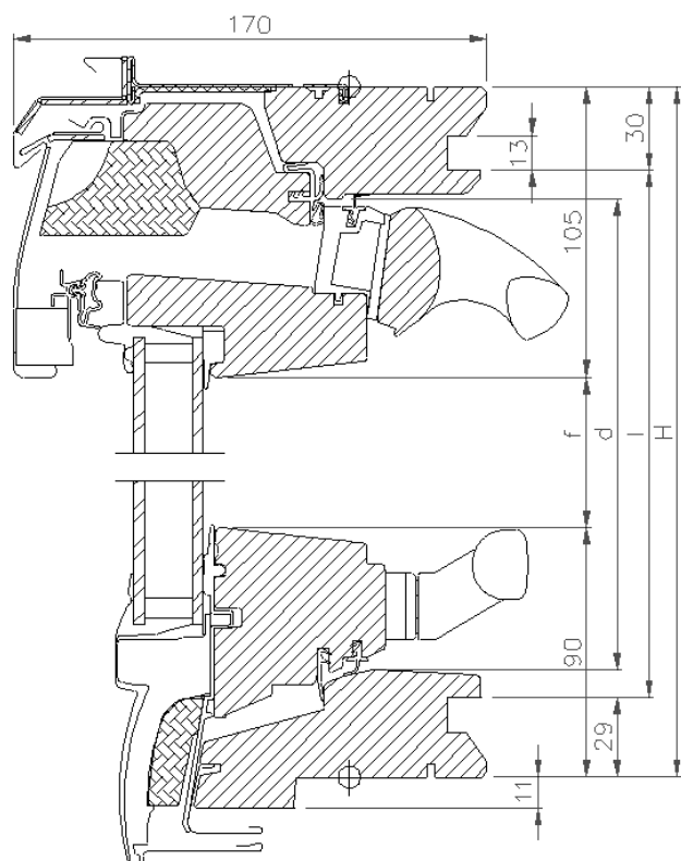
Coupe verticale
