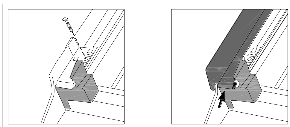
Emboîtement Profilé Lateral Encastré
