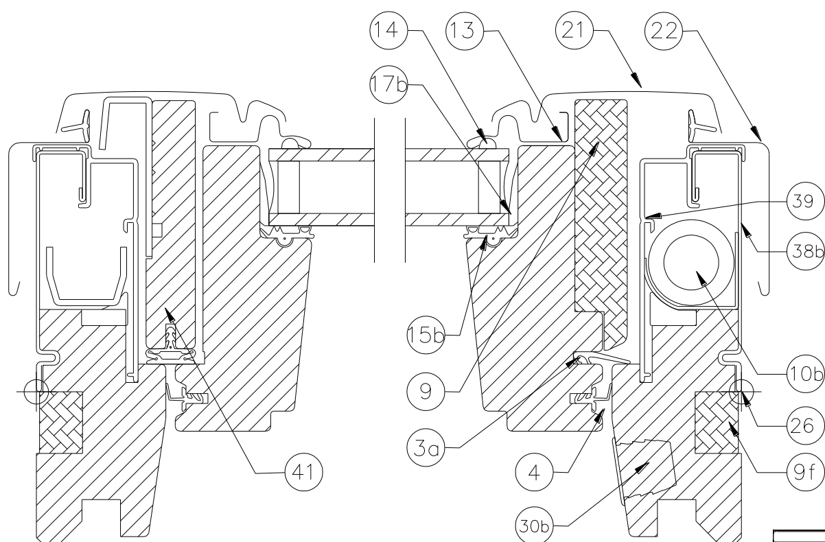
Coupe horizontale
