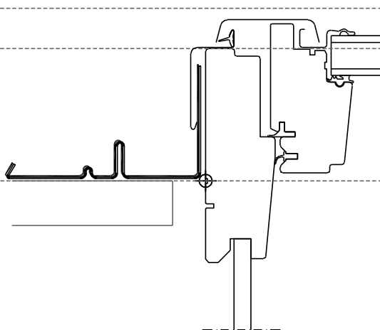
FENETRE NOUVELLE GENERATION ET POSITION 'RENOVATION'
