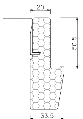
TRAVERSE HAUTE
