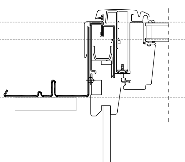
FENETRE NOUVELLE GENERATION ET POSITION 'RENOVATION'
