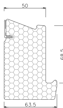
TRAVERSE BASSE
