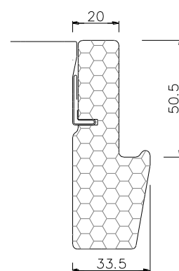
TRAVERSE BASSE
