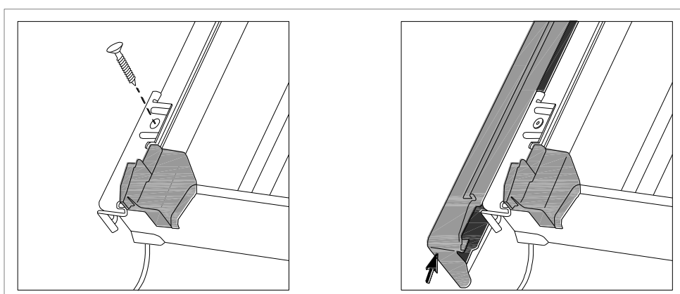
Emboîtement Profilé Lateral Standard
