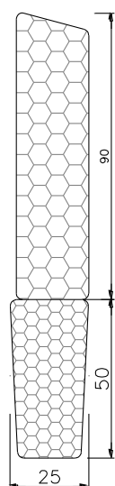
TRAVERSE HAUTE
