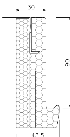
MONTANT
