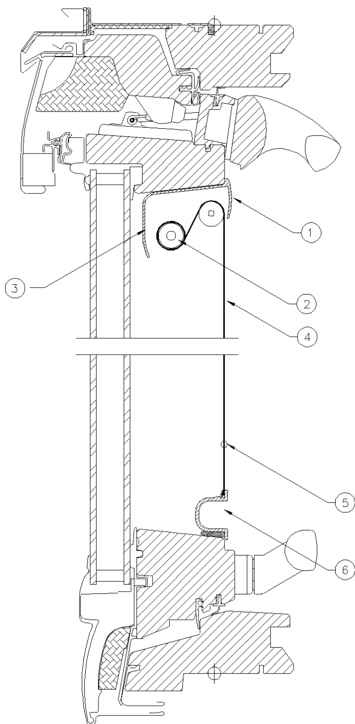
Coupe horizontale
