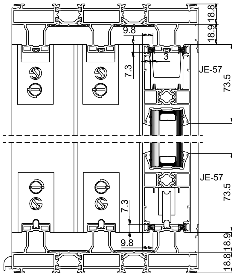
(COUPE VERTICALE)
