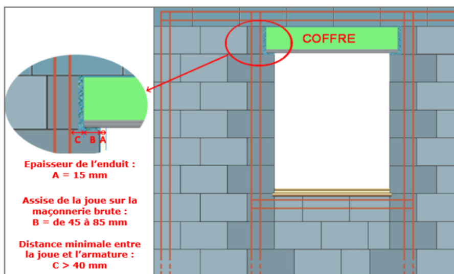
II.2.5 Pose en maçonnerie sismique = passage du pilier dans la joue, vue de face. Largeur minimale du chaînage \geq 150 mm
