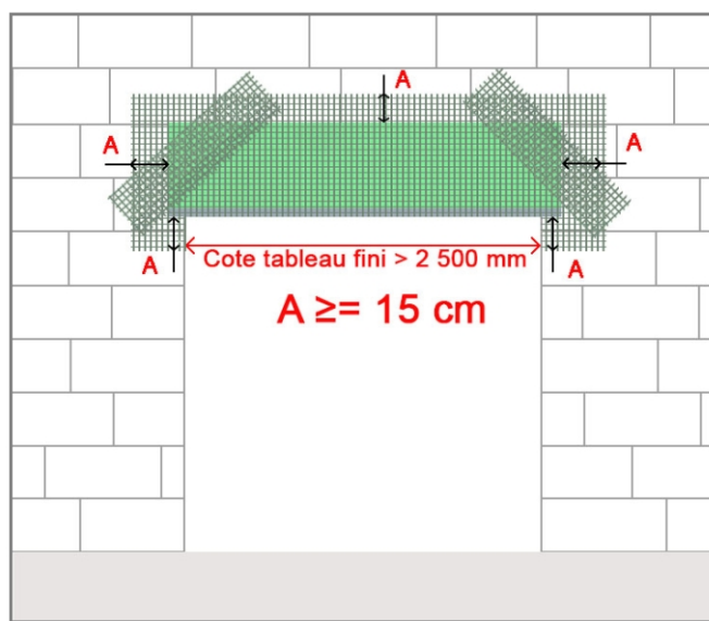
III.3 Renforcement de l'enduit au-delà de 2500 mm
