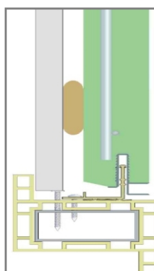
PVC à languette + renfort
