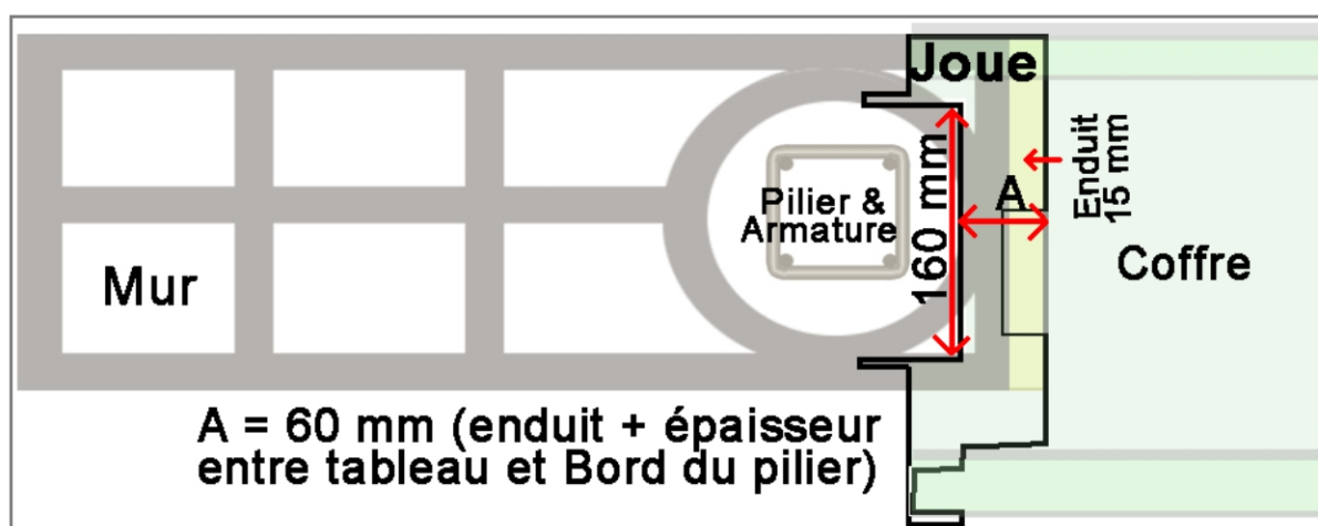
II.2.2 Vue du dessus
