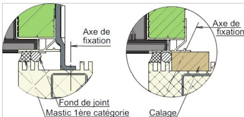
Coupe au niveau du renfort linteau additionnel
