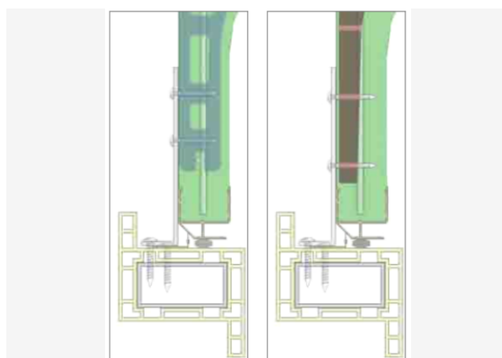
Rail PVC à languette + renfort
