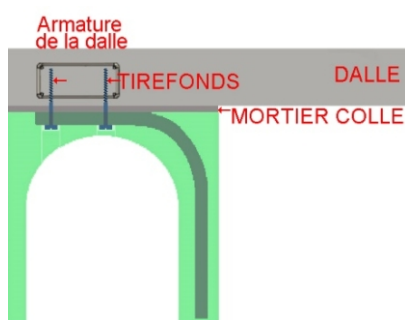
Pose sous dalle, en réservation avec les renforts et des tirefonds
