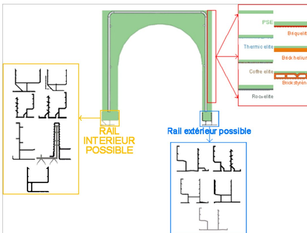
I.2 Composition et définition d'un coffre
