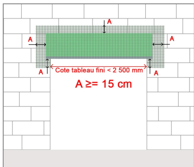
III.2 Renforcement de l'enduit jusqu'à 2500 mm
