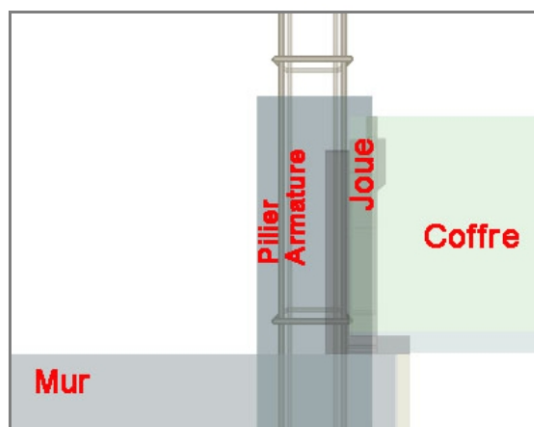
II.2.1 Pose en maçonnerie sismique = passage du pilier dans la joue, vue de face, côté extérieur
