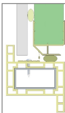
Rail PVC à languette
