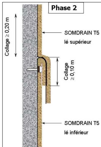
Figure 15 - Réparation en zone encollée : phase 2
