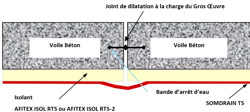
Figure 13 - Traitement des joints de dilatation sur voile béton
