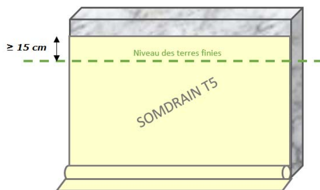
Figure 6b : positionnement du SOMDRAIN® T5 sur support en béton banché \geq 15 \text{ cm}
