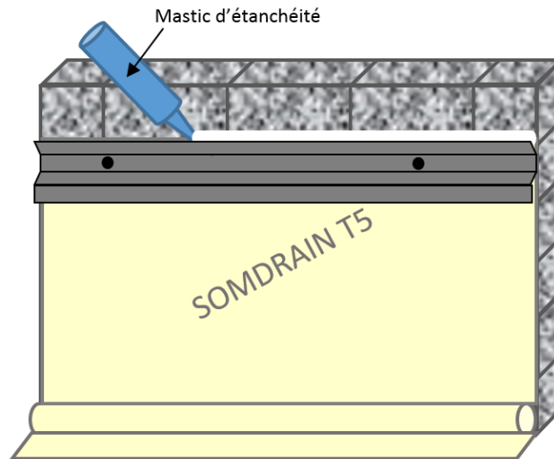
Figure 5e : Mise en place du mastic d'étanchéité sur le solin
