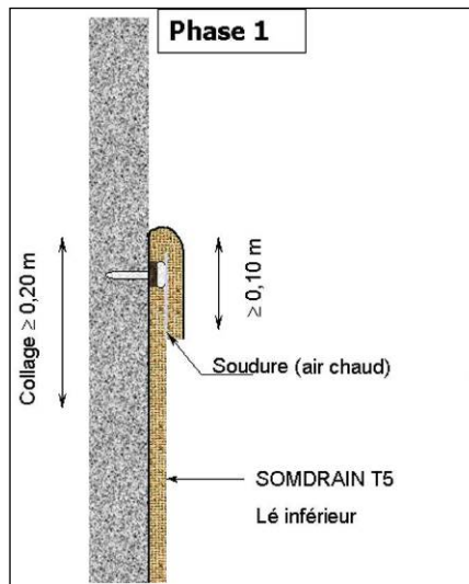
Figure 14 - Réparation en zone encollée : phase 1
