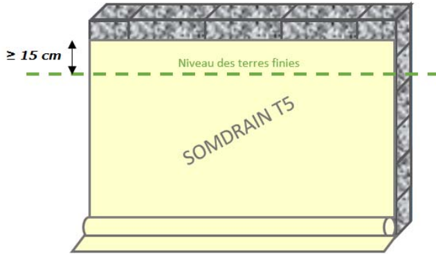
Figure 5c : positionnement du SOMDRAIN® T5 sur le support en parpaing
