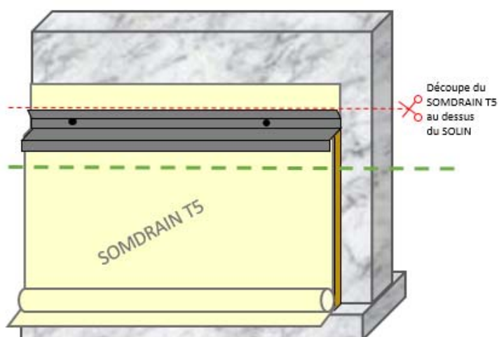
Figure 7e : positionnement du solin compatible avec un isolant et découpe du SOMDRAIN® T5
