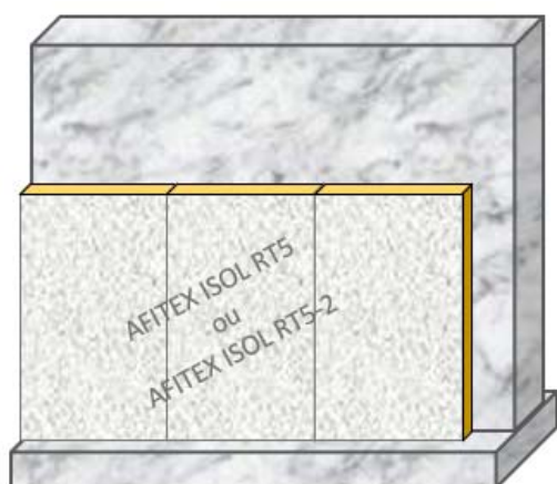
Figure 7c : positionnement des isolants AFITEX ISOL RT5 ou AFITEX ISOL RT5-2
