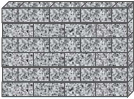
Figure 5a : support en parpaing nu – mur de type II et III uniquement et avec aspérités \leq 2 mm sous la règle des 20 cm
