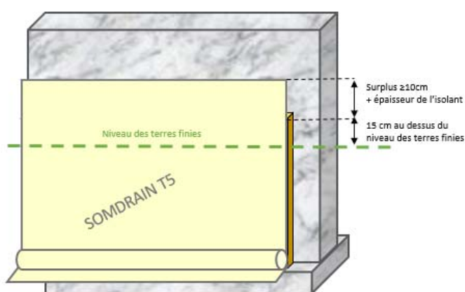
Figure 7d : positionnement du SOMDRAIN® T5 sur l'isolant AFITEX ISOL RT5 ou AFITEX ISOL RT5-2 support en béton banché
