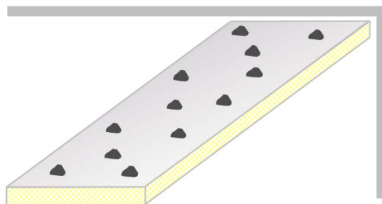
Figure 7b : positionnement des plots d'AFICOL RT5 sur l'isolant AFITEX ISOL RT5 ou AFITEX ISOL RT5-2
