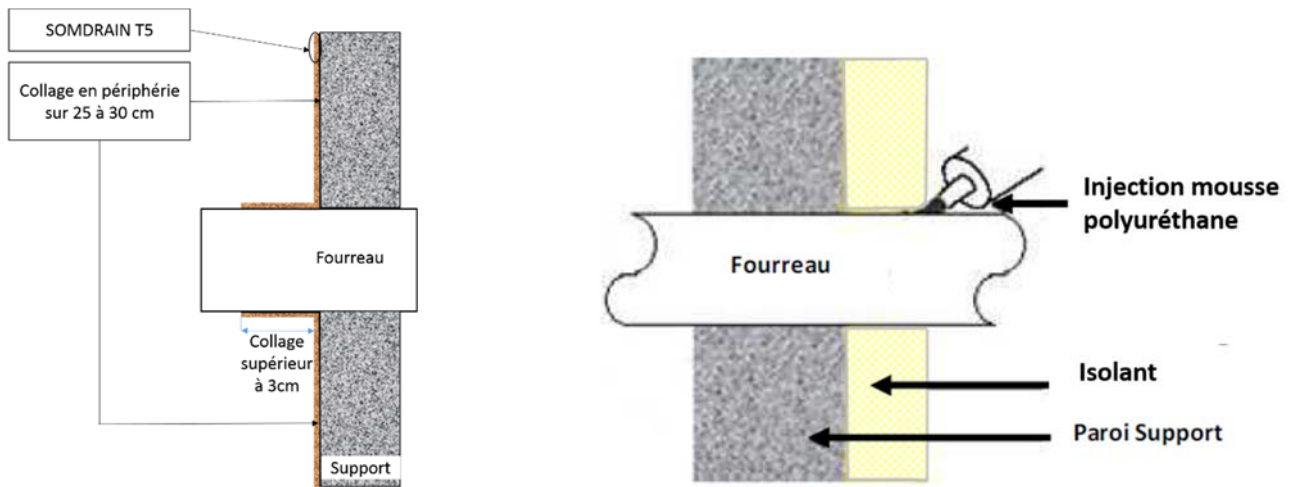
Figure 12 - Traitement des pénétrations
