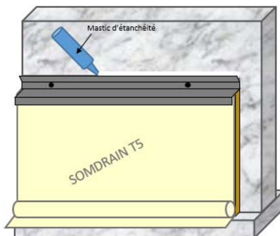
Figure 7f : Mise en place du mastic d'étanchéité sur le solin
