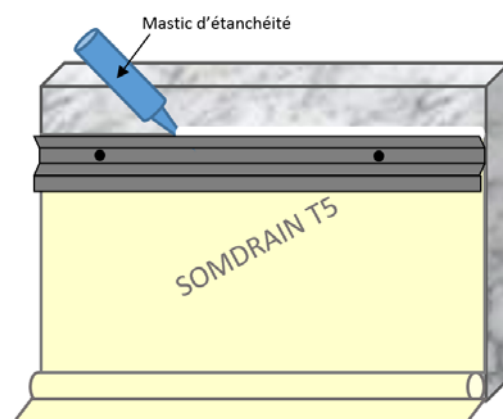
Figure 6d : Mise en place du mastic d'étanchéité sur le solin
