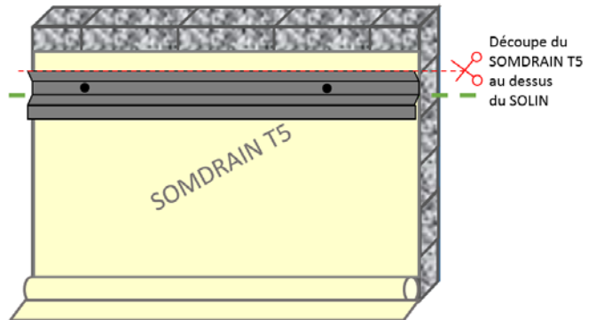
Figure 5d : positionnement du solin et découpe du SOMDRAIN® T5 sur le support en parpaing
