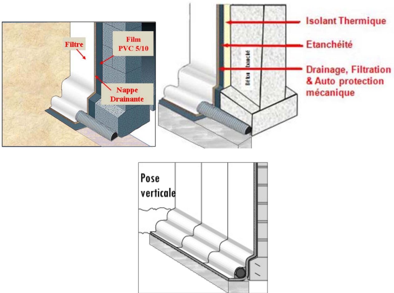
Figure 1 - Orientation du SOMDRAIN® T5 par rapport au support
