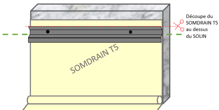
Figure 6c : positionnement du solin et découpe du SOMDRAIN® T5
