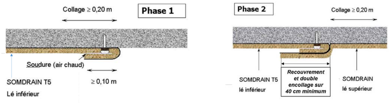
Figure 16 - Fermeture de l'étanchéité (lorsque le SOMDRAIN® T5 fait le tour du bâtiment)
