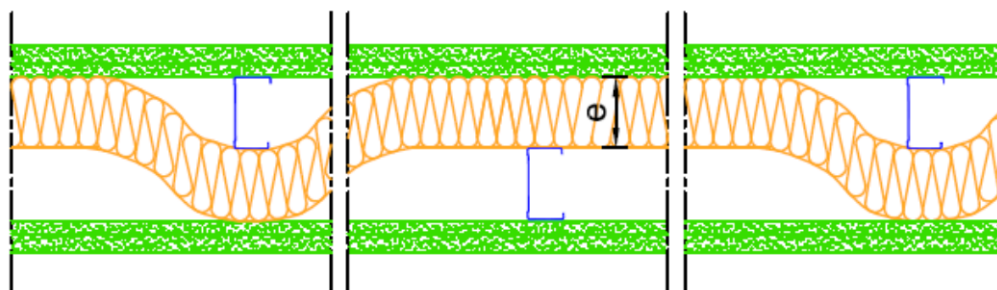
Figure 2 – Coupes horizontales – Cloison PREGYMETAL S (cf. article 2.4.3.4) et PREGYMETAL S TWIN
