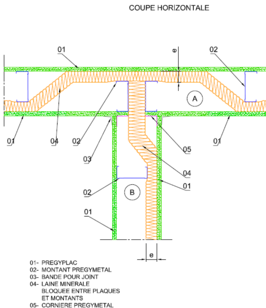
Figure 5 – Coupe horizontale – Jonction en T – Cloisons PREGYMETAL S et PREGYMETAL S TWIN
