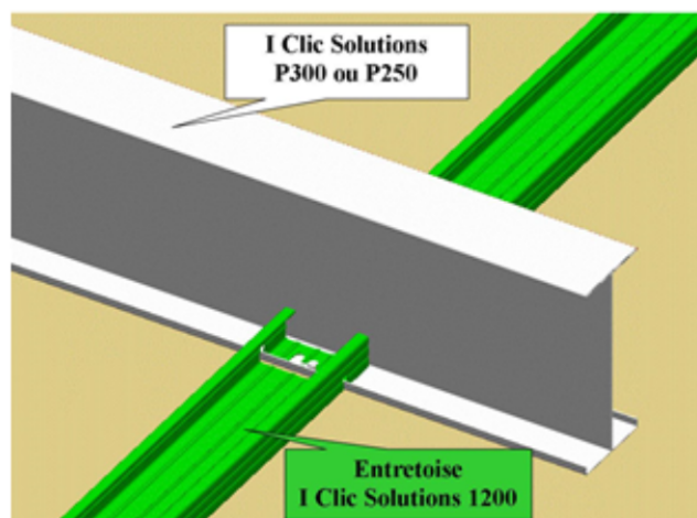
Figure 4 : Entretoise F45-18 1200
