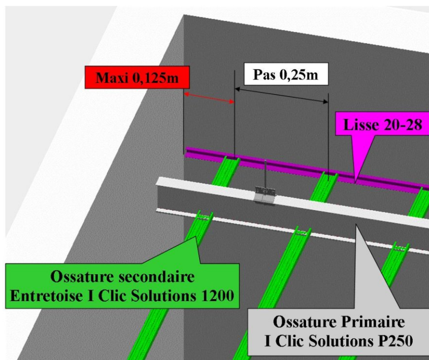
Figure 15d : I Clic Solutions P250 avec Ossature secondaire au pas de 0,25m (sans Rail R101)
