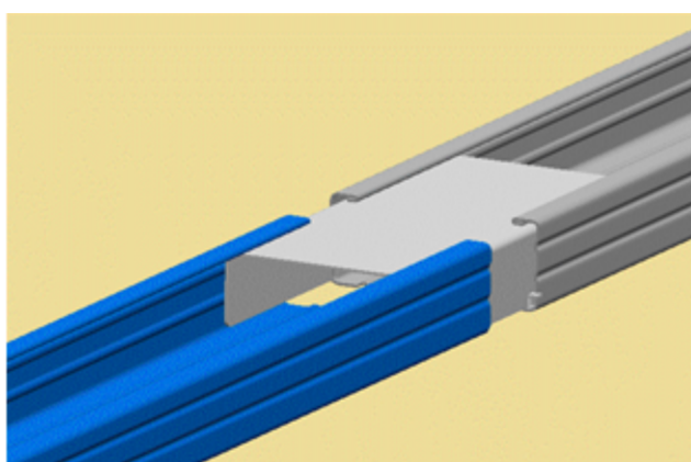
Figure 7 : Eclisse Fourrure
