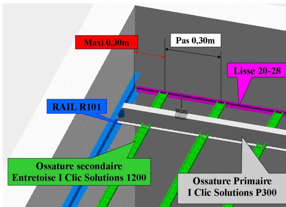
Figure 14b : I Clic Solutions P300 avec Ossature secondaire au pas de 0,30m
