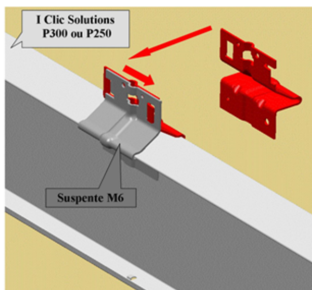
Figure 8 : Suspente M6
