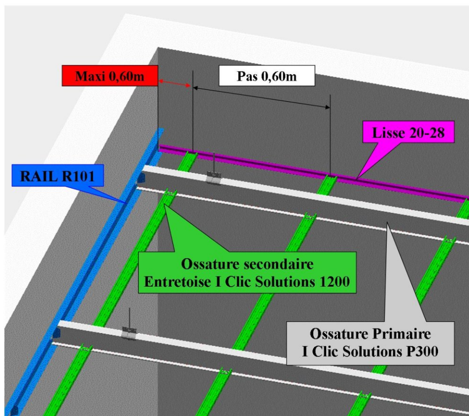
Figure 14a : I Clic Solutions P300 avec Ossature secondaire au pas de 0,60m.
