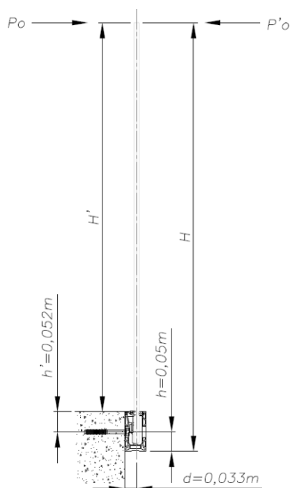
Figure 15 – Dimensionnement des chevilles de fixation montage latéral
