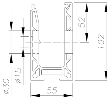
Figure 3 – Modèle OSF – Pose latérale
