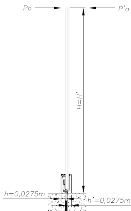
Figure 14 – Dimensionnement des chevilles de fixation montage sur dalle
