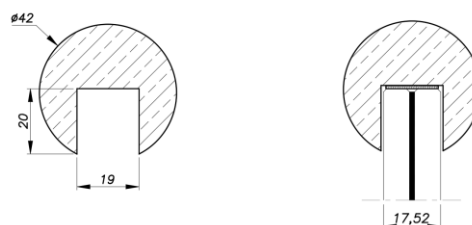
Figure 21 – Exemple de main courante
