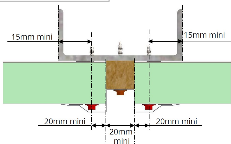
Figure 27 - Jonction en pose horizontale avec fixations traversantes (en complément de celles prévues dans l'emboîtement)
