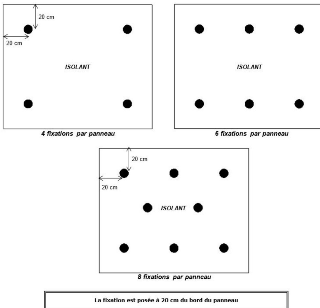
Figure 2 – Implantation des fixations en fonction de leur nombre
