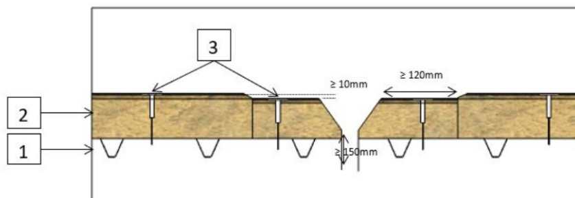
Figure 4 - Coupe sur l'isolation au droit d'une évacuation d'eau « en fond de noue »
