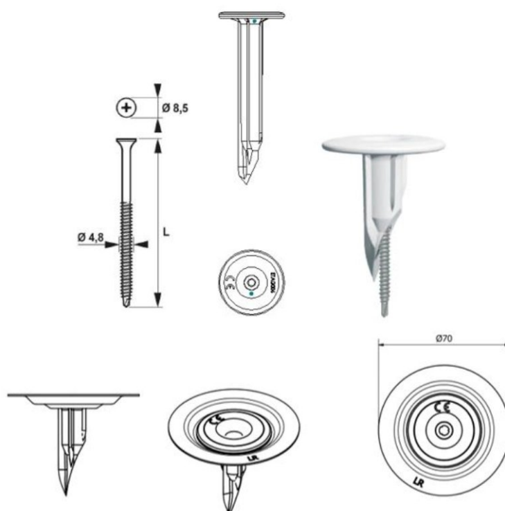
Figure 5 – Vue de coupe du fût ETANCOPLAST HP4L
