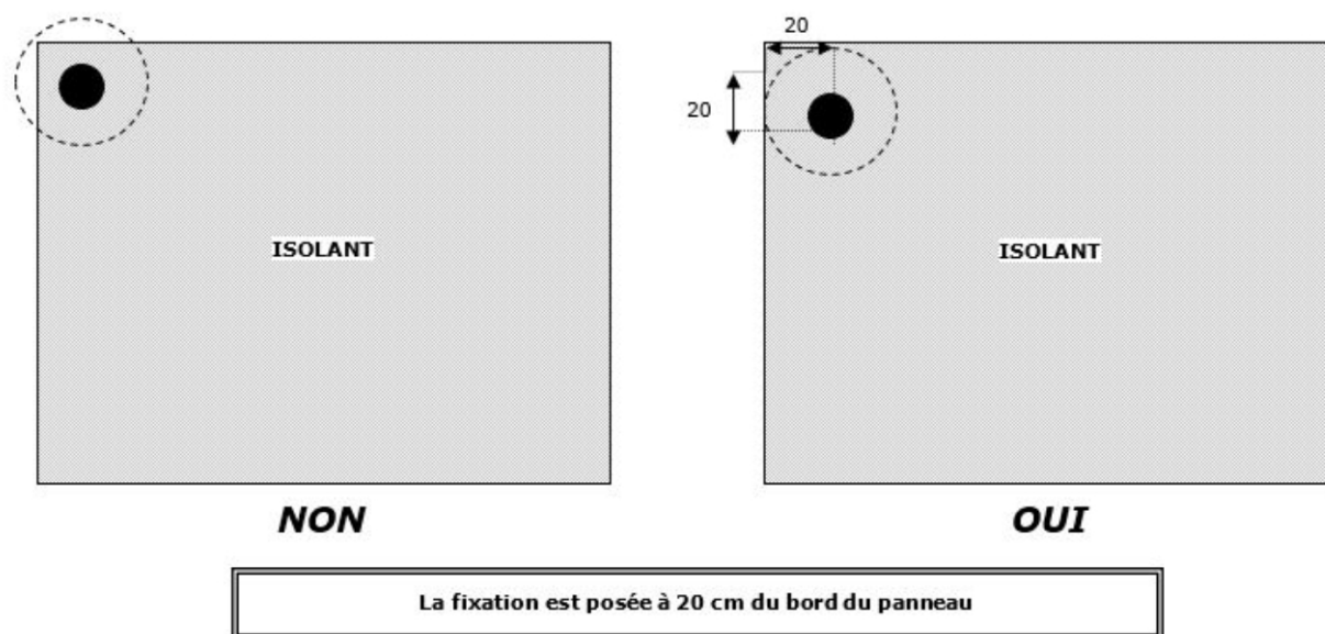
Figure 1 – Implantation des fixations pour une mise en œuvre du revêtement en adhérence
