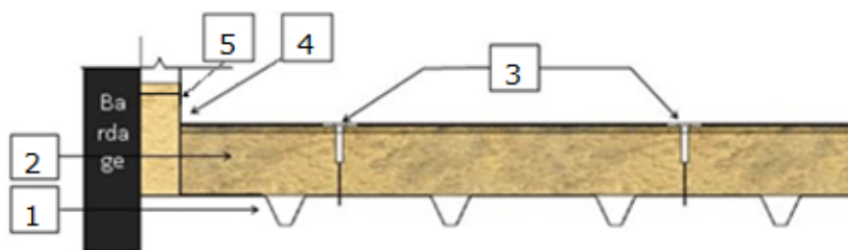
Figure 3 - Principe de relief isolé sur tôles d'acier nervurées
