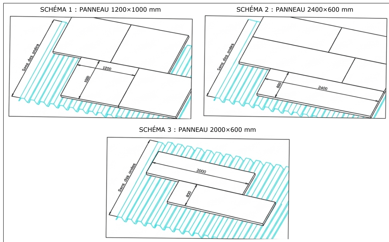
Figures de principe - Orientation des panneaux Rockacier C Nu Energy sur TAN conformes au NF DTU 43.3 ou au Cahier du CSTB 3537_V2
