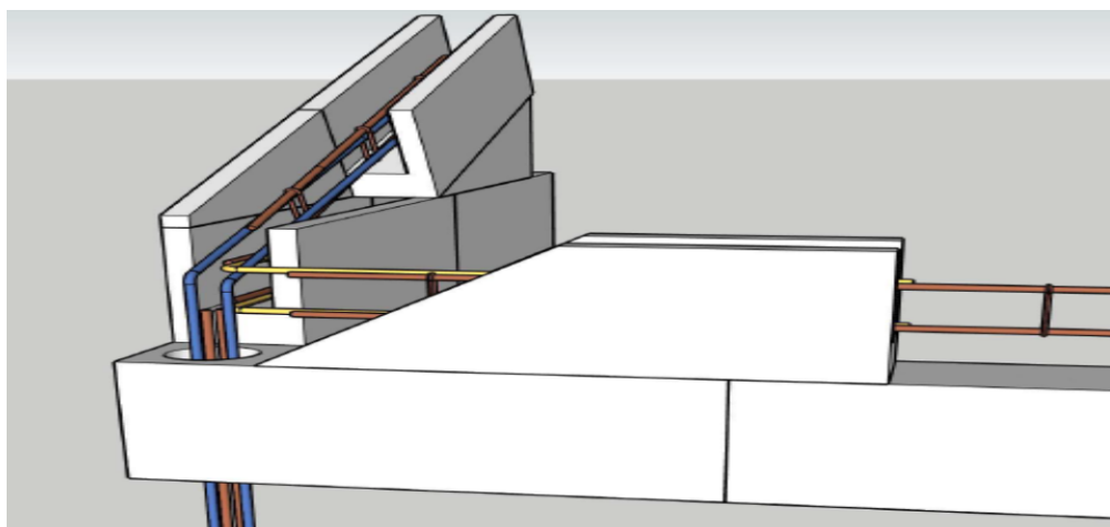
Figure 12 : Elévation d'un angle de mur Ytong Compact 15 au droit du pignon Principe de liaison chaînage vertical / chaînage horizontal / chaînage sous rampant
