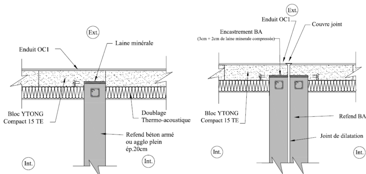
Figure 16 : Jonction entre façade et refend en béton armé ou en bloc béton - Cas de refend séparatifs entre différents locaux
