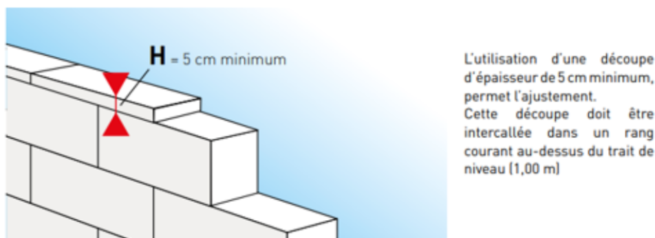
Figure 5 : Découpe horizontale des blocs en rang courant
