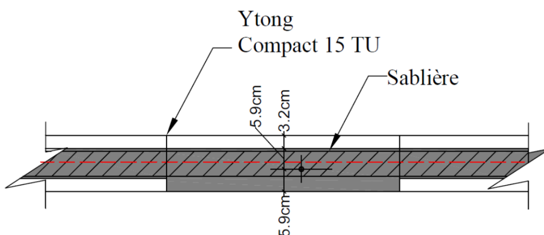
Figure 19 : Modes de fixation de la charpente industrielle sur le chaînage horizontal de couronnement avec une cheville de 6 mm de diamètre
