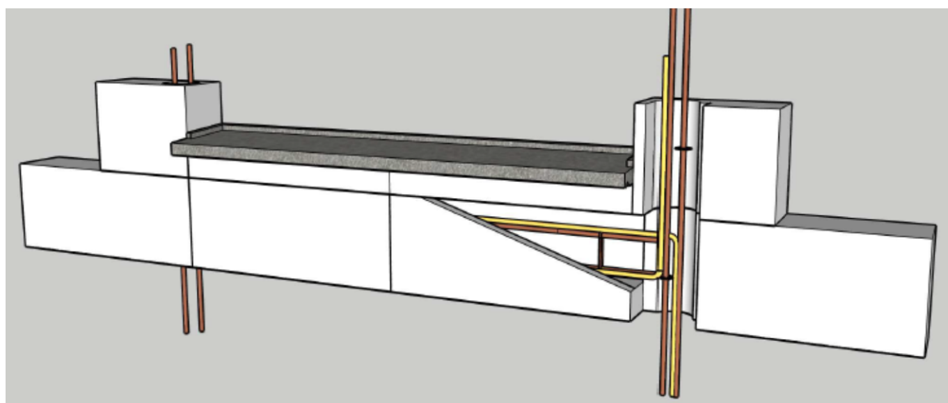
Figure 18 : Réalisation des tableaux de baie Elévation sur chaînages verticaux au droit d'une ouverture Principe de liaison d'armatures entre le renfort d'allège et les chaînages verticaux
