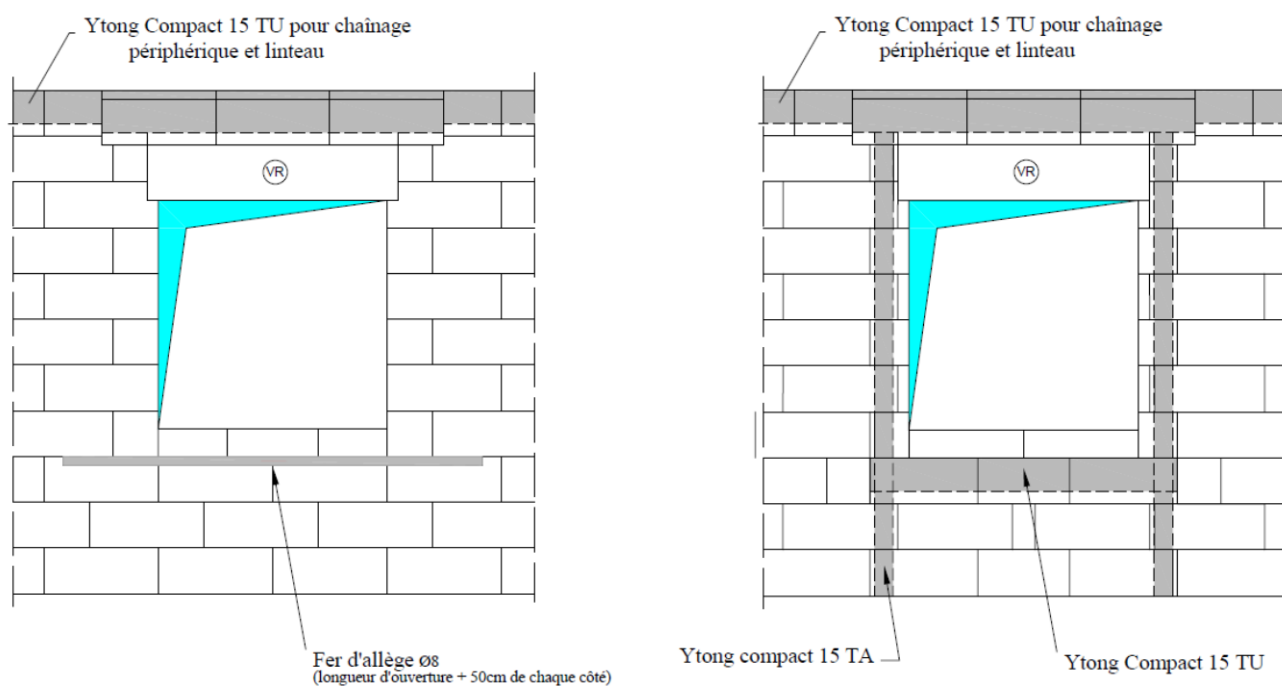
Figure 17 : Elévations au droit d'une ouverture
