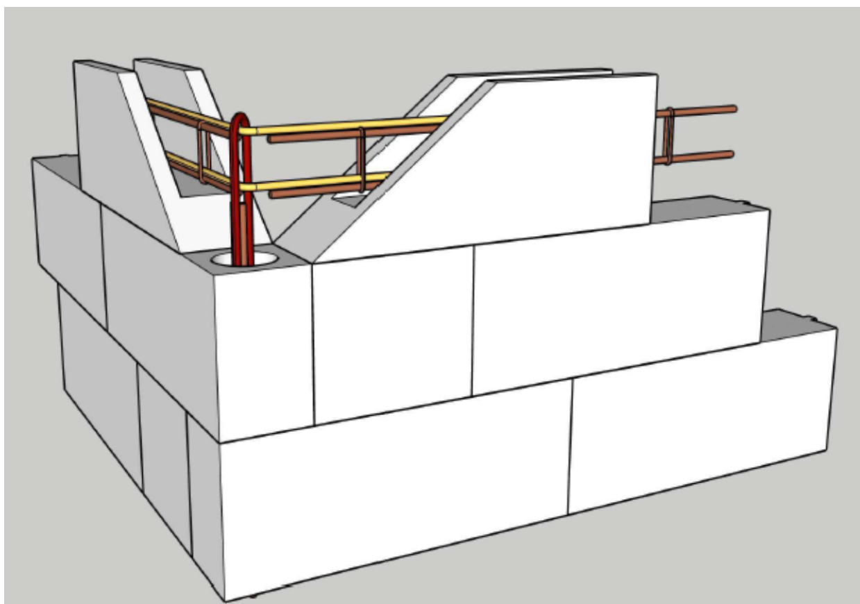
Figure 9 : Elévation d'un angle de mur Ytong Compact 15 Principe de liaison chaînage vertical / chaînage horizontal
