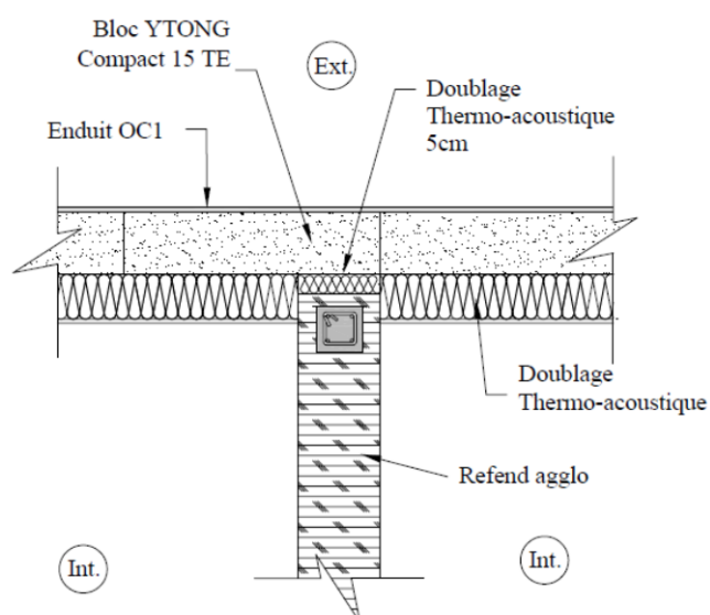
Figure 15 : Cas de refend non séparatifs (façade Ytong Compact 15 / refend en bloc béton)
