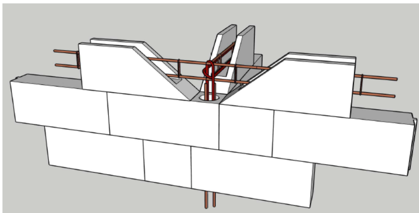
Figure 14 : Elévation sur jonction façade/refend en béton cellulaire Ytong Compact 15
