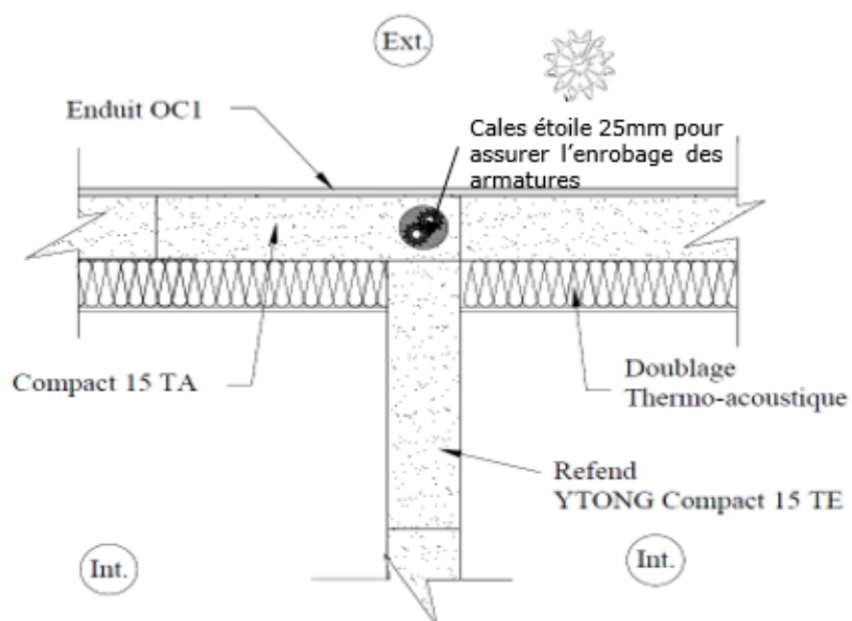
Figure 13 : Jonction façade refend Ytong compact 15 – vue en plan
