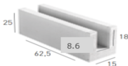
Figure 3 : Bloc de chaînage horizontal
