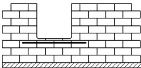
Figure 7 : Renfort par fer d'allège
