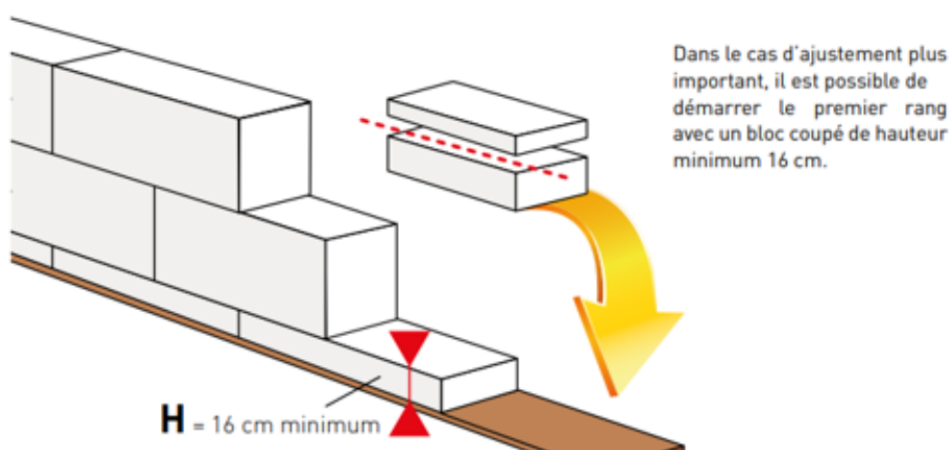
Figure 6 : Découpe horizontale des blocs en premier rang
