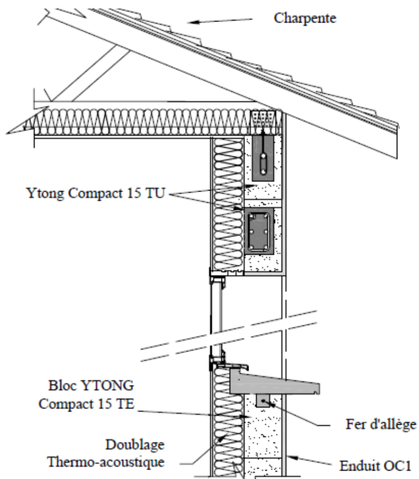
Figure 11 : Coupe sur Chaînage horizontal et linteau ajusté avec blocs Ytong Compact 15 TU
