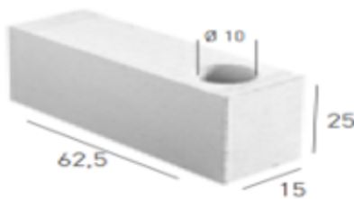
Figure 2 : Bloc de chaînage vertical
