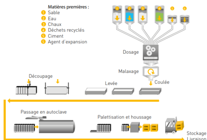
Figure 8 : Illustration du processus industriel de fabrication des éléments en béton cellulaire
