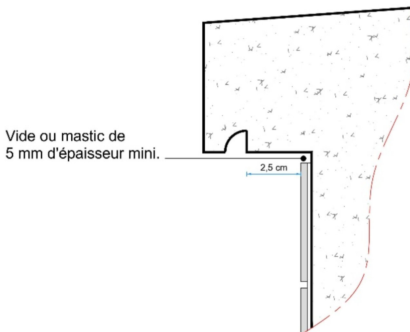
Figure 5 - Traitement acrotère
