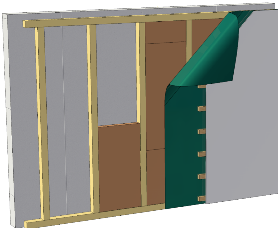
Figure 1-Isolation intérieure sur mur extérieur (maçonnerie ou béton) en ossature bois
