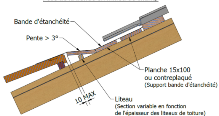
Pose de la bande en milieu de champ
