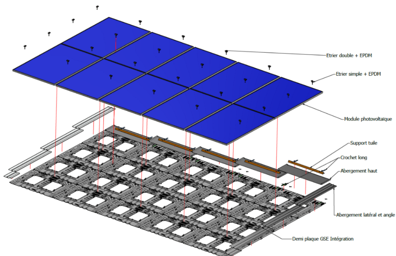
Figure 2 – Schéma éclaté du procédé
