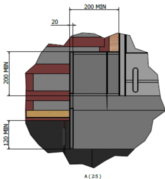
Figure 33 – Mise en œuvre du bas de champ (kit A-2)
