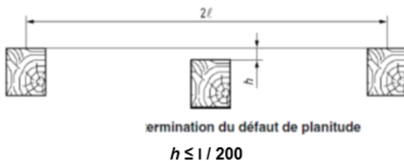
Figure 18 – Contrôle de la planitude
