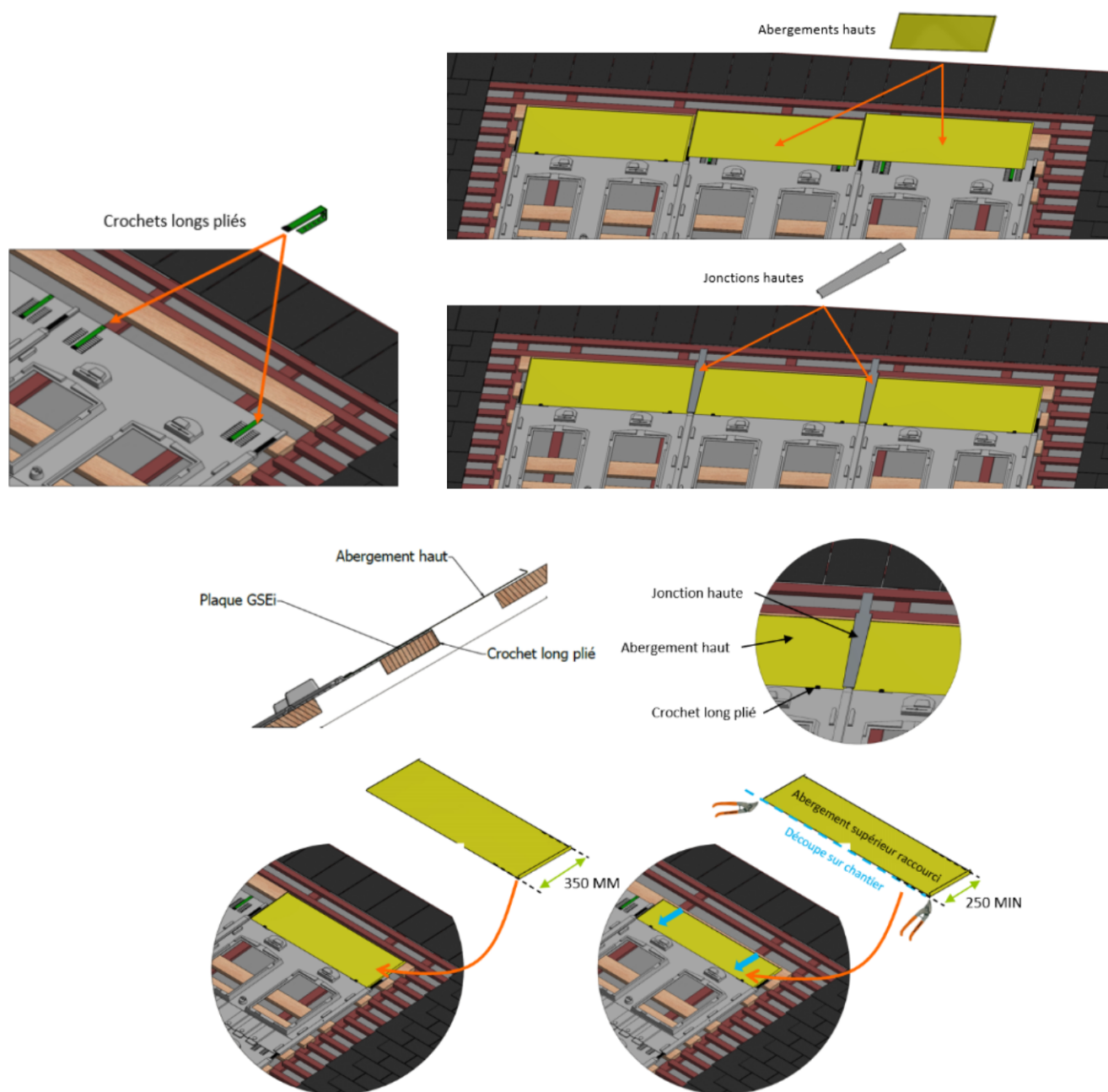
Figure 34 – Pose des abergements supérieurs (kit A-2)
