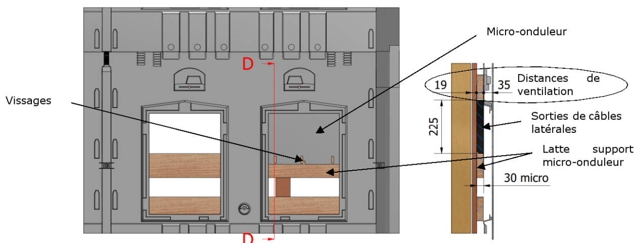
Exemple d'un micro-onduleur par module
