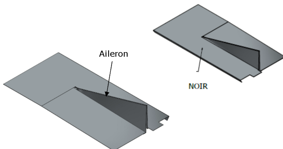
Figure 10 – Abergements supérieurs kit A-2 (et kit TP-1)
