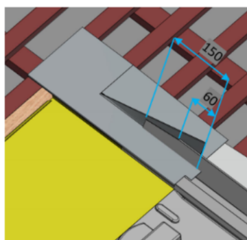
Fig 1. Cotes de recouvrement
