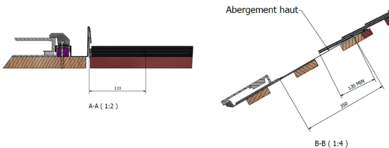
Figure 36 – Mise en place des éléments de couverture (kit A-2)
