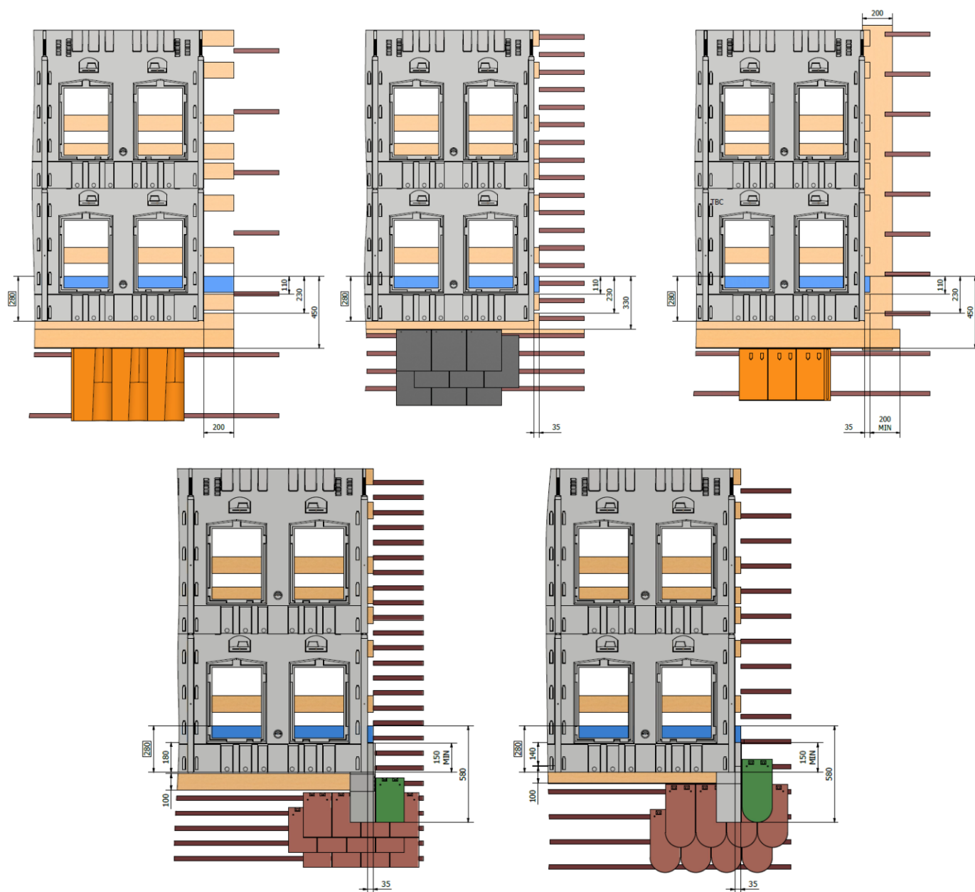
Figure 21 – Détail de la position de la latte de référence – plaque DPo_1650_XXX et DPo_1840_XXX
