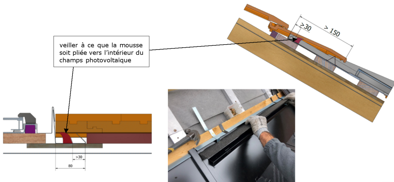
Figure 42 – Mise en place des éléments de couverture (kit TN-1)
