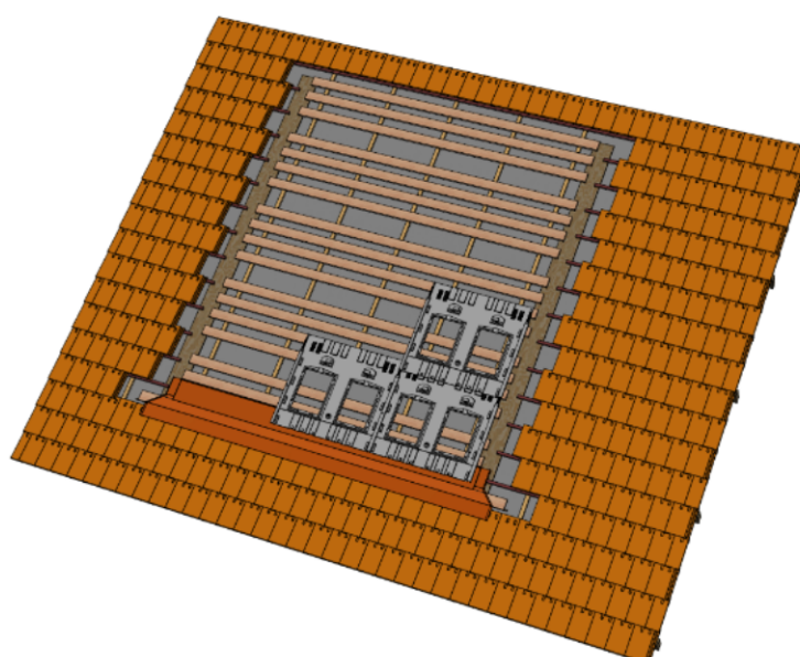
Figure 39 – Mise en œuvre du bas de champ (kit TN-1)
