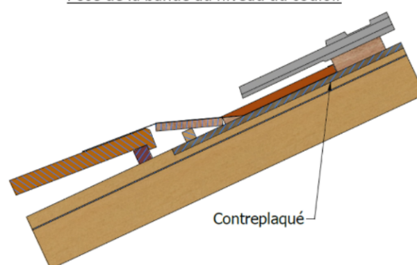
Pose de la bande au niveau du couloir
