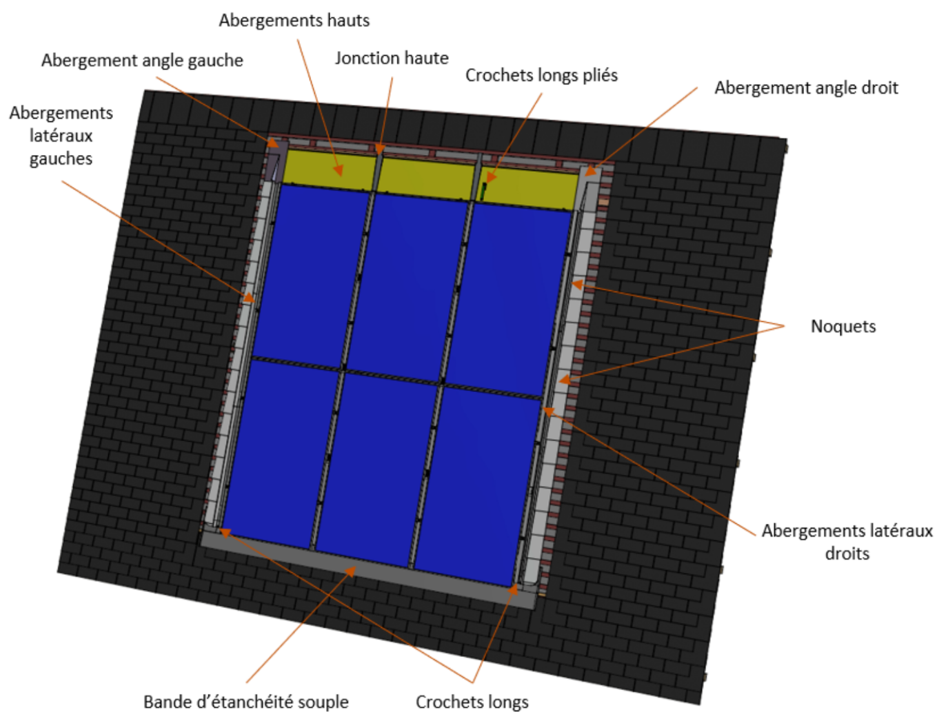
Figure 37 – Éléments du kit A-2 mis en œuvre
