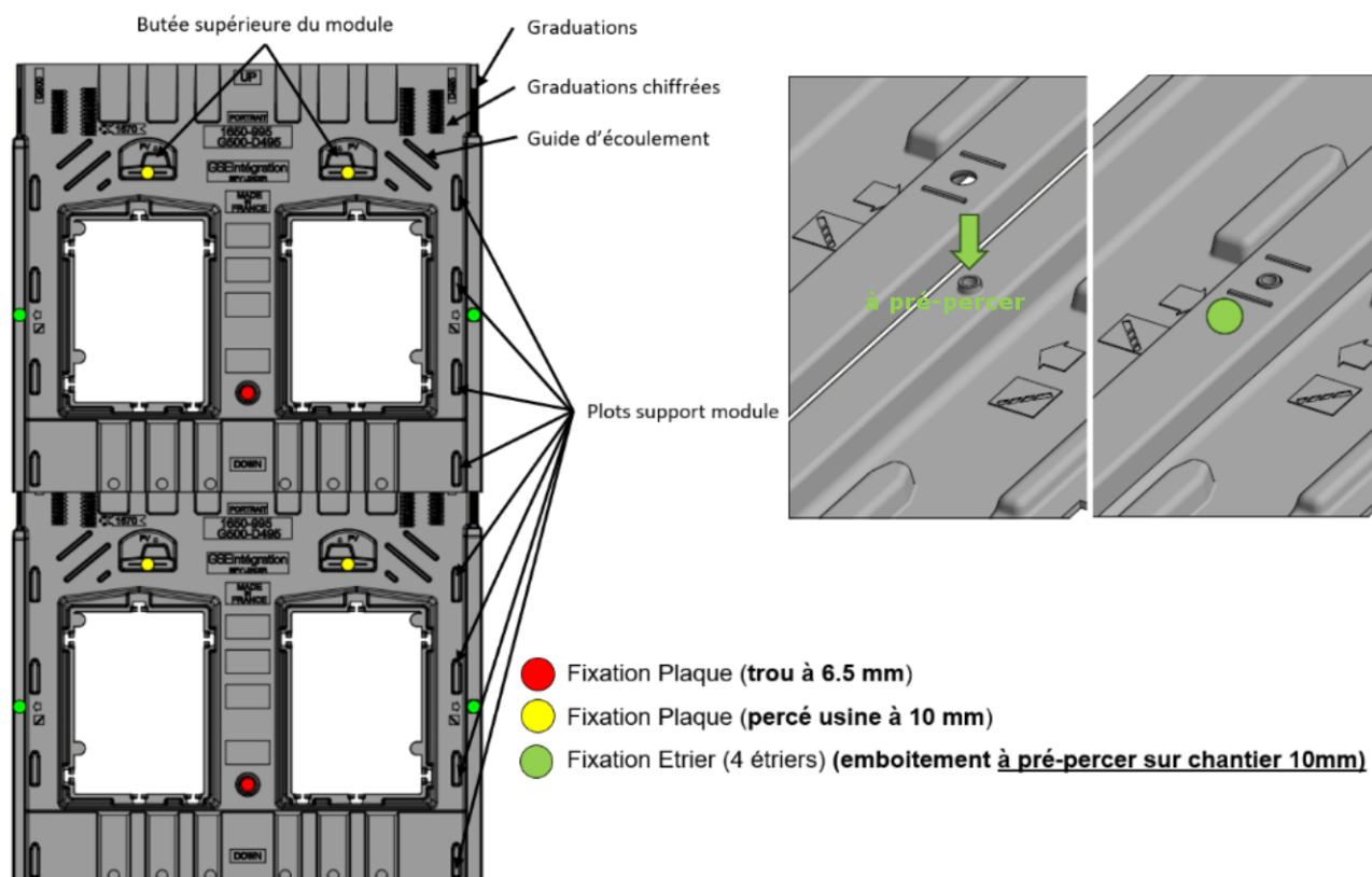
b. Vues et coupes de la plaque : cotes communes à toutes les plaques DPo_1650
