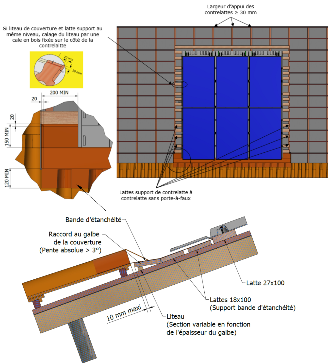
Figure 26 – Mise en œuvre du bas de champ (kit TS-2)
