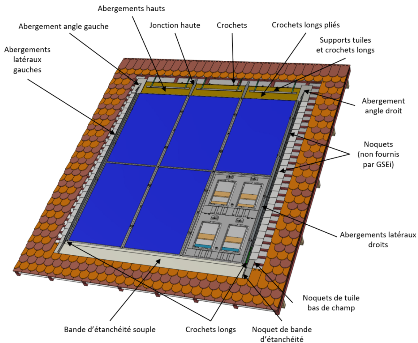
Figure 51 – Éléments du kit TP-1 mis en œuvre
