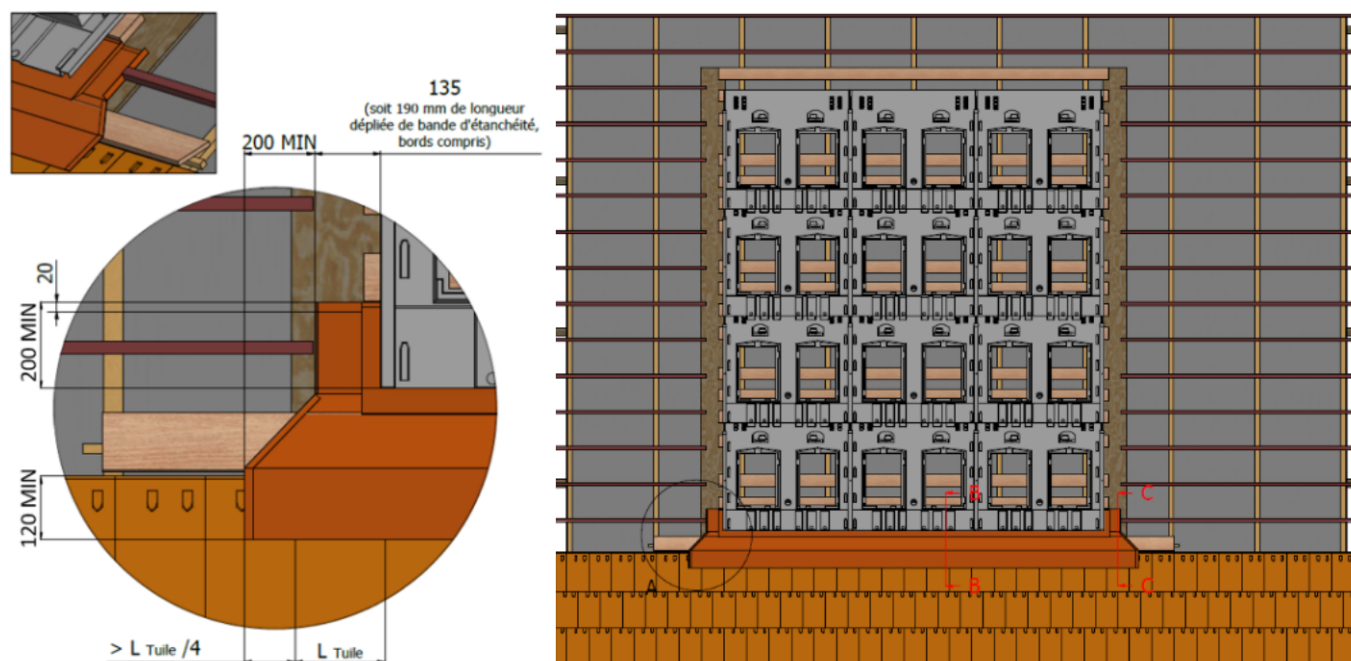
Pose de la bande en milieu de champ
