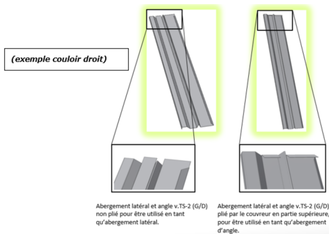
Figure 28 – Pose des abergements latéraux (kit TS-2)
