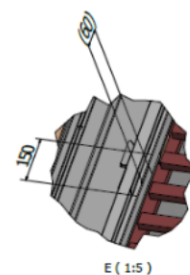
Figure 35 (suite) – Pose des abergements latéraux et d'angles supérieurs (kit A-2)
