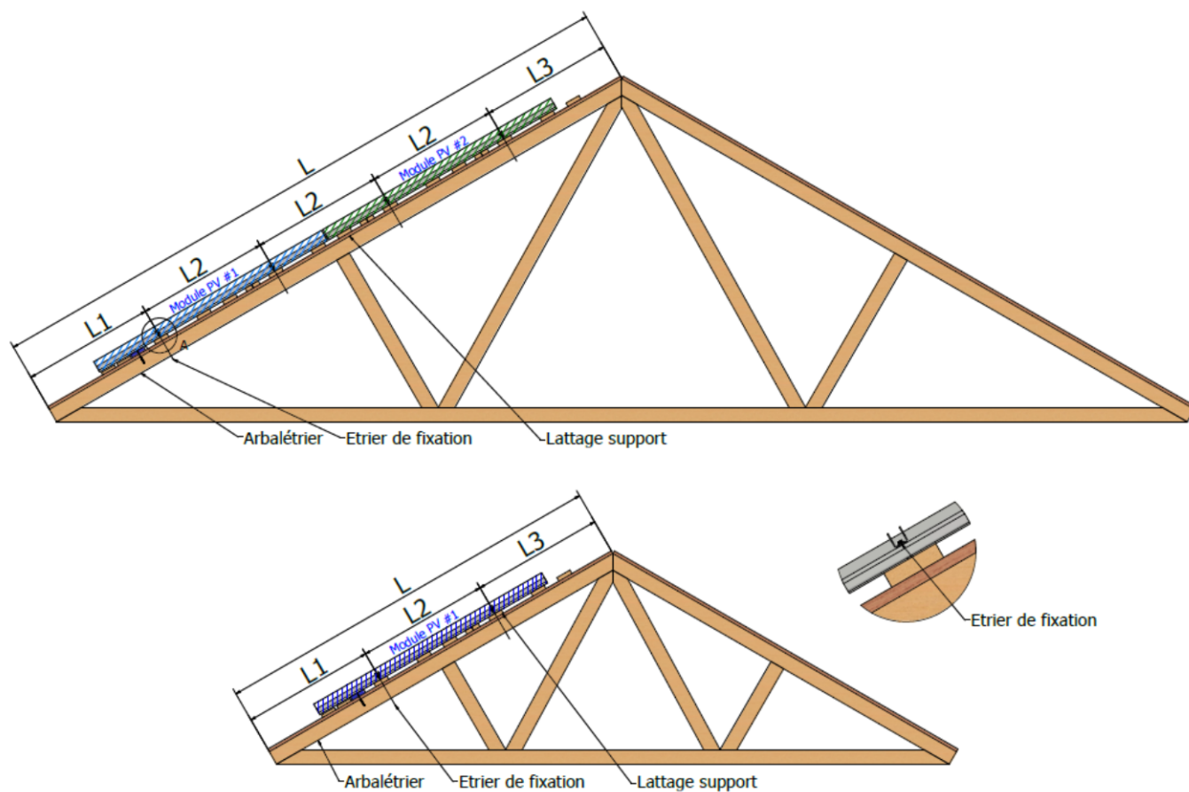
Figure 1 – Dimensionnement des fermettes en considérant des chargements linéiques : longueur L , distances L1 , L2 et L3
