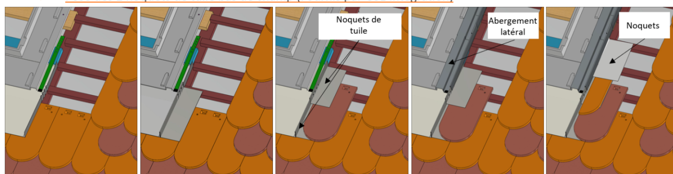
Figure 46 – Pose des abergements latéraux et d'angles supérieurs (kit TP-1)
