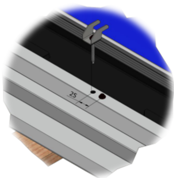
C: Effectuer un nouveau pré-perçement de 10mm décalé de 25 mm au-dessus de l'ancienne position
