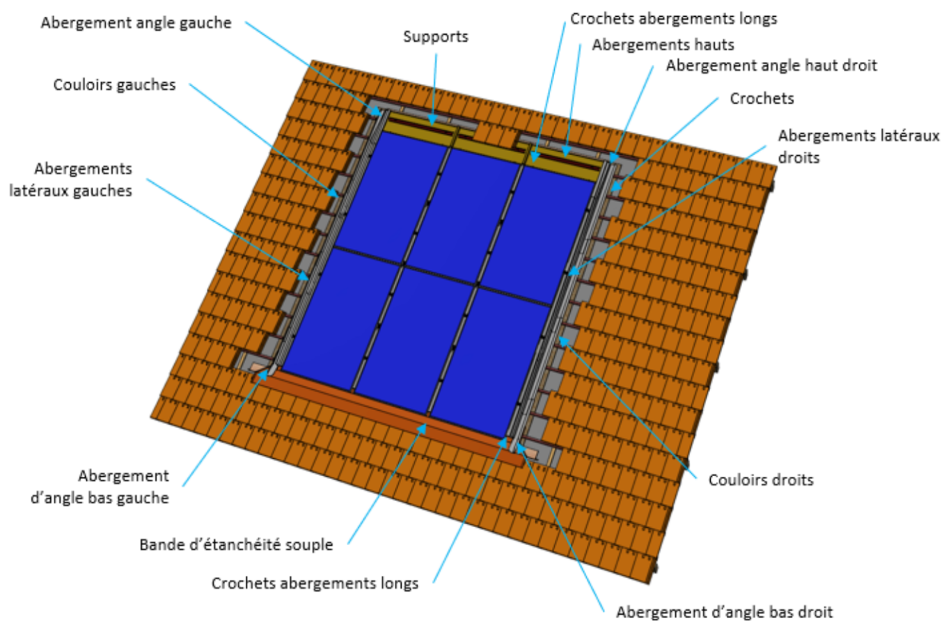
Figure 43 – Éléments du kit TN-1 mis en œuvre
