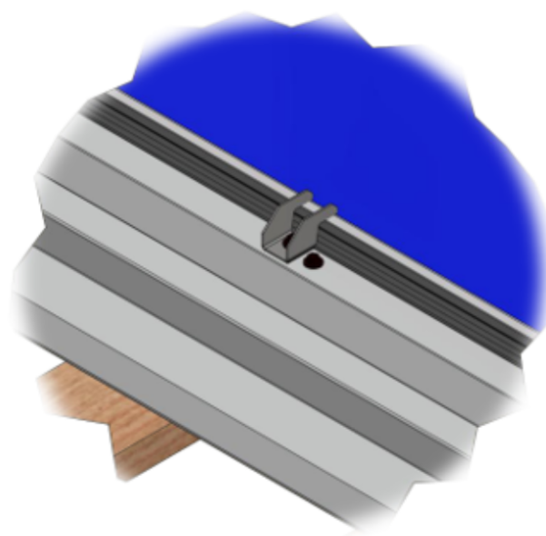
D : Placer le module et fixer les nouveaux ensembles (étrier + joint EPDM + vis CAPINOX).
