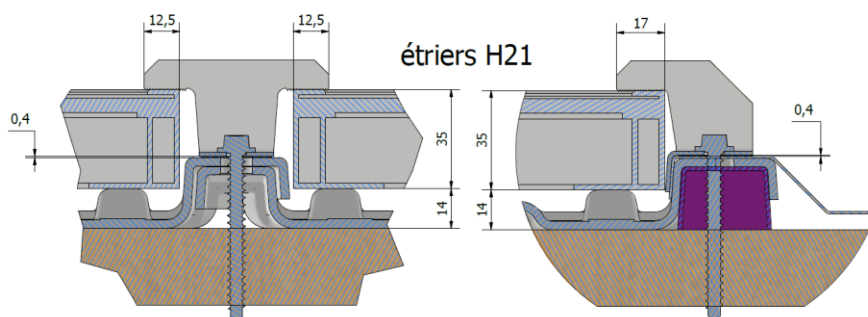
Figure 24 bis –Chaines de cotes de l'écrasement du joint EPDM sous les étriers (suite)
