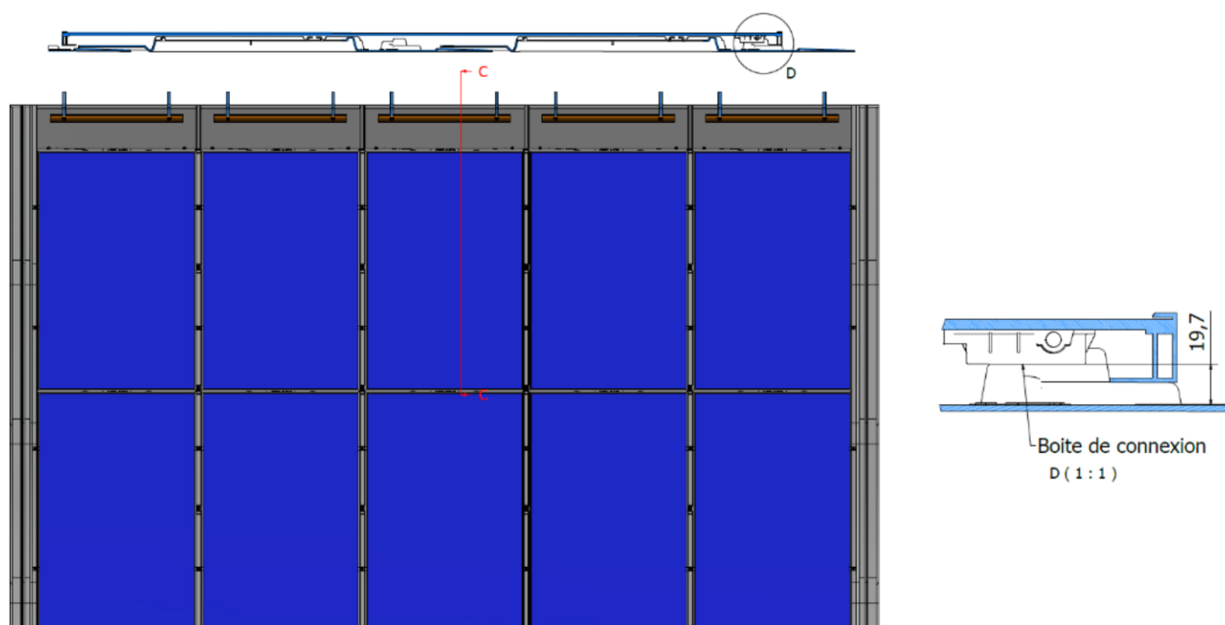
Coupes de l'espace intermodule dans le sens de la pente :
