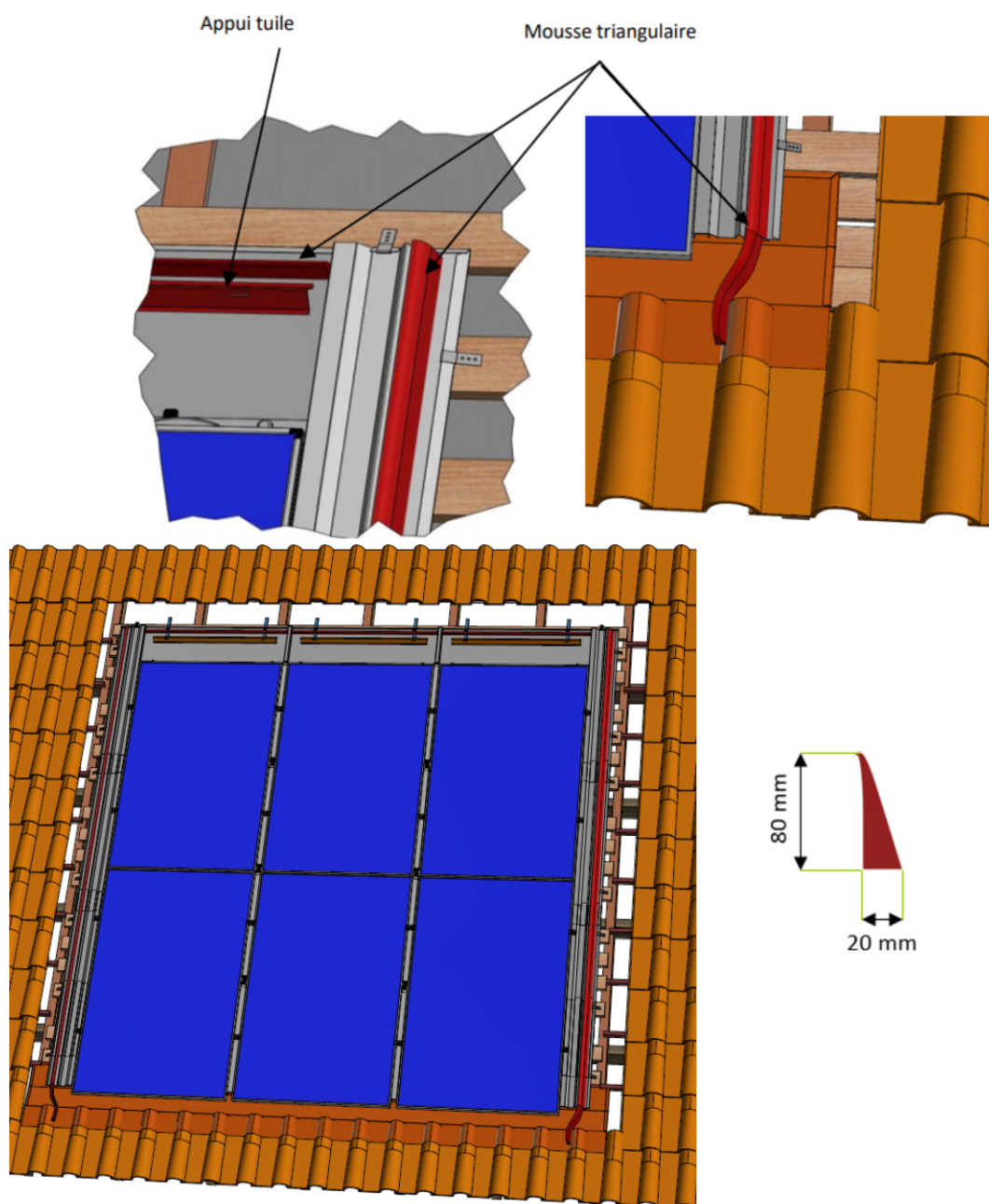
Figure 30 – Pose de la mousse triangulaire (kit TS-2)
