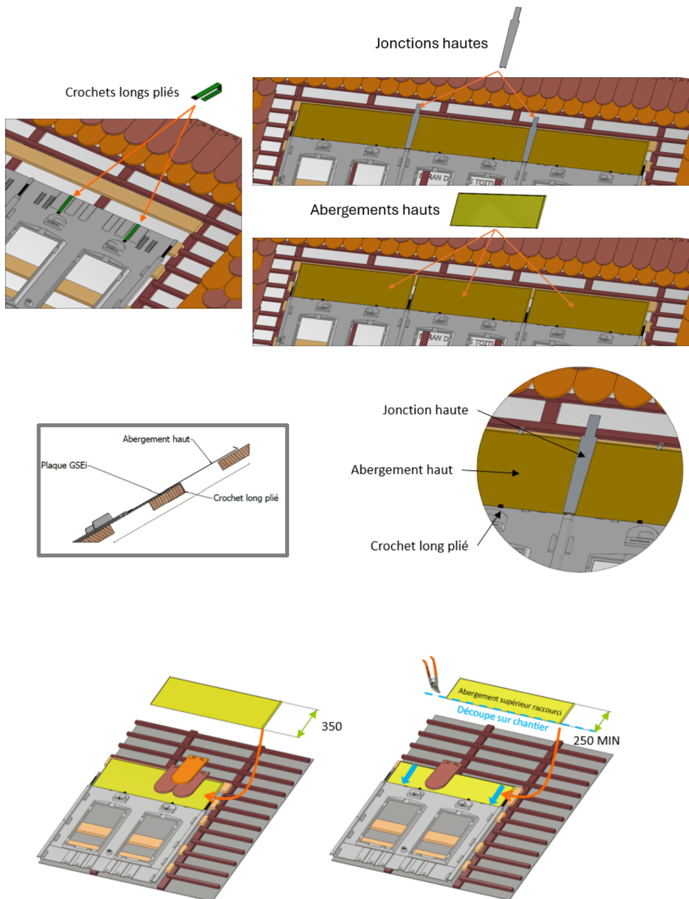
Figure 45 – Pose des abergements supérieurs (kit TP-1)
