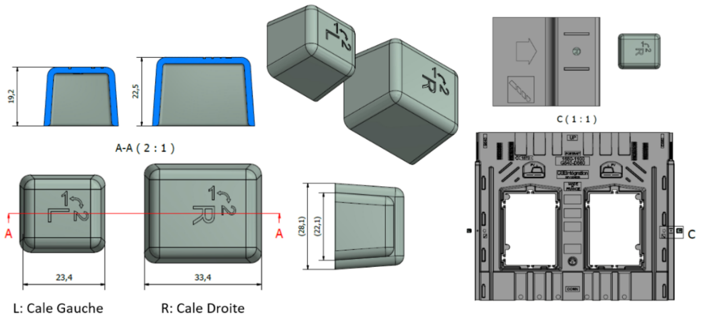
Figure 5 – Cales de bord de champ
