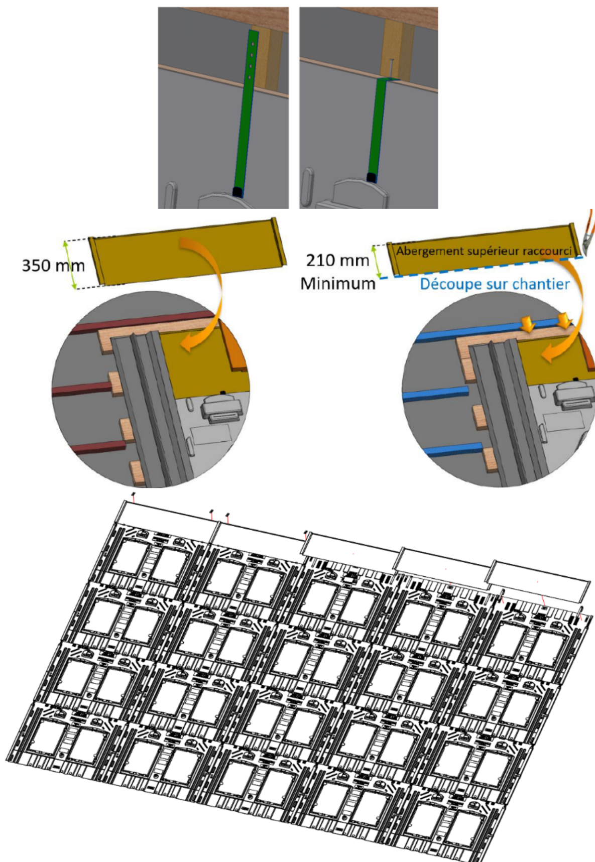
Figure 27 – Pose des abergements supérieurs (kit TS-2)
