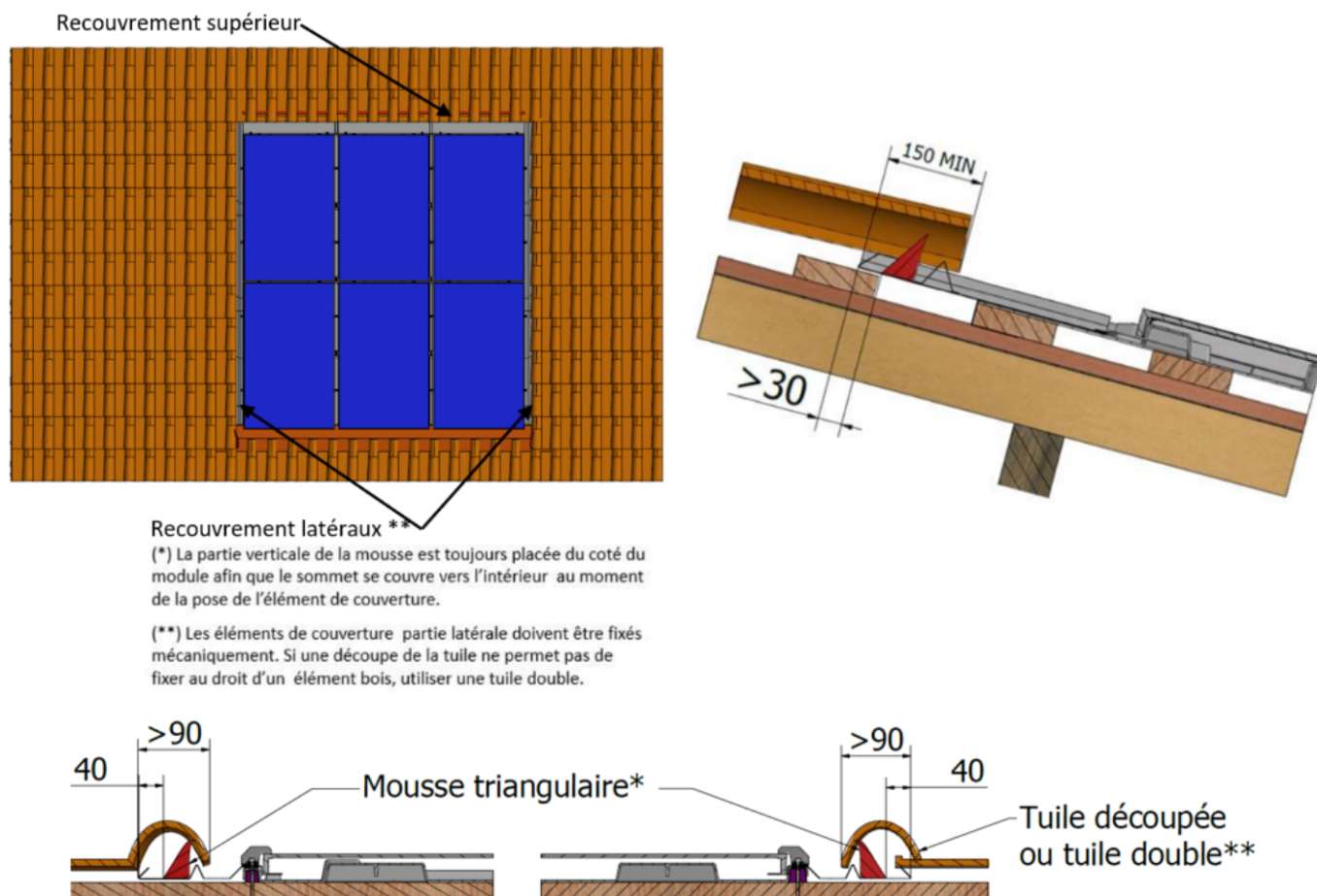
Figure 31 – Mise en place des éléments de couverture (kit TS-2)
