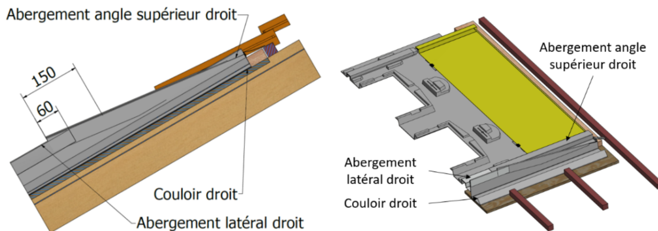
Figure 41 – Pose des abergements latéraux et d'angles supérieurs (kit TN-1) 2/2
