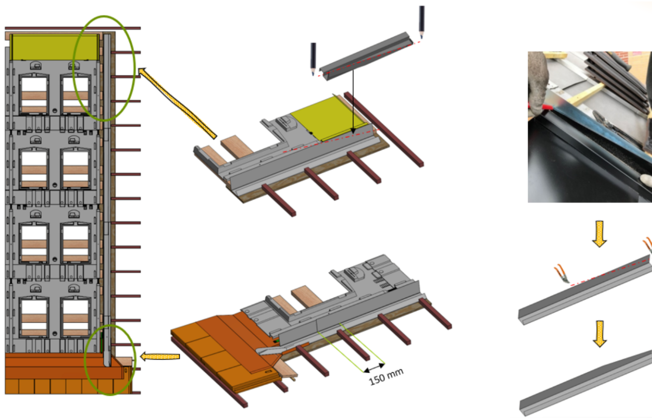
Figure 41 – Pose des abergements latéraux et d'angles supérieurs (kit TN-1) 1/2
