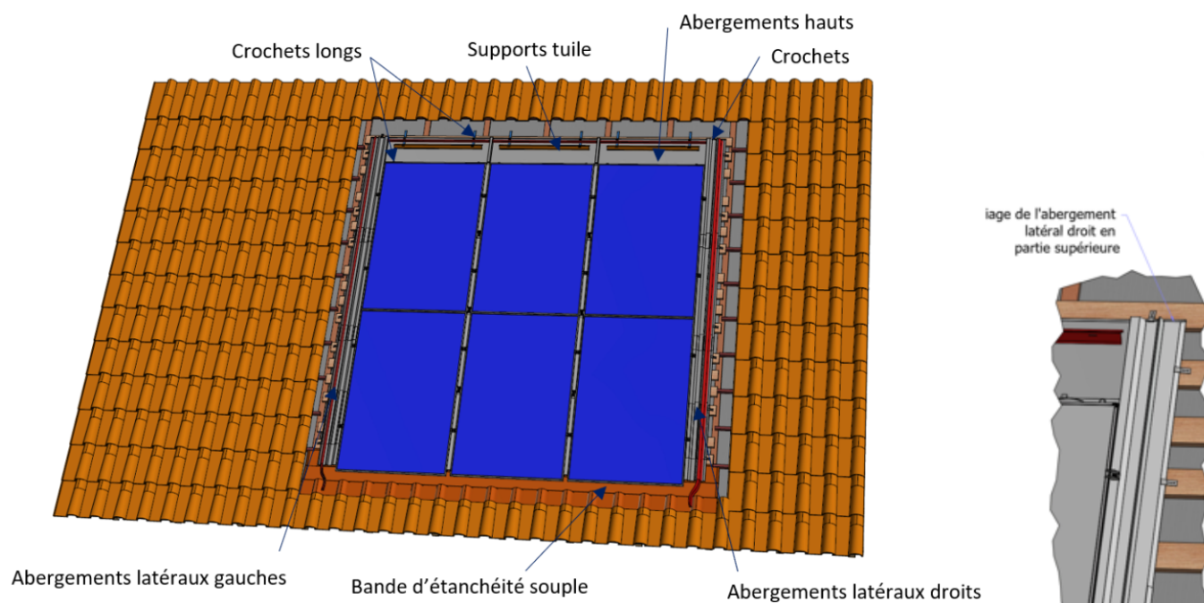
Figure 32 – Éléments du kit TS-2 mis en œuvre
