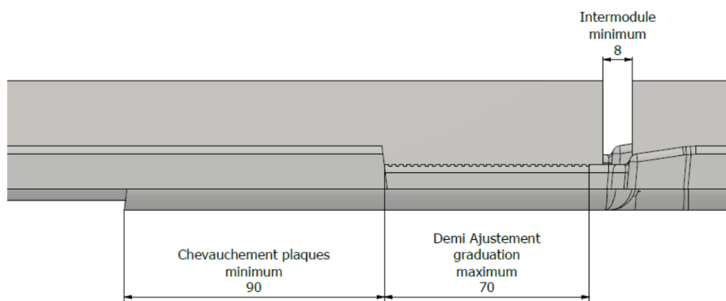
Figure 25 – Positionnement des modules verticalement et en haut de champ
