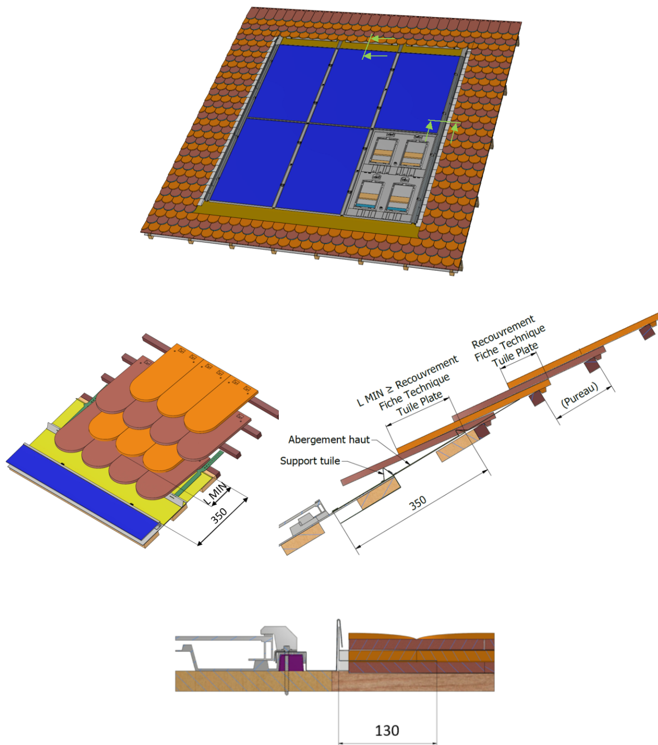
Figure 50 – Mise en œuvre des éléments de couverture (kit TP-1)
