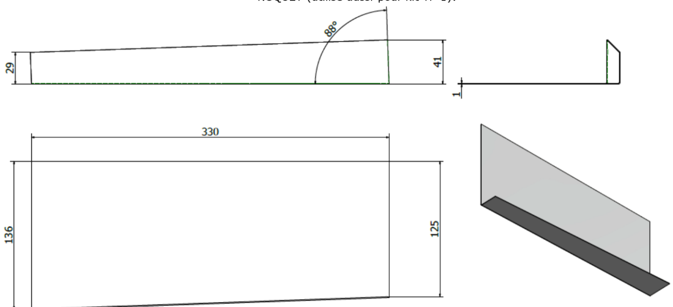
Figure 9 – Abergements latéraux pour kit A-2 (et kit TN-1 et kit TP-1)
