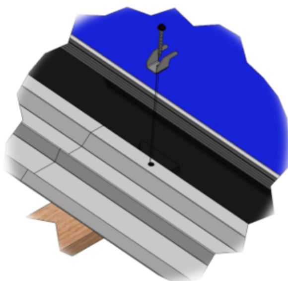
A : Dévisser l'ancien étrier, retirer le module et retirer la cale sous-jacente
