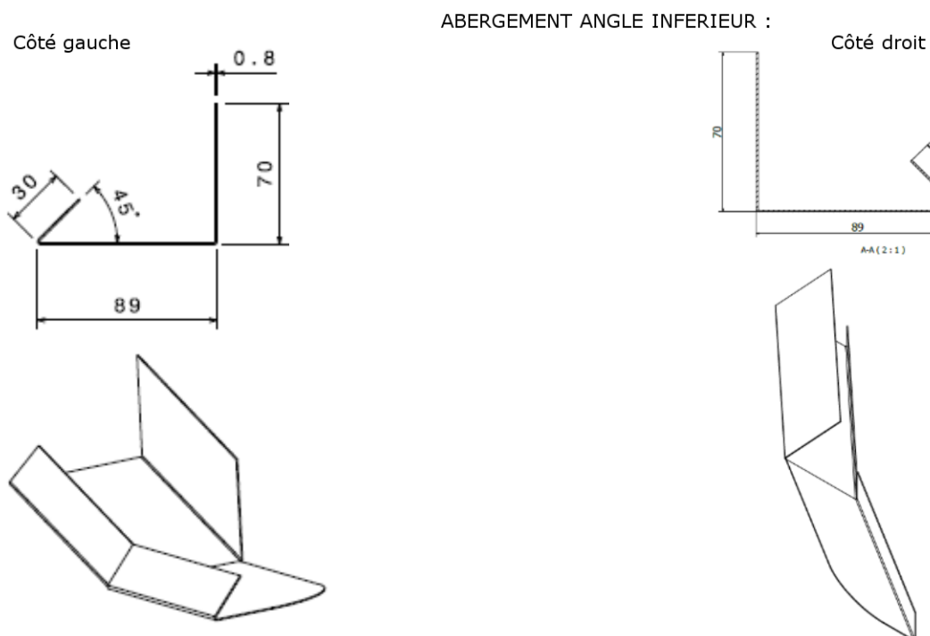
Figure 11 – Ensemble d'abergement latéral pour kit TN-1
