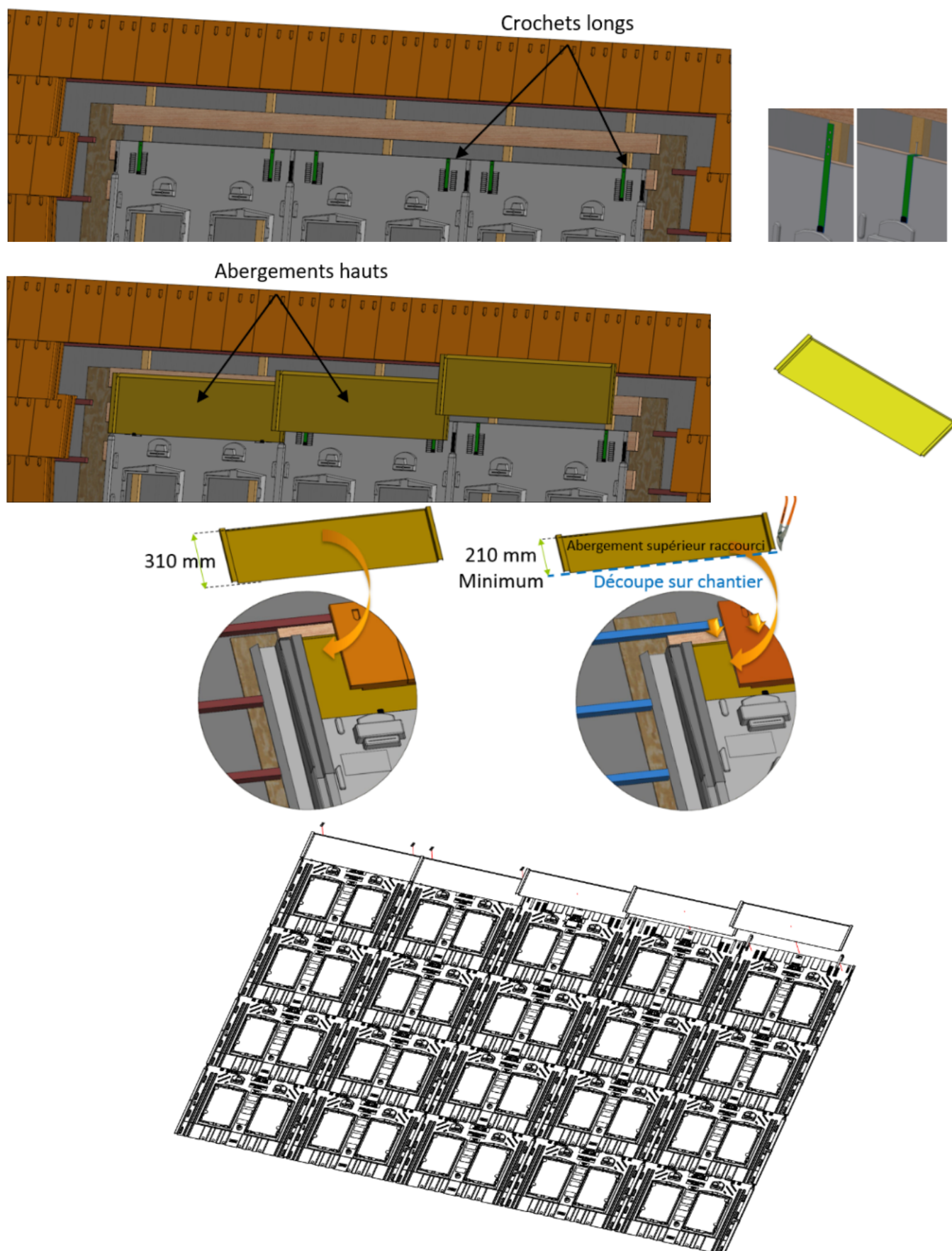
Figure 40 – Pose des abergements supérieurs (kit TN-1)
