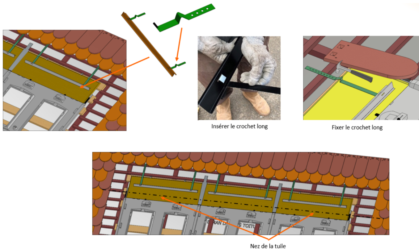
Figure 49 – Pose des appuis de tuiles (kit TP-1)
