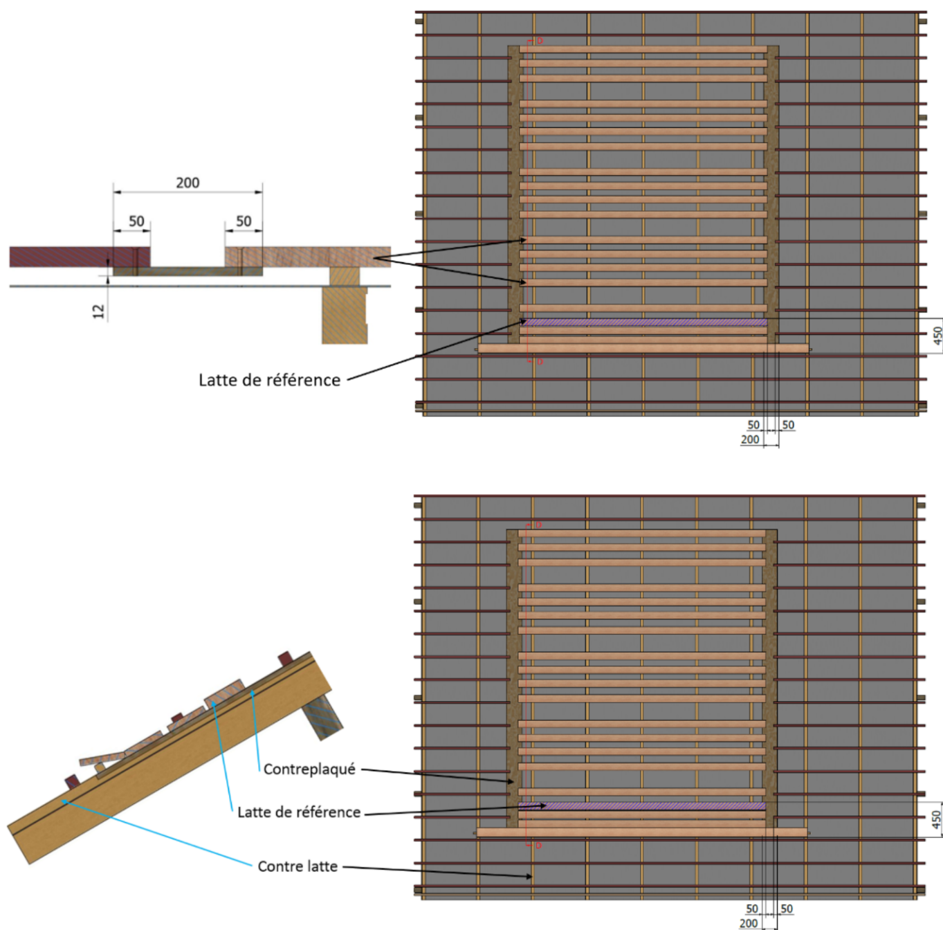
Figure 38 – Pose de la fonçure (kit TN-1)
