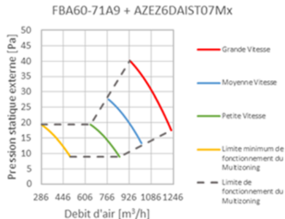
Figure 8 – Unités intérieures FBA60A9 et FBA71A9 Courbes débit/pression
