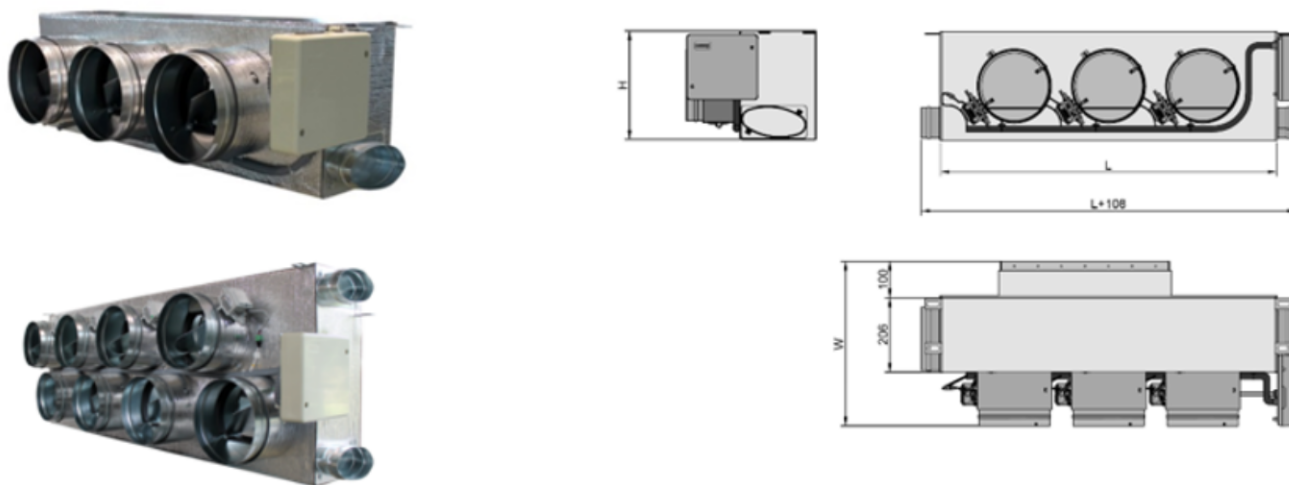
Figure 1 – Plénum motorisé Multizoning Airzone Standard Visuels et caractéristiques dimensionnelles
